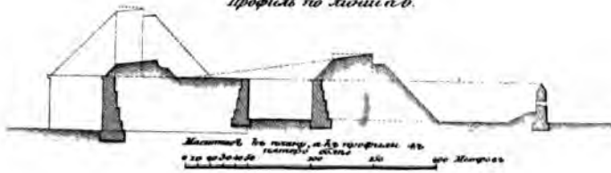
Профиль по линии а-в.
