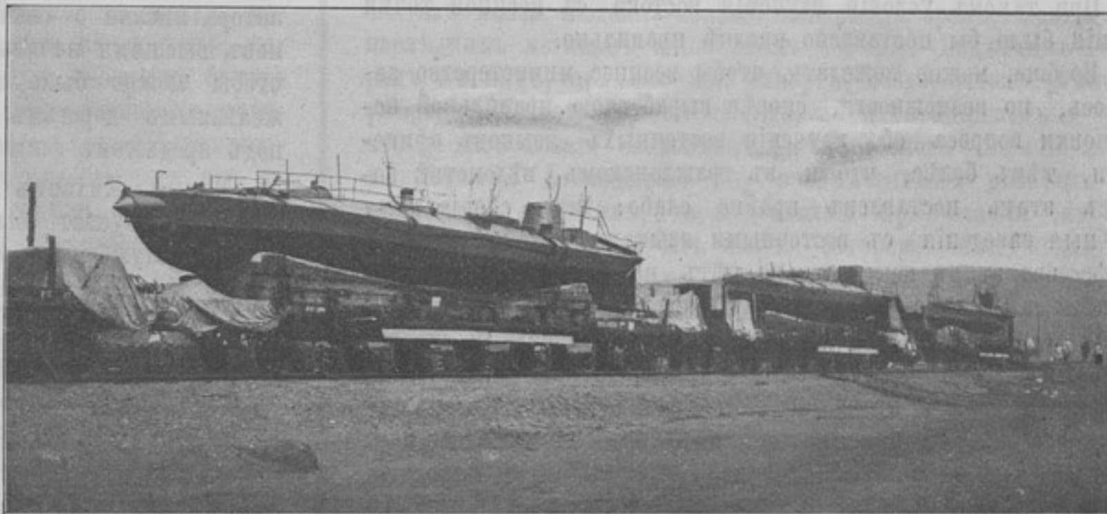
Миноноски, спущенныя въ 1904 году въ 12 вер. отъ Стрѣтенска. (Фотогр. собств. корресп.)
