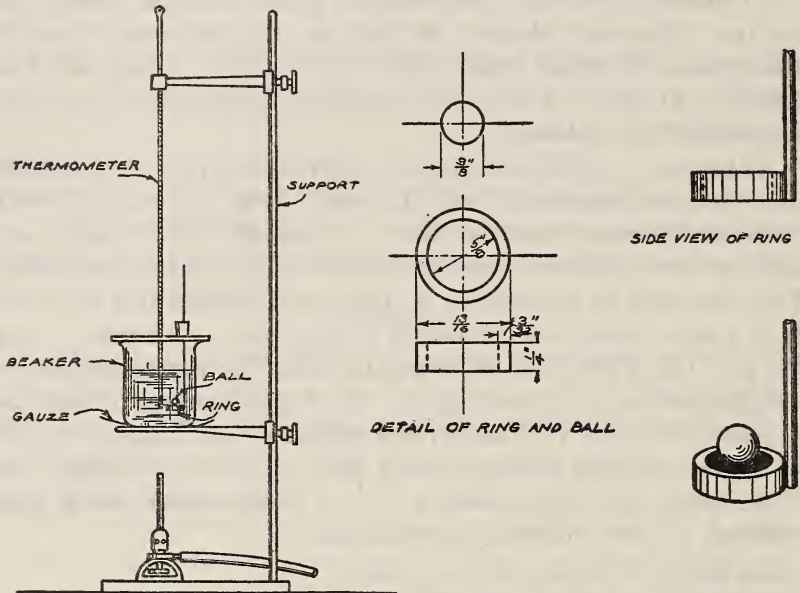
FIG. 1.—Melting point apparatus.
