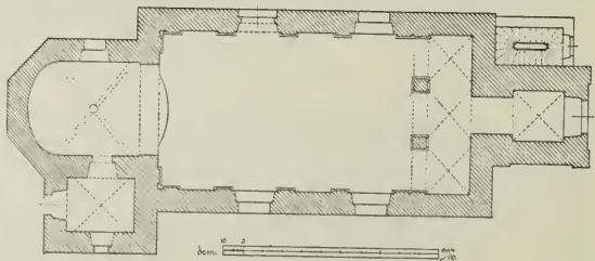
Fig. 7. Borotitz. Grundriss der Kirche.
