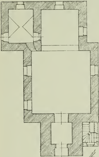
Fig. 85. Lang-Lhota. Grundriss der Kirche.
