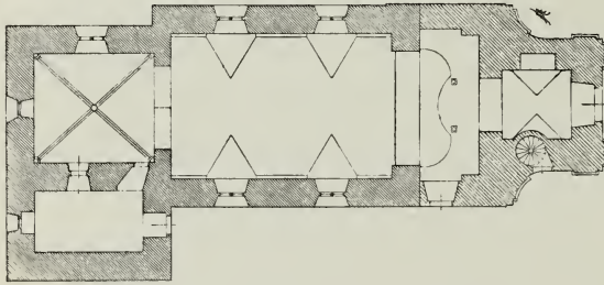
Fig. 118. Pitschin. Grundriss. der Kirche.
