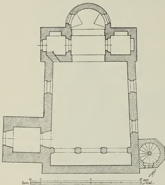
Fig. 212. Suchdol. Grundriss der Kirche.
