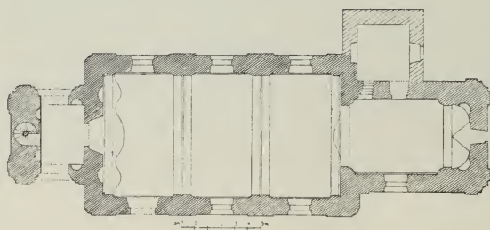
Fig. 72. Alt-Knin. Grundriss der Kirche.
