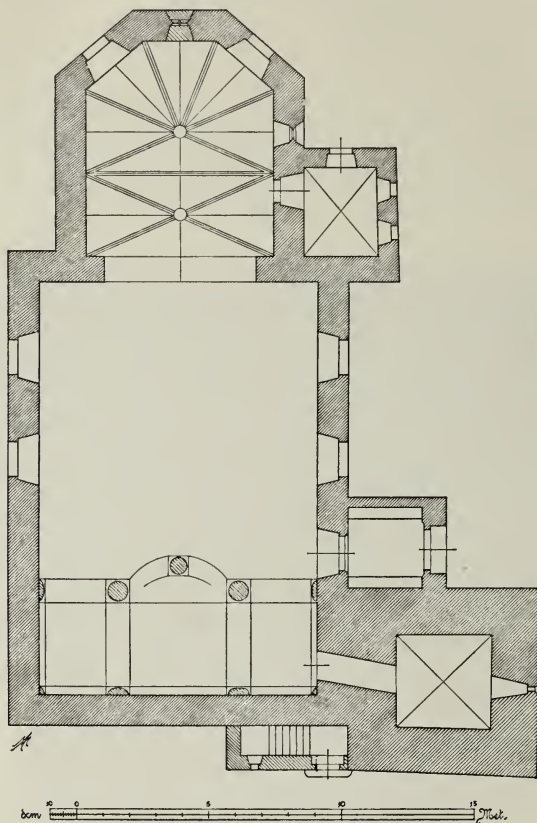
Fig. 192. Sliwitz. Grundriss der Kirche.
