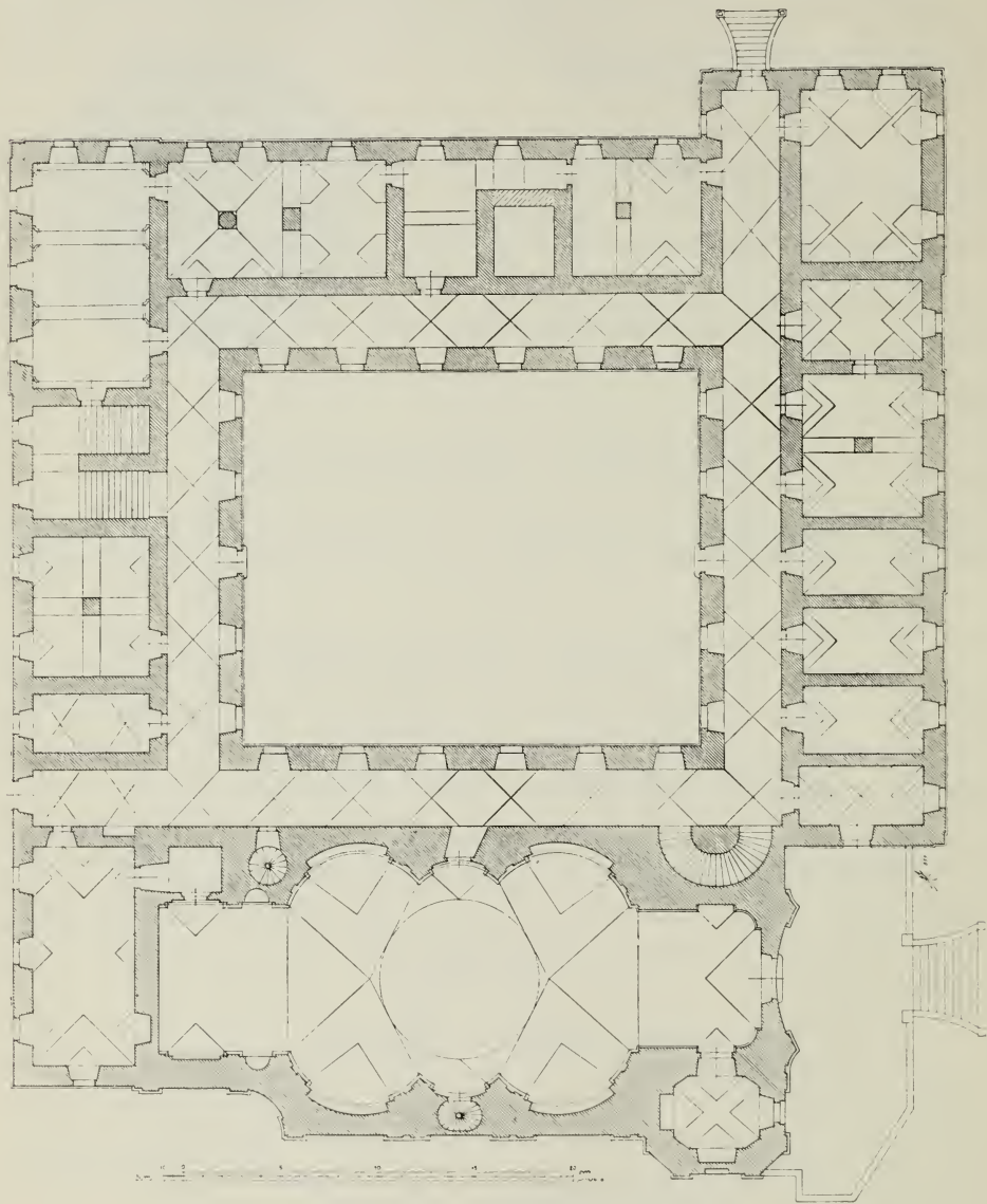
Fig. 103. Wobörscht, Grundriss der Kirche und des Klosters.
