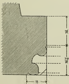
Fig. 194. Sliwitz. Profil des Portals.
