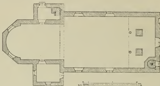
Fig. 215. Werměřitz. Grundriss der Kirche.
