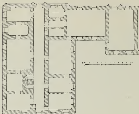
Fig. 209. Sudowitz. Grundriss des Schlosses.
