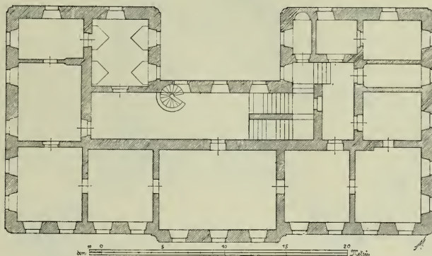
Fig. 12. Buková. Grundriss des Schlosses.
