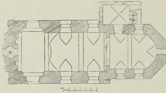
Fig. 67. Neu-Knin. Grundriss der Kirche.
