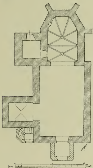
Fig. 219. Wischnowa. Grundriss der Kirche.
