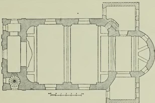
Fig. 17. Dobříš. Grundriss der Pfarrkirche.
