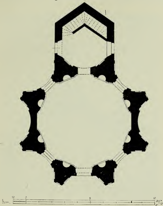
Fig. 15. Čelýň. Grundriss der Kapelle.
