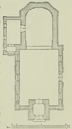
Fig. 1. Birkenberg. Grundriss der Kapelle.
