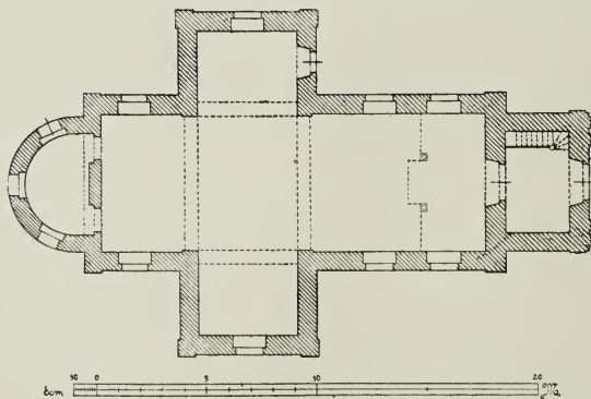
Fig. 102. Obecnitz. Grundriss der Kirche.
