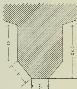
Fig. 119. Pitschin. Console und Rippen-Profil.
