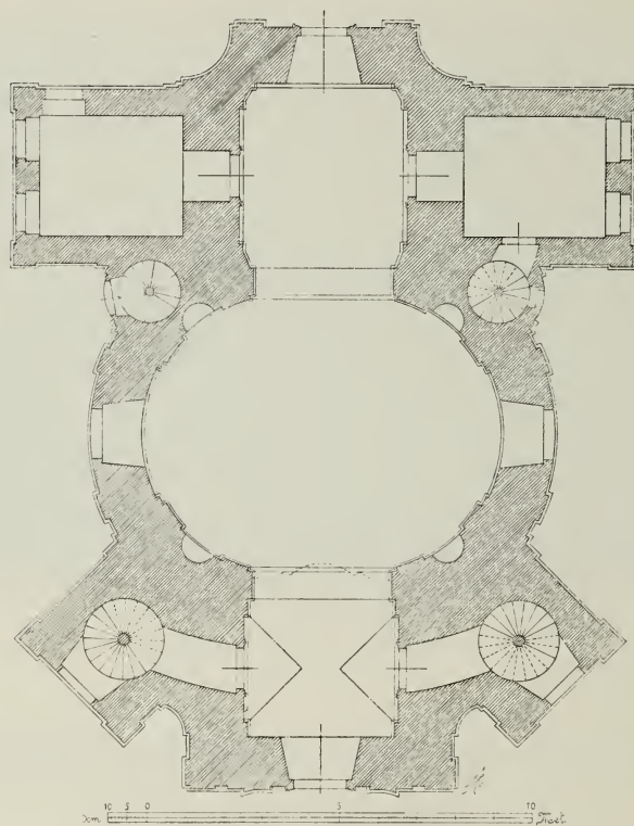
Fig. 91. Makowa. Grundriss der Kirche.
