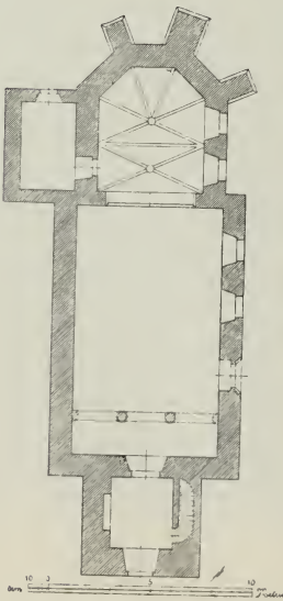
Fig. 111. Gross-Petschitz. Grundriss der Kirche.
