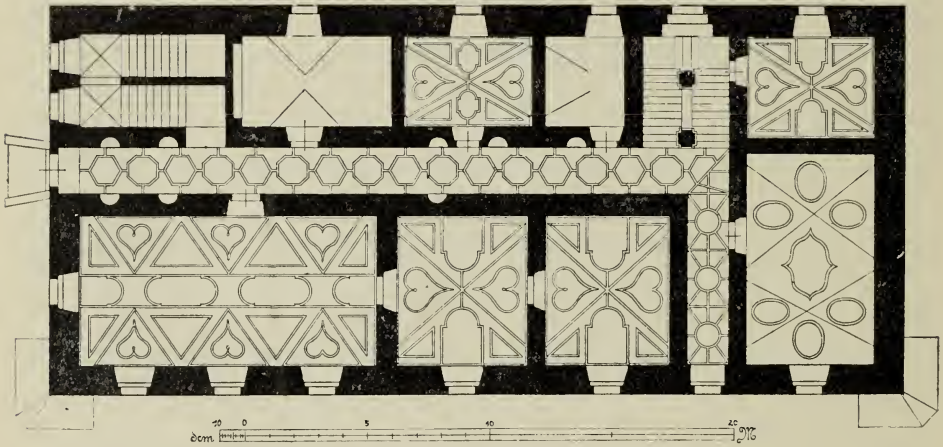
Fig. 223. Zduchowitz. Grundriss des Schlosses.
