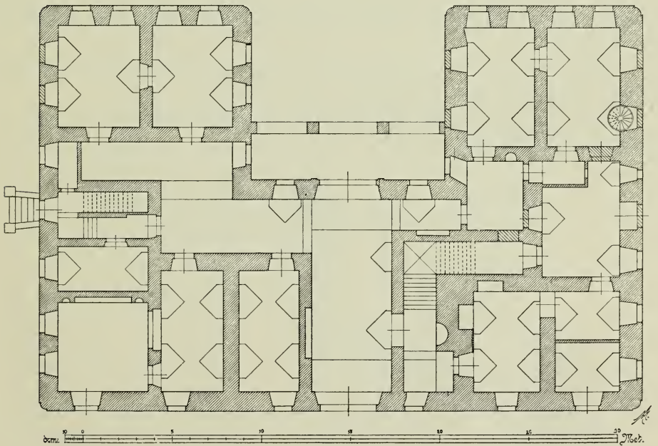
Fig. 199. Smolitel. Grundriss des Schlosses.
