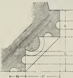
Fig. 115. Gross-Petschitz. Profil des Kirchen-Portales.
