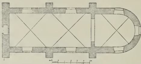
Fig. 38. Dobříš. Grundriss der Friedhofskirche.
