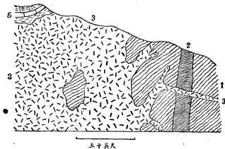
第一圖 泰山系(山東張夏縣)
