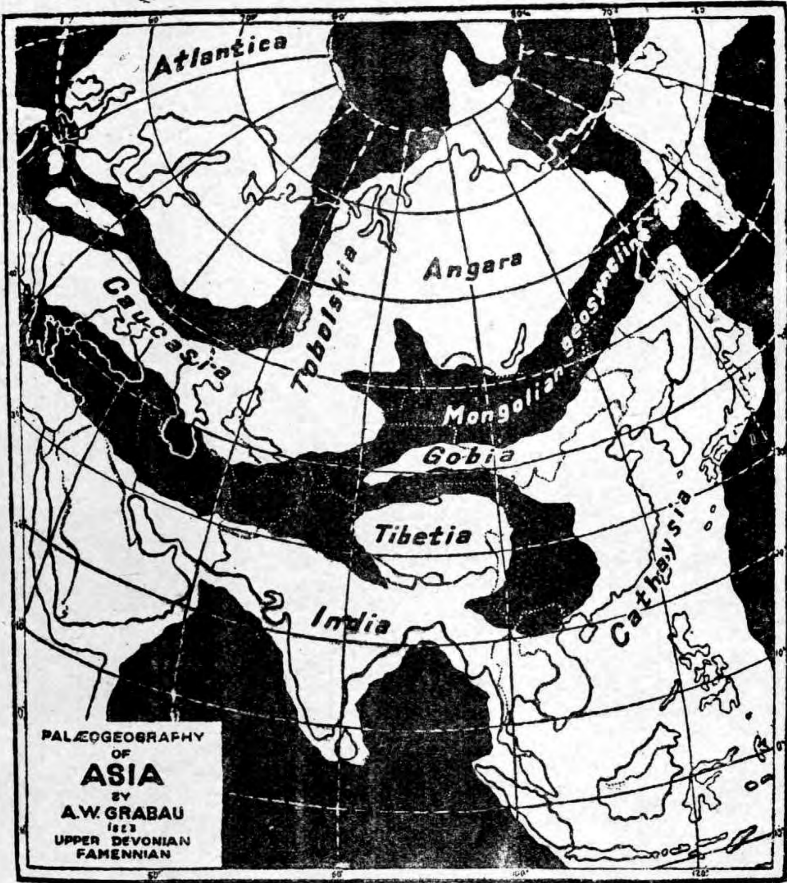
第二十圖 第十七圖之後期
