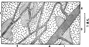
第二圖 泰山系局部的擴大
