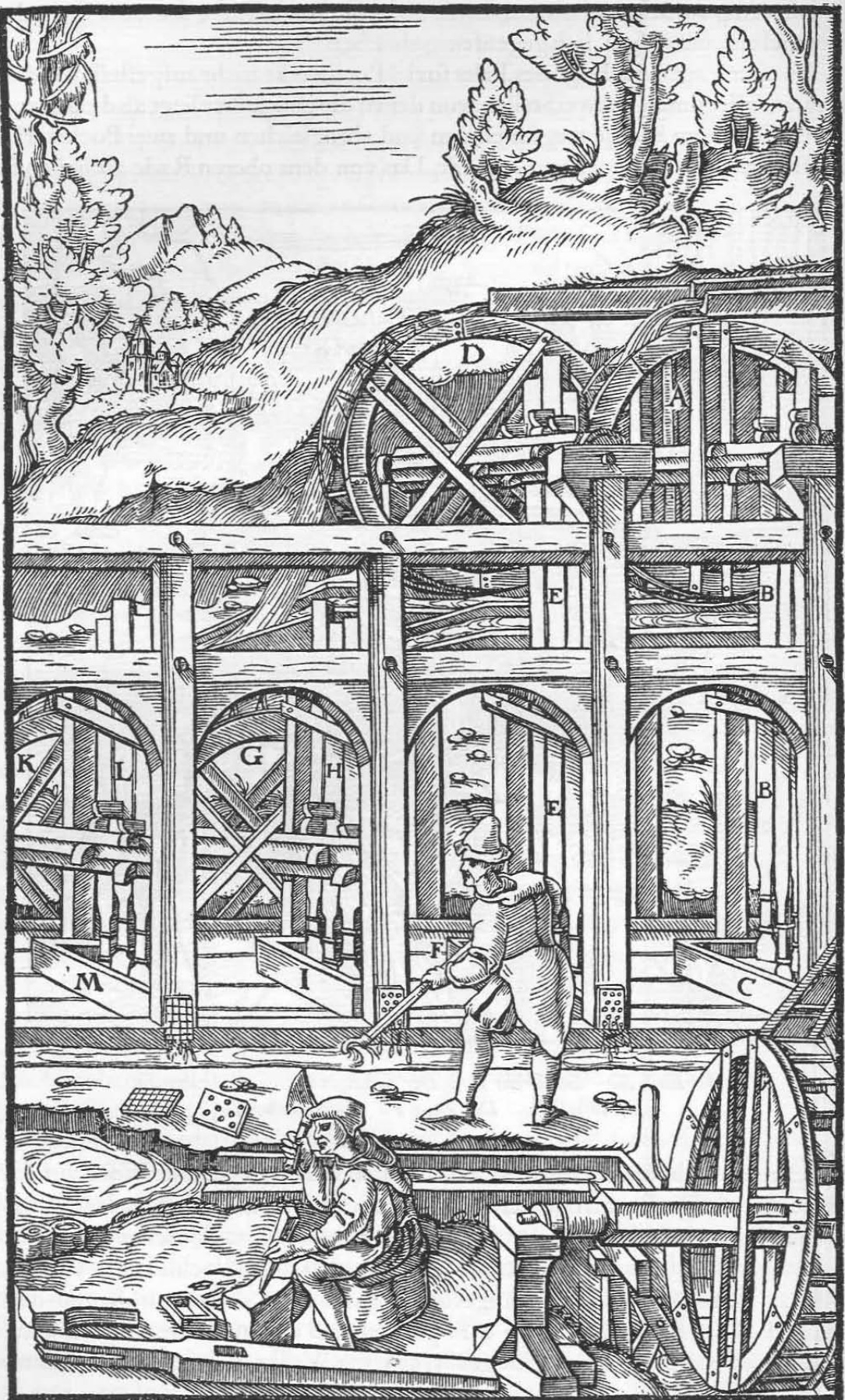
Das erste Gezeug A. Seine Stempel B. Sein Pochtrog C. Das zweite Gezeug D. Seine Stempel E. Sein Pochtrog F. Das dritte Gezeug G. Seine Stempel H. Sein Pochtrog I. Das vierte Gezeug K. Seine Stempel L. Sein Pochtrog M.
