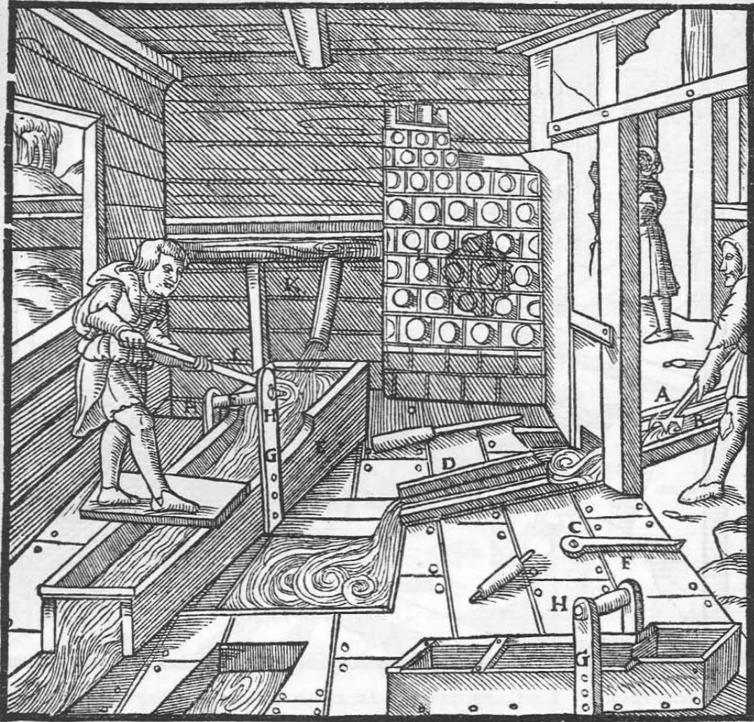
Das erste Gerinne A. Der dreizinkige Krähl B. Der Trog C. Die großen Gräben D. Der Durchlaß E. Die kleine Walze F. Die Bretter G. Ihre Bohrungen H. Die Schaufel I. Das Gebäude K. Der Ofen L.
