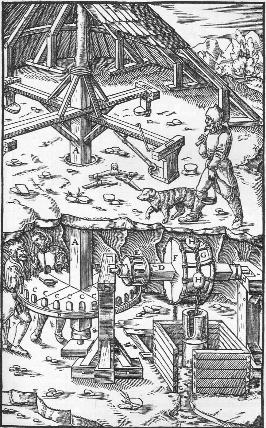
Die stehende Welle A. Das Zahnrad B. Die Kämme C. Die liegende Welle D. Das Getriebe E. Der Kettenkorb F. Die Förderkette G. Die Taschen H.
