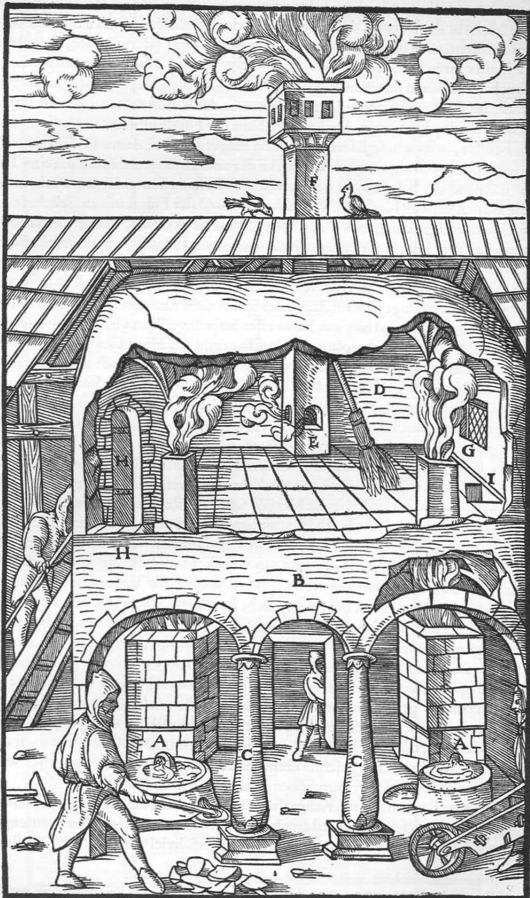
Die Öfen A. Das Gewölbe B. Die Pfeiler C. Die Flugstaubkammer D. Die Öffnung E. Der Rauchfang F. Das Fenster G. Die Tür H. Der Kanal I.
