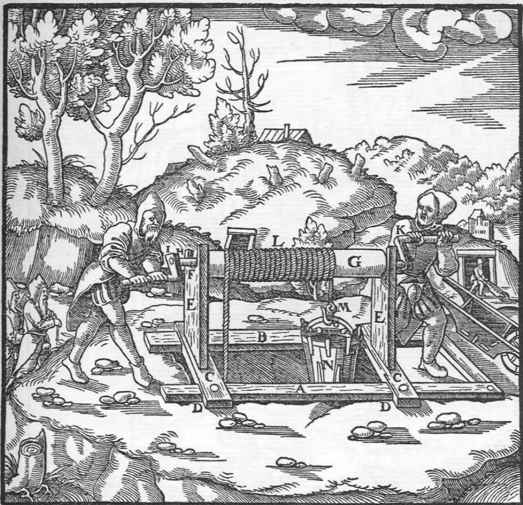
Der vorn am Schacht verlegte Pfühlbaum A. Der hinten am Schacht verlegte Pfühlbaum B. Die zugespitzten Pfähle C. Die Querhölzer D. Die Haspelstützen E. Die Pfadeisen F. Der Rundbaum G. Seine Zapfen H. Das Holz I. Die Kurbel K. Das Förderseil L. Der Seilhaken M. Das Fördergefäß N. Sein Bügel O.
