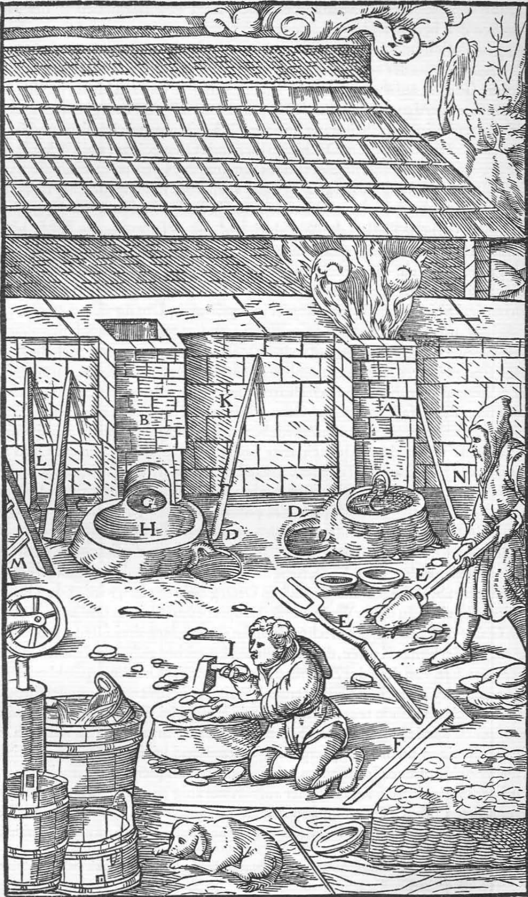
Zwei Öfen A und B. Der obere Vorherd C. Der untere Vorherd D. An dem einen Ofen steht der Arbeiter und entfernt mit einer eisernen Gabel die Schlacken. Die Gabel E. Die hölzerne Krücke, mit welcher der aus den Kiesen erschmolzene Stein abgezogen wird F. Beim zweiten Ofen der in das Ofeninnere hineinragende Teil des oberen Vorherdes G. Der außerhalb befindliche Teil H. Der Vorarbeiter, der den Vorherd vorrichtet, aber abseits vom Ofen I. Die Stange K. Der hölzerne Stampfer L. Die Treppe M. Die Kelle N.
