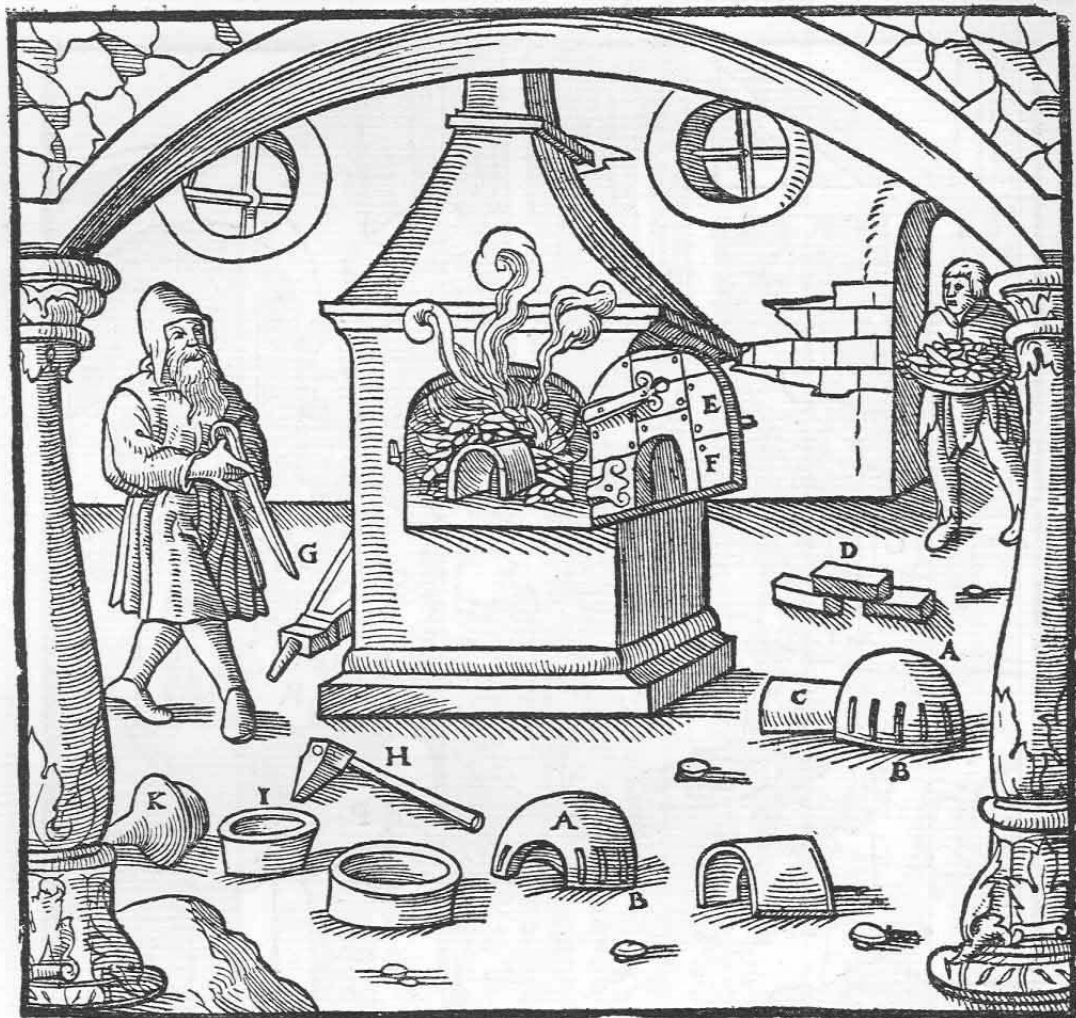
Die Muffel A. Ihre Fensterchen B. Ihr Steglein C. Backsteine D. Die Eisentür E. Ihr Fensterchen F. Der Blasebalg G. Das meißelförmige Gerät H. Der Eisenring, den manche an Stelle eines Teftſcherbens verwenden I. Das Piſtill zum Stampfen der Aſche im Ring K.
