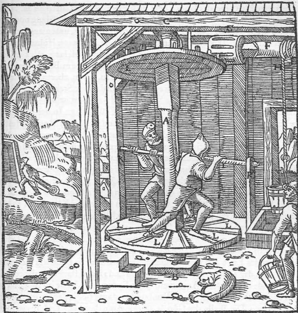
Die stehende Welle A. Der Klotz des Fußlagers B. Das Gebälk C. Die Scheibe D. Das Kammrad E. Die liegende Welle F. Das Getriebe G. Das Förderseil H. Die Stange I. Die Säulen K. Die Leisten der Scheibe L.
