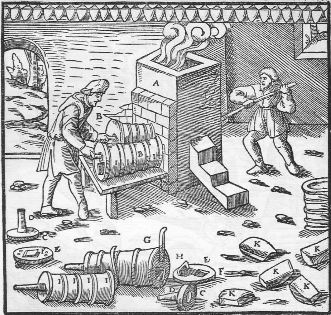
Der Ofen A. Die Blasebälge B. Die eiserne Scheibe C. Die Düse D. Die hölzerne Scheibe E. Das Windventil F. Die Handhabe G. Der Henkel H. Die eisernen Ringe I. Zinnbarren K.
