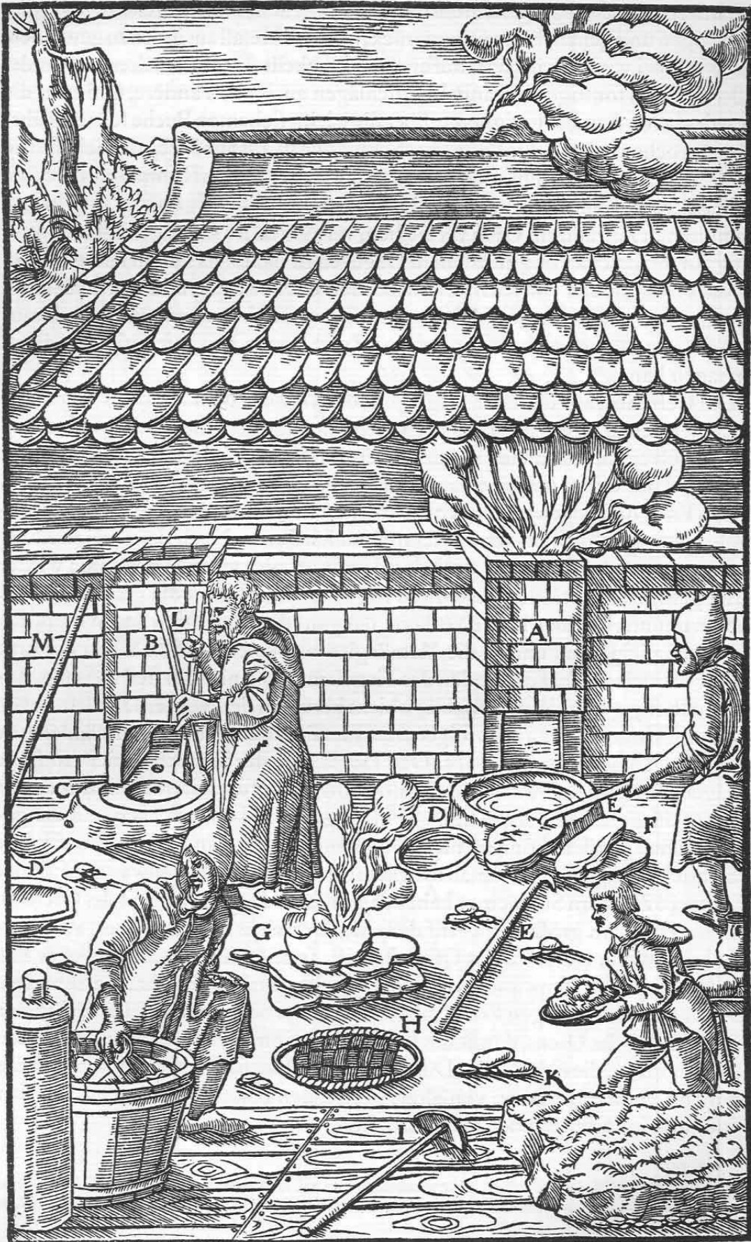
Zwei Öfen A B. Der obere Vorherd C. Der untere Vorherd D. Der am ersten Ofen stehende Schmelzer zieht mit einem Schlackenhaken die Schlacken ab. Der Schlackenhaken E. Schlacken F. Der Arbeiter schöpft Wasser in einen Eimer und gießt es auf die glühenden Schlacken, um sie abzulöschen G. Die aus Holzspänen gestochene Mulde H. Die gewöhnliche Krücke I. Das zu verschmelzende Erz K. Der am andern Ofen stehende Arbeiter stellt durch Stampfen mit zwei Stampfern den Vorherd her. Die Stampfer L. Eine Stange M.
