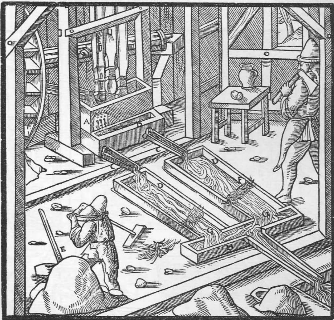
Das gelochte Blech A. Das Quergerinne B. Die kleinen Gerinne C. Die großen Gräben D. Die Schaufel E. Die Reisfigbündel F. Die Bretter, welche die Kanäle abschließen G. Das andere Quergerinne H.
