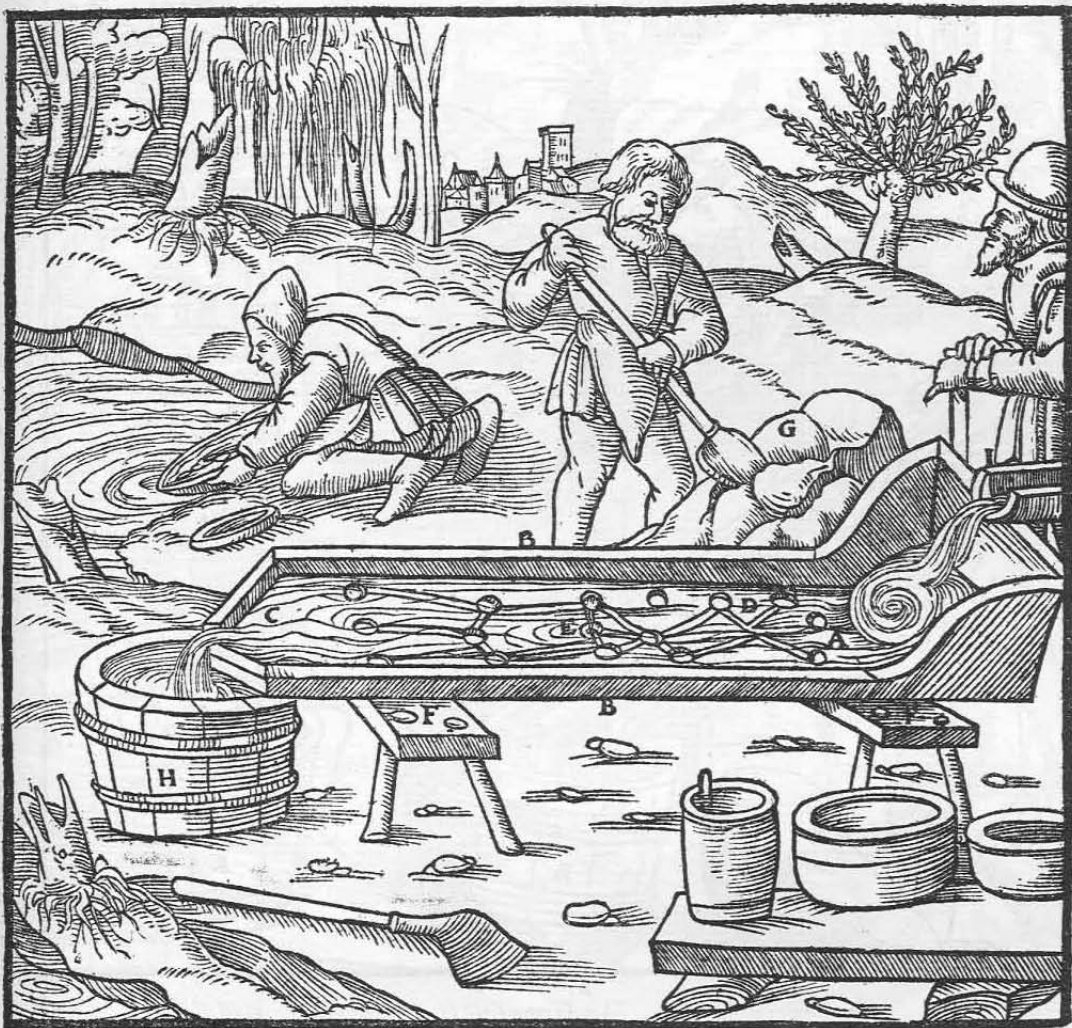
Das Haupt des Herdes A. Die Seitenbretter B. Der unterste Teil des Herdes C. Die Näpfchen D. Die Rillen E. Die Böcke F. Die Schaufel G. Das Unterfaß H. Das Wassergerinne I.
