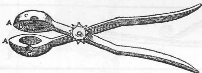
Die Backen der Zange A. Der eiförmige Teil B. Der Einguß C.
