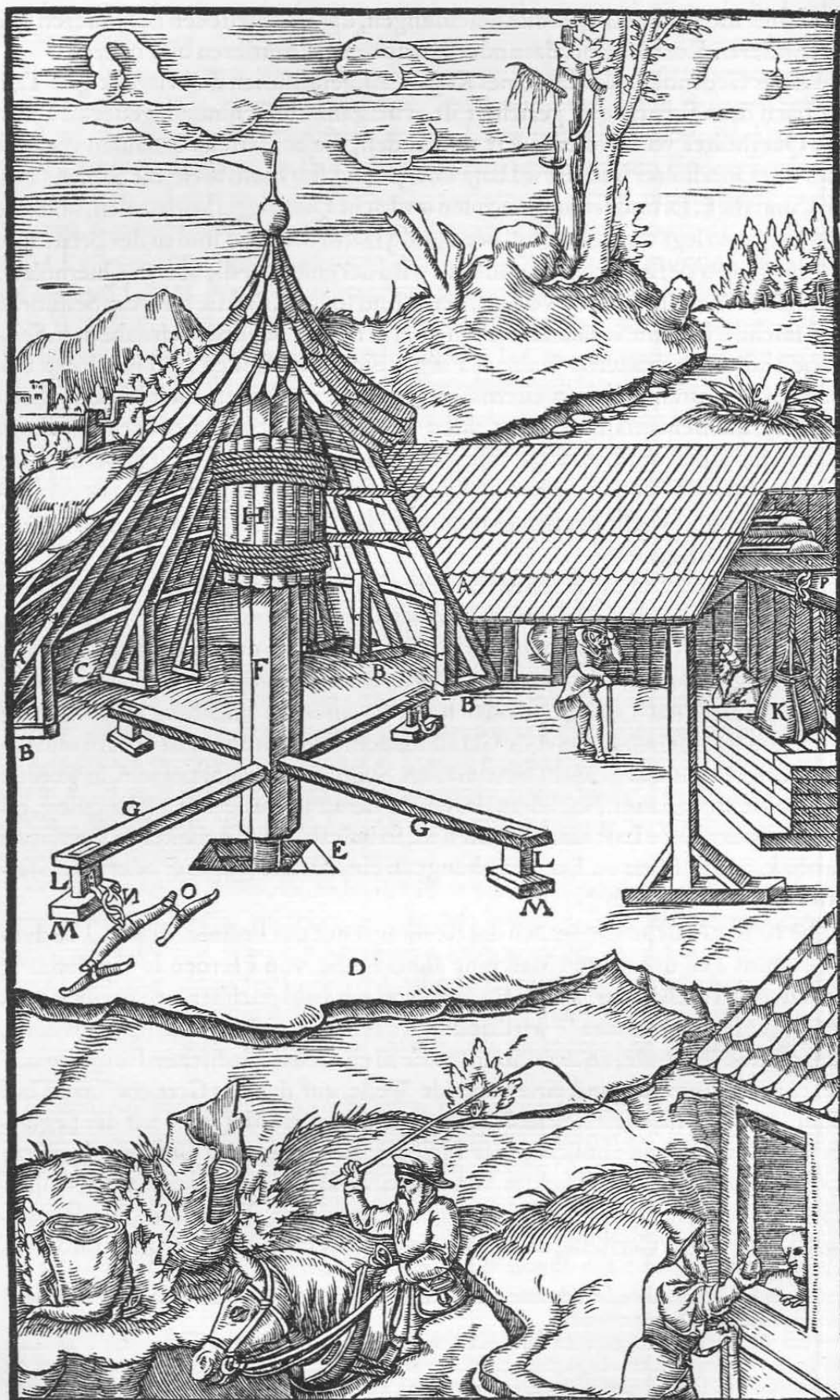
Die Sparren A. Die Schuhe B. Die Steifen C. Der Umlauf im Göpel D. Der Holzklotz für den Fußlager E. Die Welle F. Die Schwengel G. Der Seilkorb H. Die Seile I. Das Fördergefäß K. Die in die Schwengel eingesetzten Hölzer L. Der Schemel für den Treiber, an den auch die Pferde gespannt werden M. Die Kette N. Die Wage O. Der Sturzhaken P.
