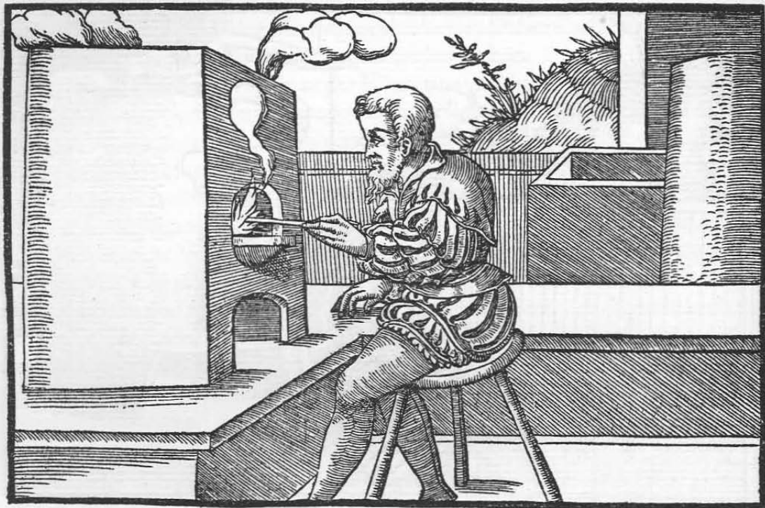
Rechteckiger Probierofen.
