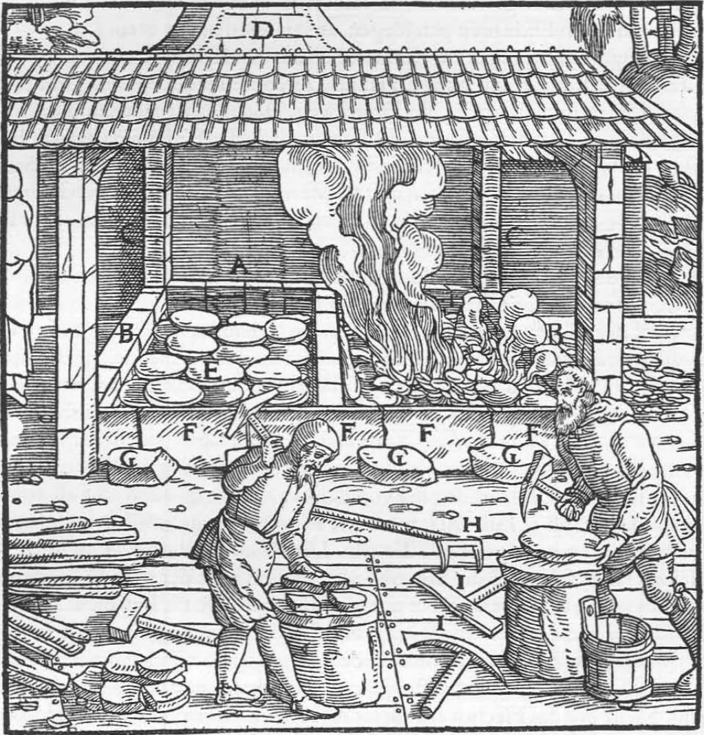
Die Rückwand A. Die Seitenwände B. Die Tragsäulen C. Der Rauchabzug D. Die eingetragenen Stücke E. Die Eisenblechplatten F. Feldsteine G. Die zweizinkige Harke H. Der Hammer I.
