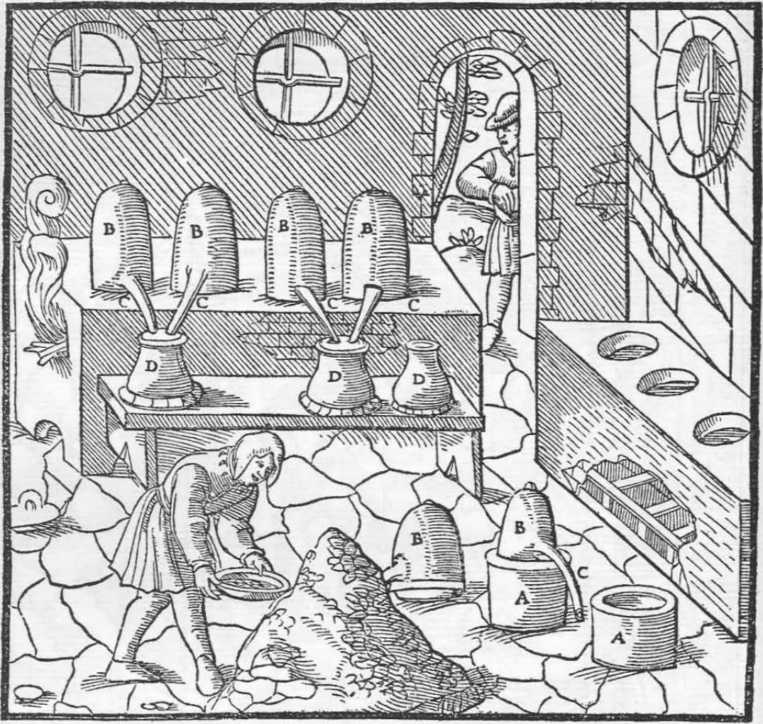
Die Töpfe A. Die Hauben B. Die Nasen C. Die kürbisförmigen Tongefäße D.
