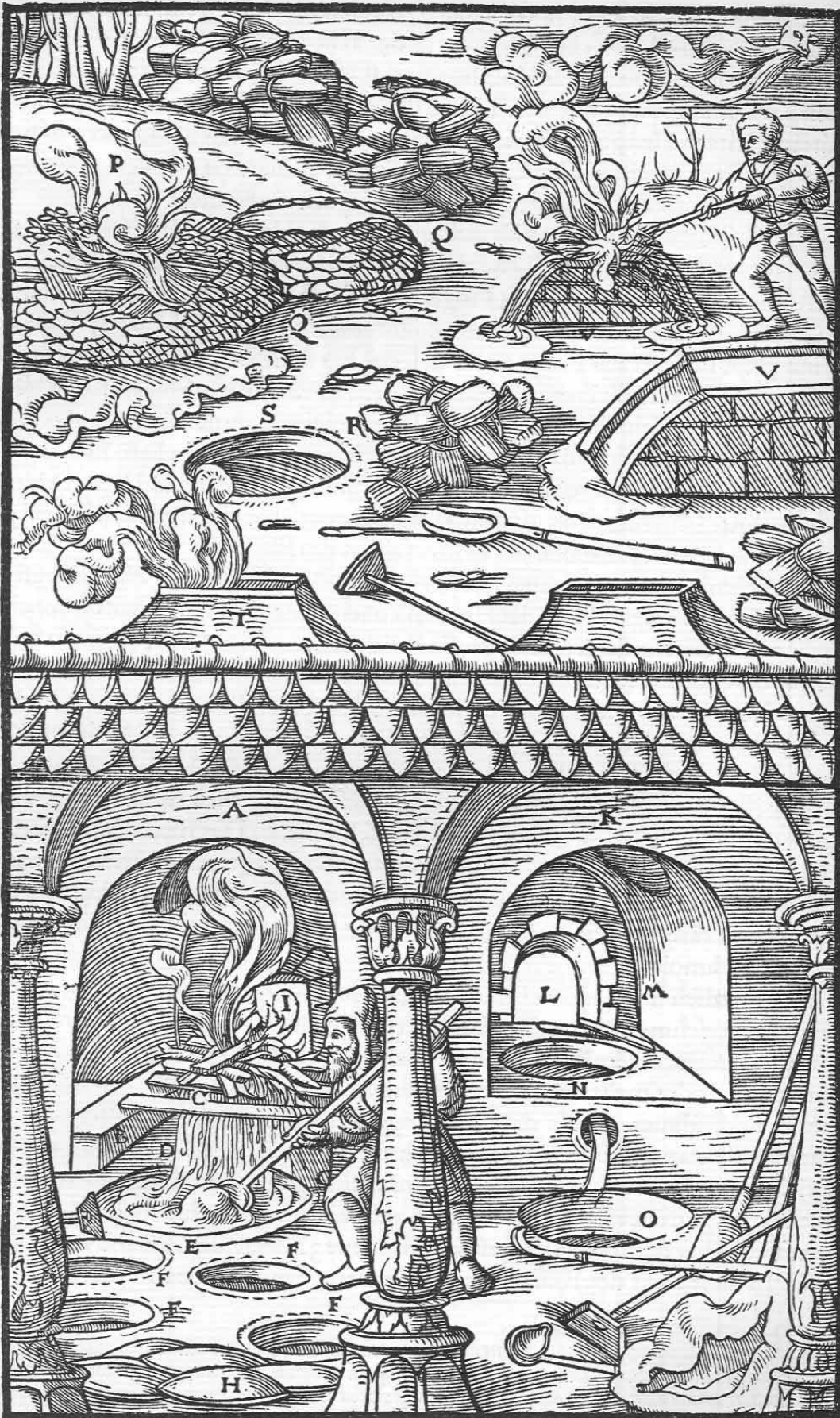
Der Kärntner Ofen A. Die eine niedrige Mauer B. Holz C. Das Erz mit dem heraustropfenden Blei D. Der große Tiegel E. Die kleinen Tiegel F. Die Kelle G. Bleikuchen H. Die rechteckige Öffnung in der Rückwand des Ofens I. Der sächsische Ofen K. Die Öffnung in der Rückwand des Ofens L. Holz M. Der obere Tiegel N. Der untere Tiegel O. Das Schmelzverfahren der Westfalen P. Kohlenhaufen Q. Strohbindel R. Die flachen Bleikuchen S. Der Tiegel T. Der ungarische Herd V.
