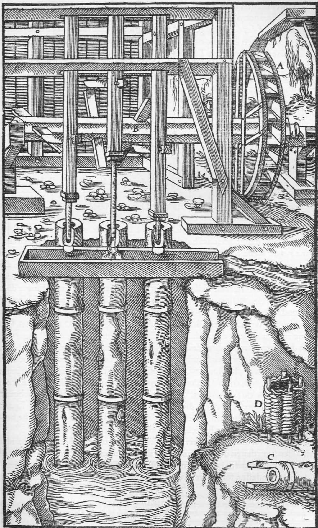
Das Wasserrad A. Die Welle B. Der Stock, auf dem das unterste Rohr steht C. Der den Stock umgebende Korb D.
