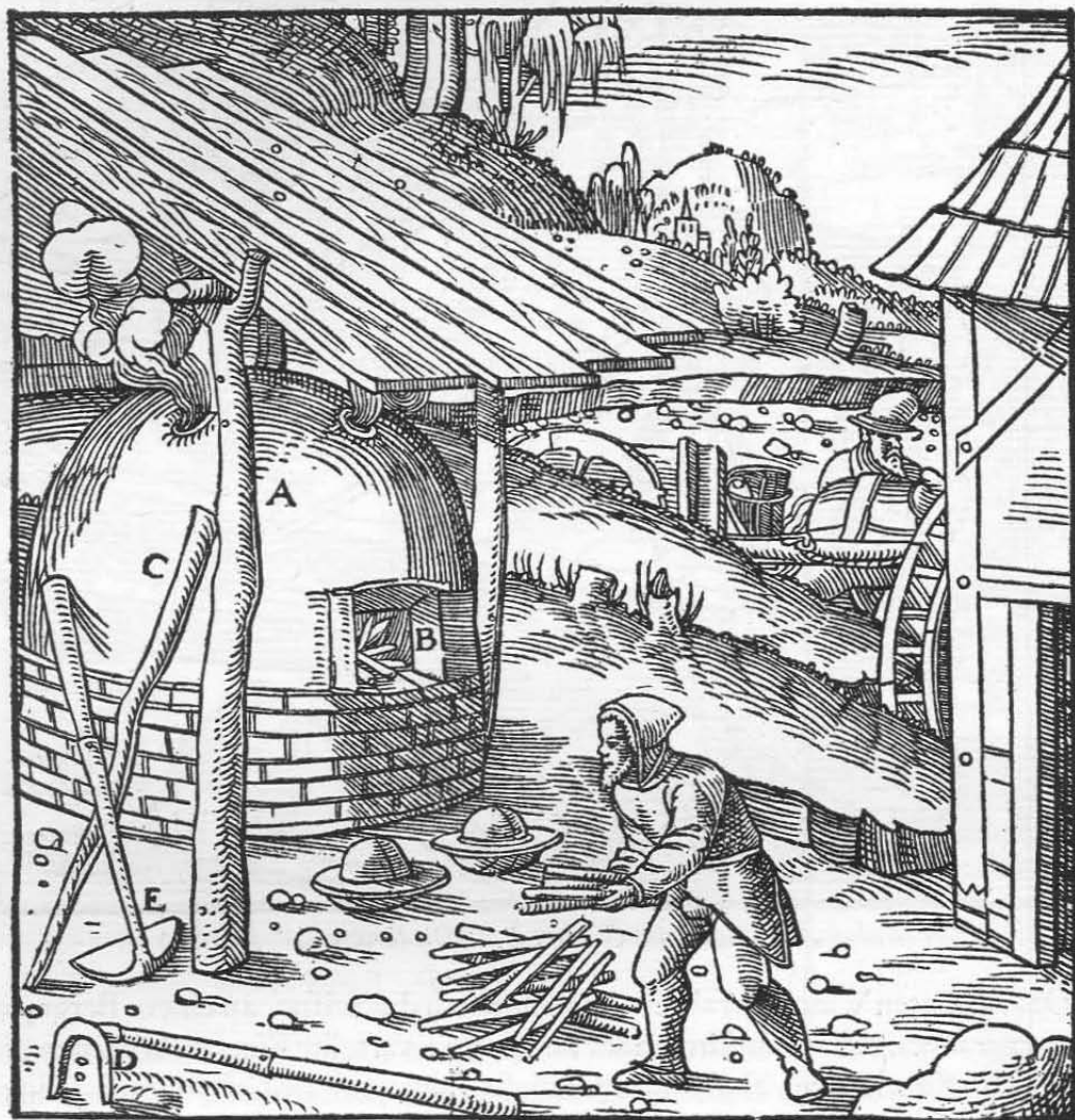
Der Ofen A. Die Eintragöffnung B. Die Schürflange C. Der Krähl mit zwei Zinken D. Die Krücke E.
