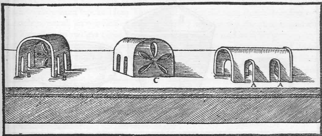
Die schmalen Fenster der Muffel A. Breite Fenster B. Die Öffnungen in der Rückwand C.
