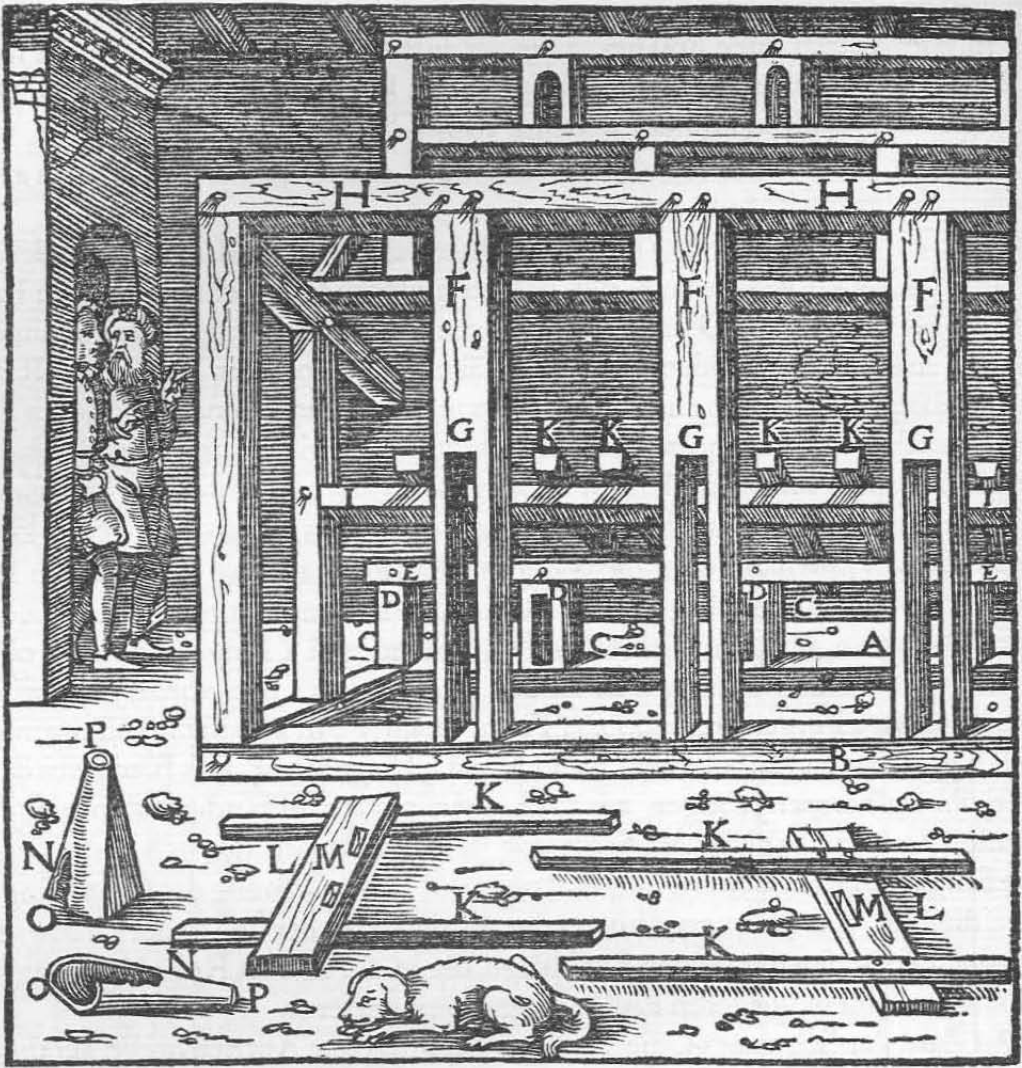
Die vordere der auf dem Erdboden liegenden Schwellen A. Die hintere Schwelle B. Die vorderen senkrechten Säulen C. Ihre Ausschnitte D. Die vordere Querschwelle E. Die hinteren senkrechten Säulen F. Ihre Ausschnitte G. Die hintere Querschwelle H. Der in die senkrechten Säulen eingezapfte Querbalken I. Die kurzen Balken K. Die Bretter L. Ihre Ausschnitte M. Das Rohr N. Sein hinteres Ende O, sein vorderes Ende P.
