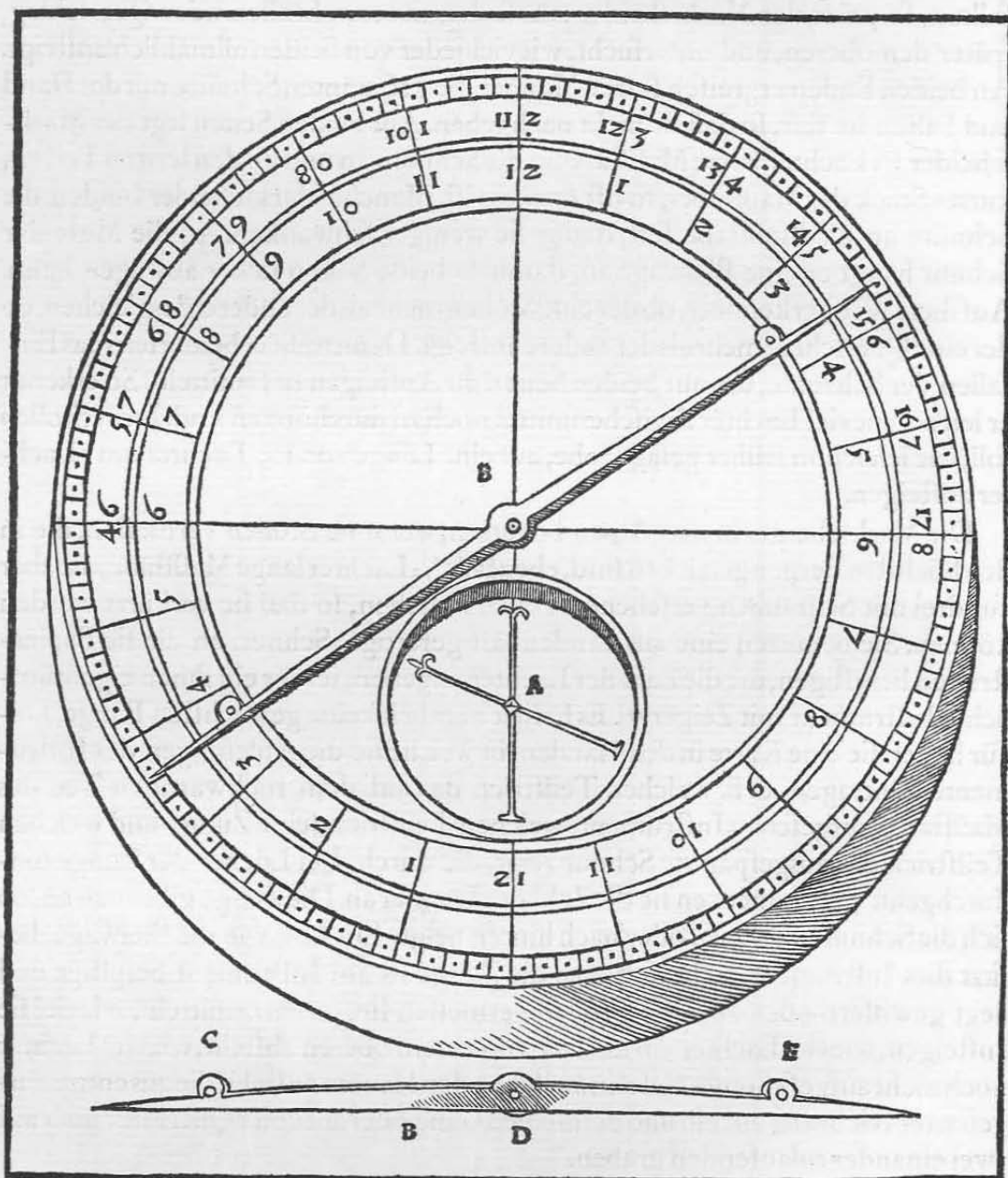
Der Zeiger des Instrumentes A. Seine Zunge B. Deren Löcher C, D und E.
