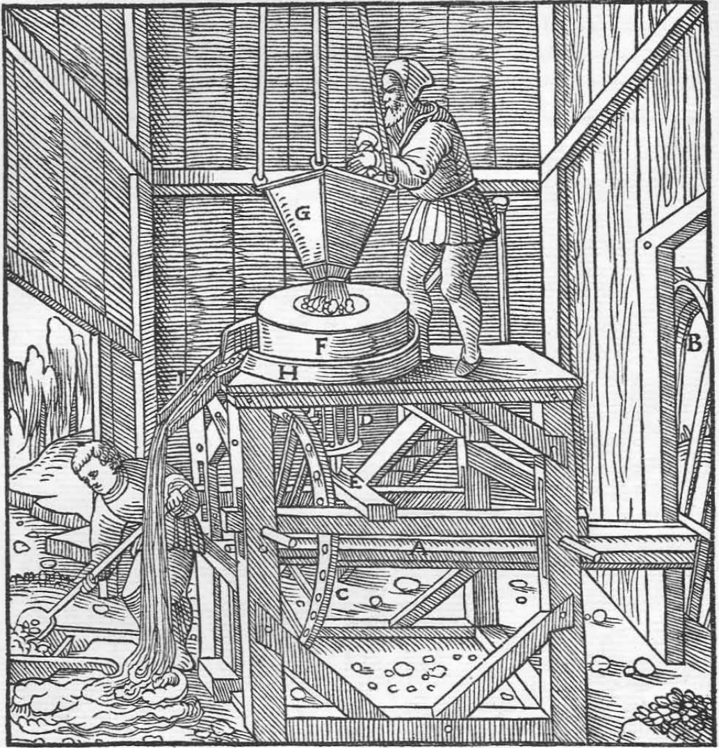
Die Wasserradwelle A. Das Wasserrad B. Das Kammrad C. Das Getriebe D. Seine eiserne Welle E. Der obere Mühlstein F. Der Trichter G. Das hölzerne runde Gerinne H. Der Austrag I.
