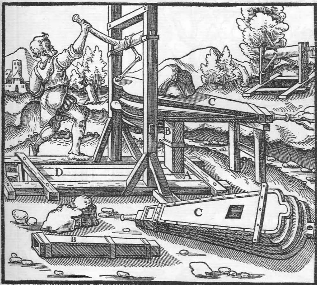
Der engere Teil des Schachtes A. Die rechteckige Lutte B. Der Blasebalg C. Der weitere Teil des Schachtes D.
