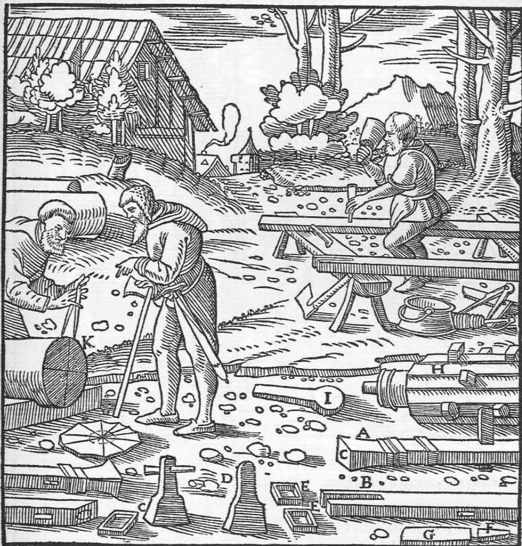
Ein Stempel mit Pochschuh A. Ein unten ausgeschnittener Stempel B. Der Pochschuh C. Ein anderer Pochschuh D 15) . Rechteckige Eisenringe E. Ein Keil F. Ein Hebling G. Die eckige Welle H. Ein Däumling I. Der Zirkel K.
