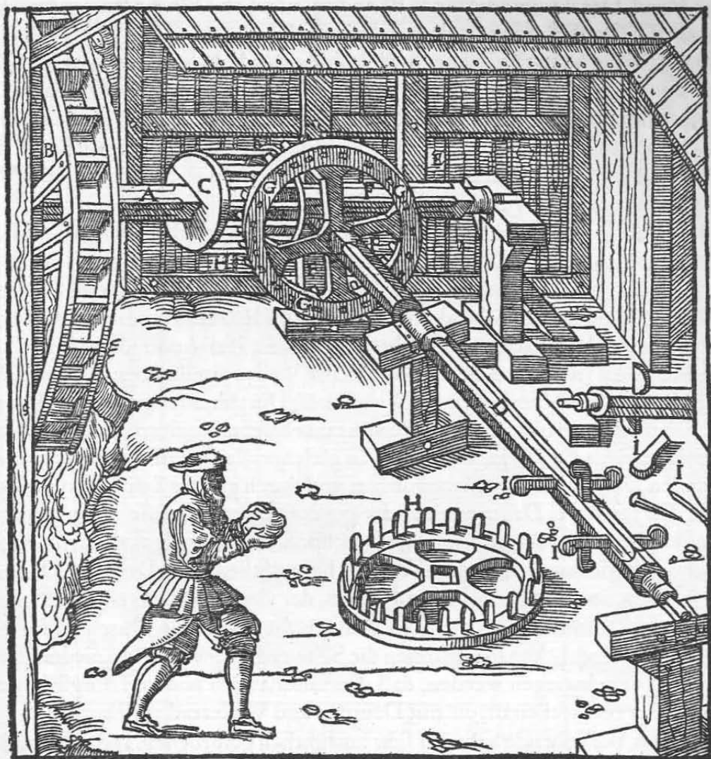
Die erste Welle A. Das Wasserrad B. Das mit Spillen versehene Vorgelege C. Die zweite Welle D. Das mit Zähnen versehene Rad E. Seine Speichen F. Seine Felgen G. Seine Zähne H. Die Daumen der Welle I.
