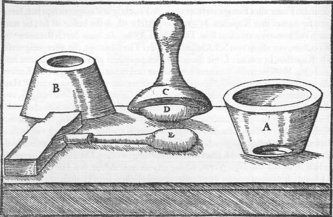
Preßform A. Umgedrehte Preßform B. Pistill C. Der Höcker des Pistills D. Ein anderes Pistill E.
