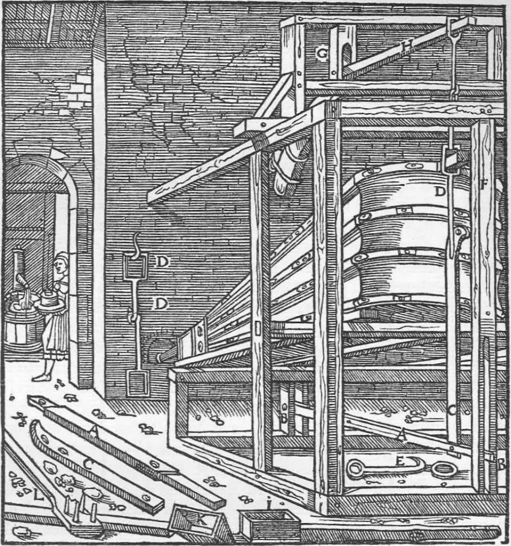
Schwengel, der durch die Daumen der Welle herabgezogen wird, wodurch der Blasebalg zusammengedrückt wird A. Der Ausschnitt der senkrechten Säulen B. Die Zugstange C. Die eiserne Vorrichtung mit dem rechteckigen Ring D. Die Vorrichtung mit dem runden Ring E. Der Balgsterzel F. Der kurze senkrechte Balken G. Die durch ihn hindurchgeführte Stange H. Kästen von gleichmäßiger Weite I. Nach unten sich verengernder Kästen K. Die in der Stange befestigten Eisenstäbe L.
