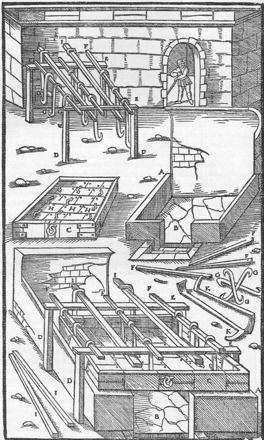
Der Herd A. Das Ofenloch B. Die Pfanne C. Die in die Erde eingegrabenen Balken D. Die darübergerlegten Querbalken E. Die kürzeren Latten F. Die kleinen Eisenhaken G. Die Öfen H. Die langen Latten I. Die größeren Eisenhaken K.
