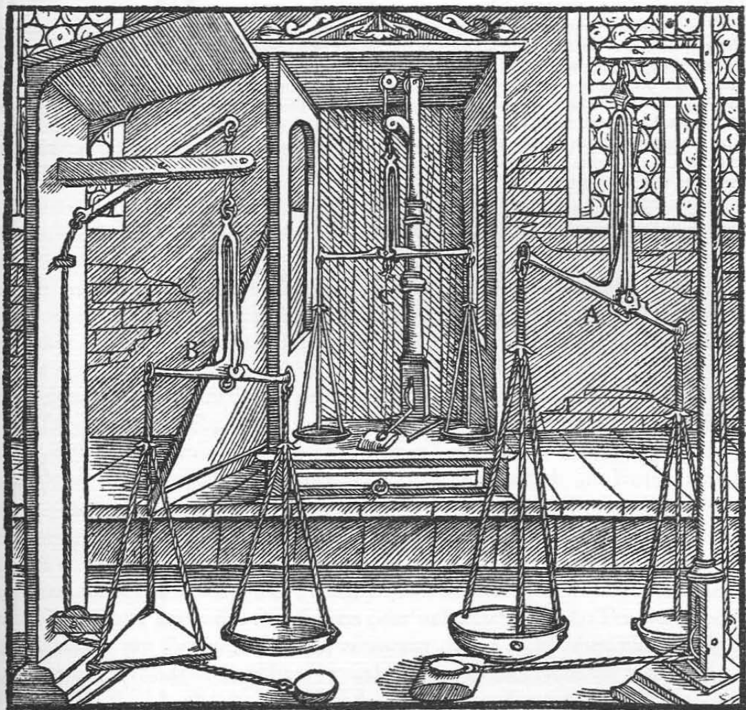
Die erste der kleinen Wagen A. Die zweite B. Die dritte, die in einem Gehäuse steht C.
