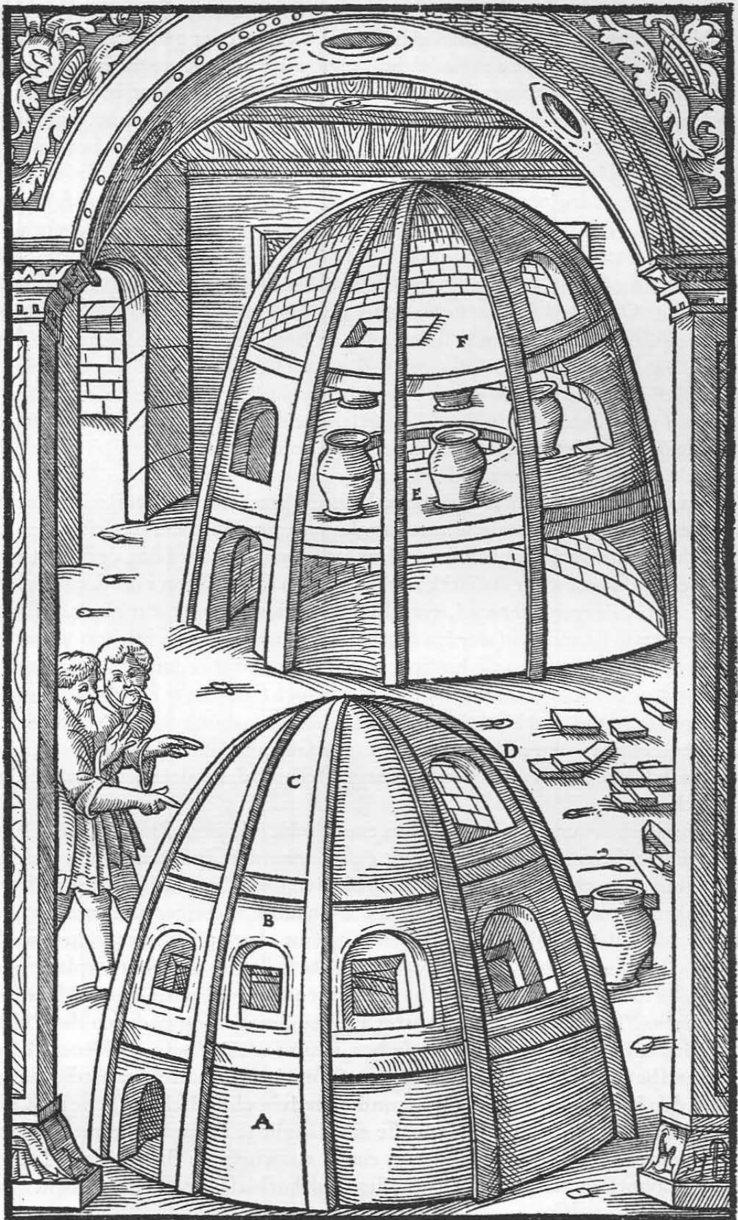
Die untere Kammer eines anderen zweiten Ofens A. Die mittlere Kammer B. Die oberste Kammer C; deren Fenster D. Die runde Öffnung E. Die viereckige Öffnung F.
