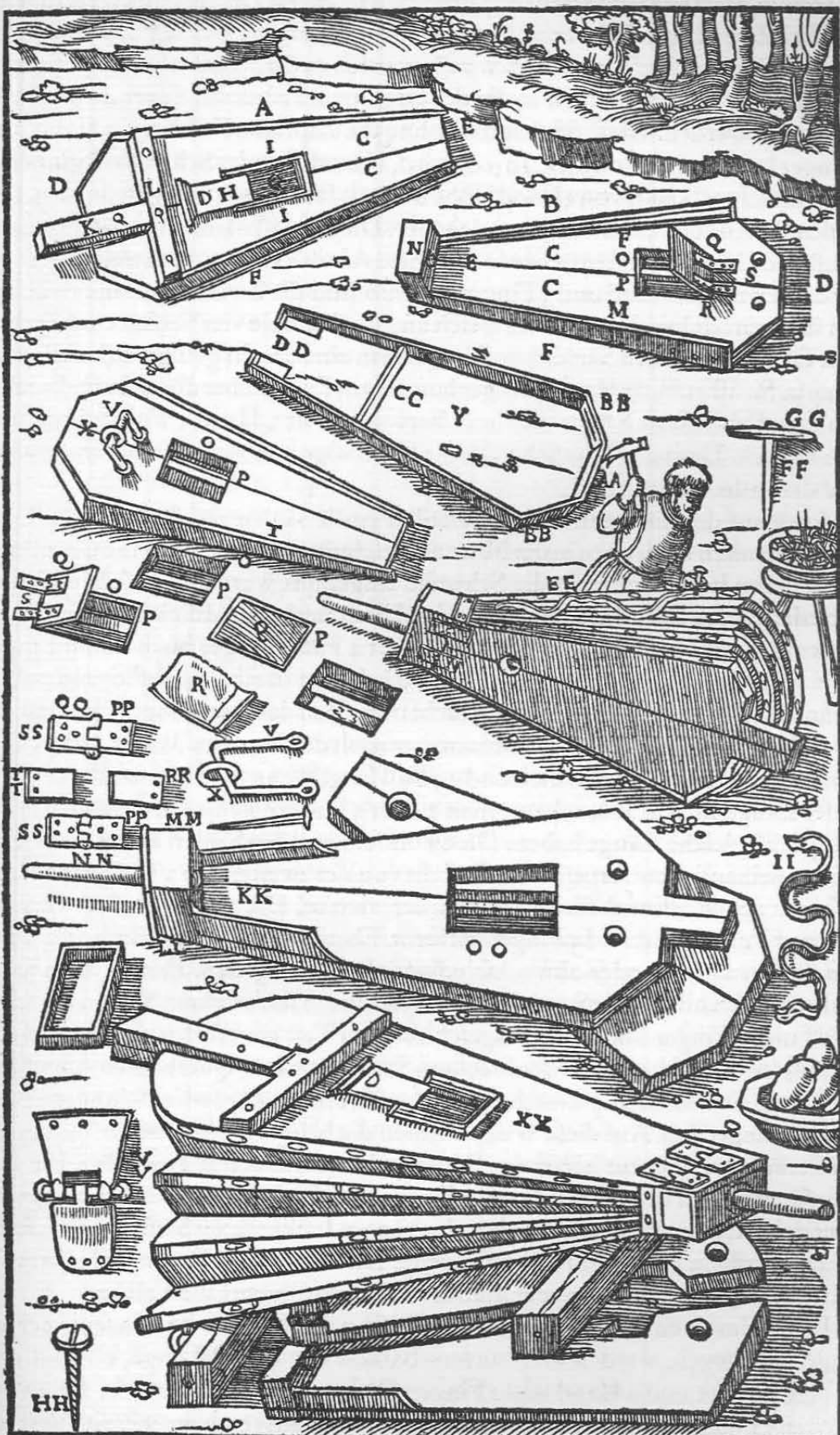
Das Deckelbrett des Blasbalges A. Das Bodenbrett B. Die zwei Bretter, aus denen Boden- oder Deckelbrett bestehen C. Der abgerundete hintere Teil D. Der vordere schmälere Teil E. Die Leisten F. Die Öffnung im Deckelbrett G. Ihr Deckel H. Dessen Rahmen I. Der Ansatz K. Die äußere Querleiste L. (Die innere ist nicht zu sehen.) Der innere Teil des Bodens M. Teil des Hauptes N. Die Windöffnung O. Der Steg P. Der Deckel Q. Das Leder R. Der Riemen S. Der äußere Teil des Bodenbrettes T. Die Klammer V. Der eiserne Ring X. Der Boden Y. Seine langen Leisten Z. Die hintere Leiste AA. Die gebogenen Leisten BB. Die lange Spreize CC. Die kurzen Leisten DD. Das Leder EE. Der Tförmige Nagel FF. Sein Kopf GG. Die Schraube HH. Langer Riemen II. Das Balghaupt KK. Seine Unterseite LL. Seine Oberseite MM. Der volle Boden OO. Die zwei äußeren Eisenplatten des Hauptes PP. Ihr umgebogener Teil QQ. Die mittlere Eisenplatte des Hauptes RR. Die beiden äußeren Platten des Deckels SS. Seine mittlere Platte TT. Seine Achse VV. Der fertige Blasbalg XX.
