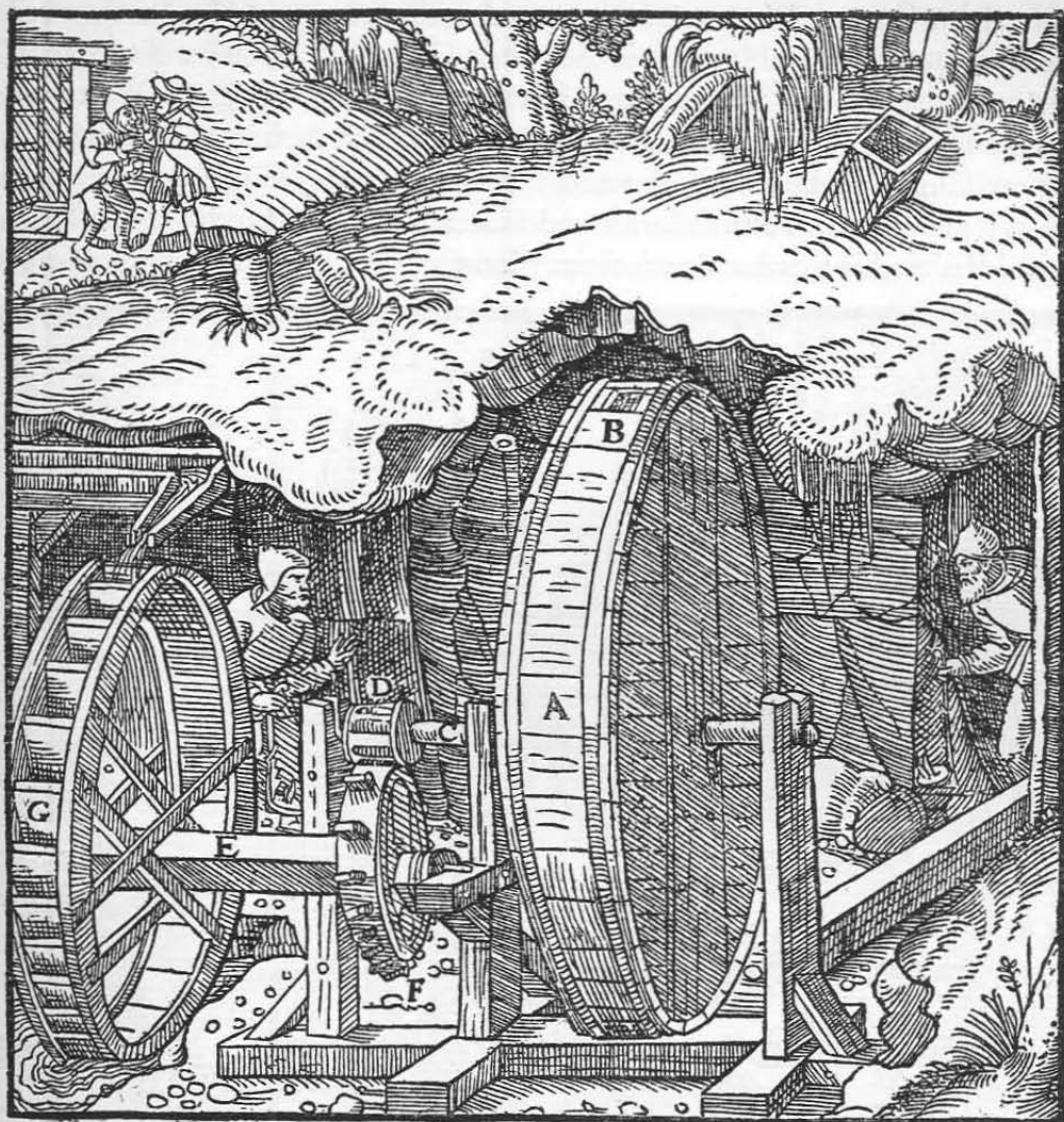
Die hohle Trommel A. Ihr Windloch B. Die Welle, auf der die Flügel sitzen C. Ihre Getriebe D. Die niedriger gelagerte Welle E. Das Zahnrad F. Das Wasserrad G.
