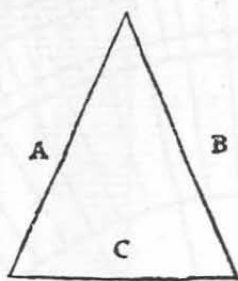
Gleichschenklig-spitzwinkliges Dreieck; die zwei gleichen Seiten A, B. Die ungleiche Seite C.
