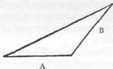
Gleichschenklig-stumpfwinkliges Dreieck; die gleichen Schenkel A, B.
