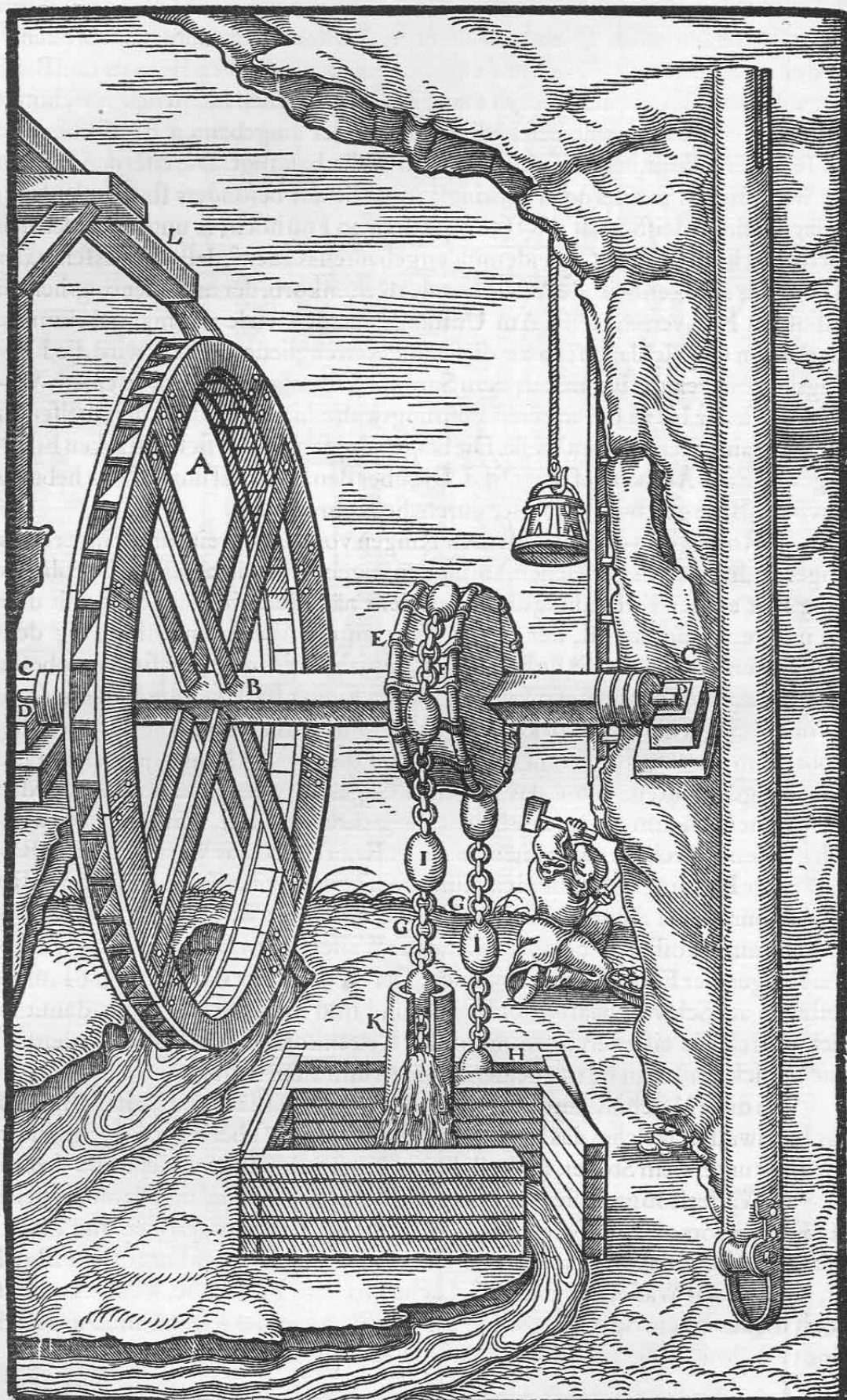
Das Rad A. Die Welle B. Die Zapfen C. Die Ringlager D. Der Kettenkorb E. Die eisernen Klammern F. Die Kette G. Die Schachthölzer H. Die Bälle I. Die Rohre K. Das Aufschlaggerinne L.
