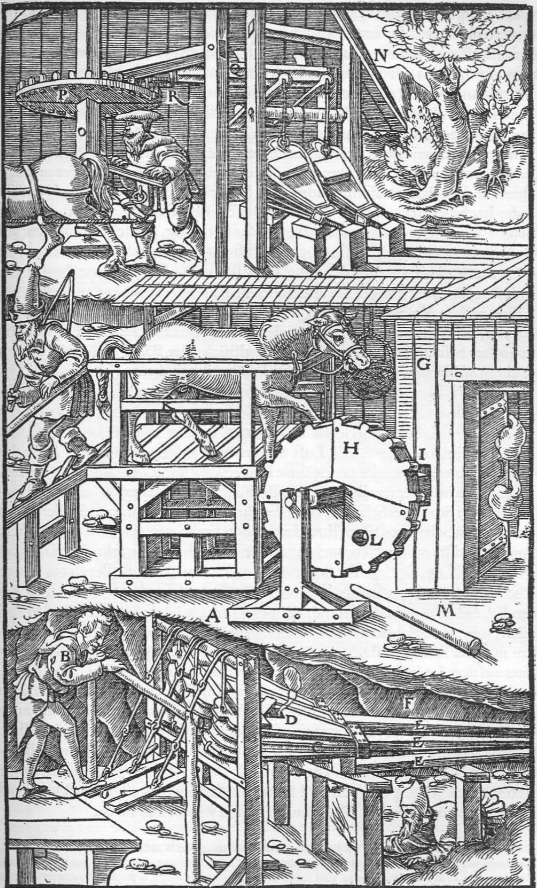
Die zuerst beschriebene Maschine A. Der Arbeiter, der durch Treten die Bälge zusammendrückt B. Die Bälge ohne Mundstücke C. Die Öffnung, durch welche die schweren Wetter oder die Luft ausgestoßen werden D. Die Lutten E. Der Stollen F. Die zweite beschriebene Maschine G. Die hölzerne Trommel H. Ihre Stufen I. Die Umzäunung K. Das runde Loch in der Trommel L. Die Stange M. Die dritte beschriebene Maschine N. Die stehende Welle O. Ihr Zahnrad P. Die liegende Welle Q. Ihr Getriebe R.
