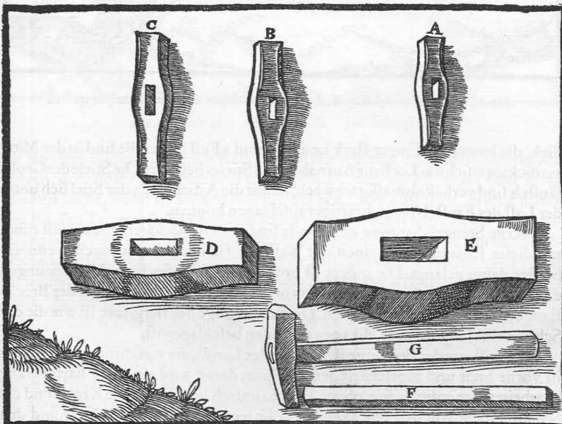
Das Ritzfäustel A. Das Handfäustel B. Das Treibefäustel C. Das zweihändige Treibefäustel D. Das Großfäustel E. Der hölzerne Stiel F. Der Stiel im Ritzfäustel G.
