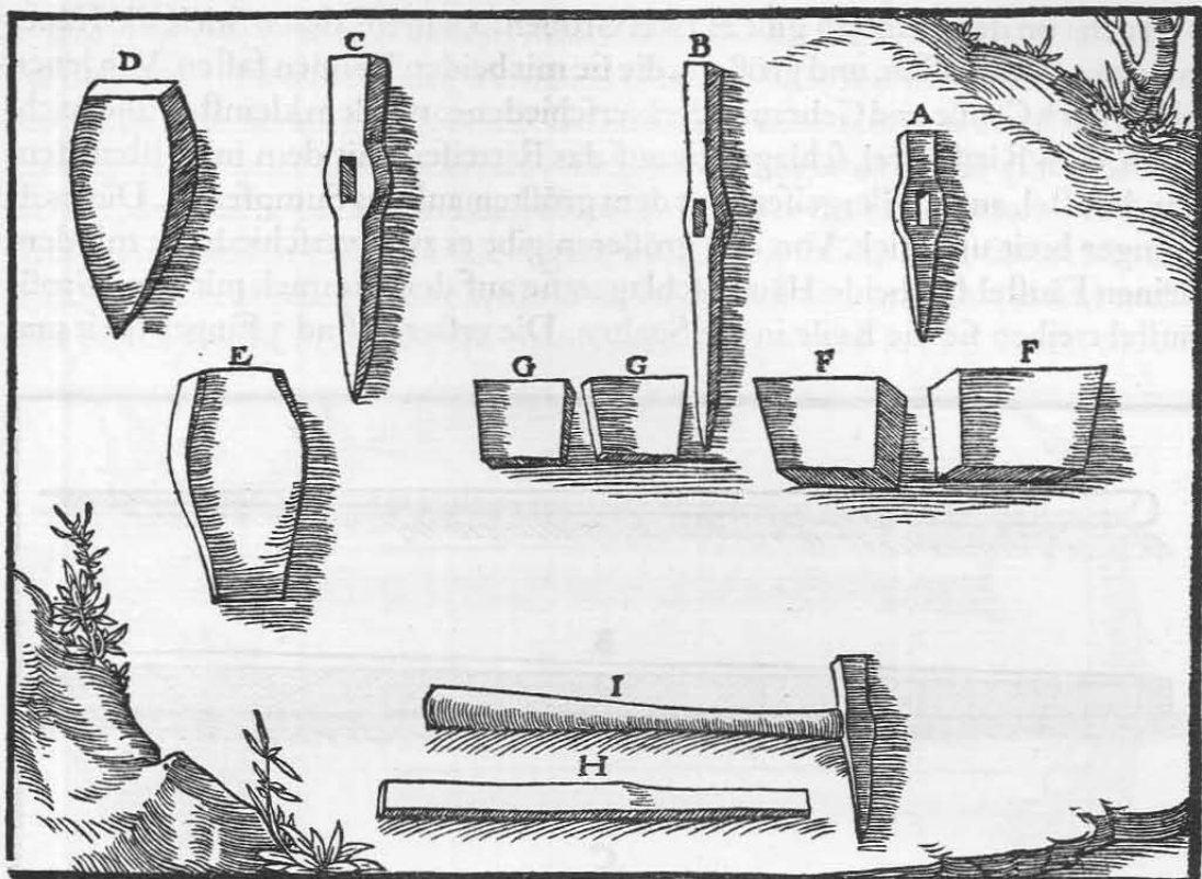
Das Bergesisen A. Das Ritzeisen B. Das Sumpfeisen C. Der Fimmel D. Der Keil E. Der Plötz F. Das Legeeisen G. Der hölzerne Stiel 2) H. Der im Bergesisen steckende Stiel I.
