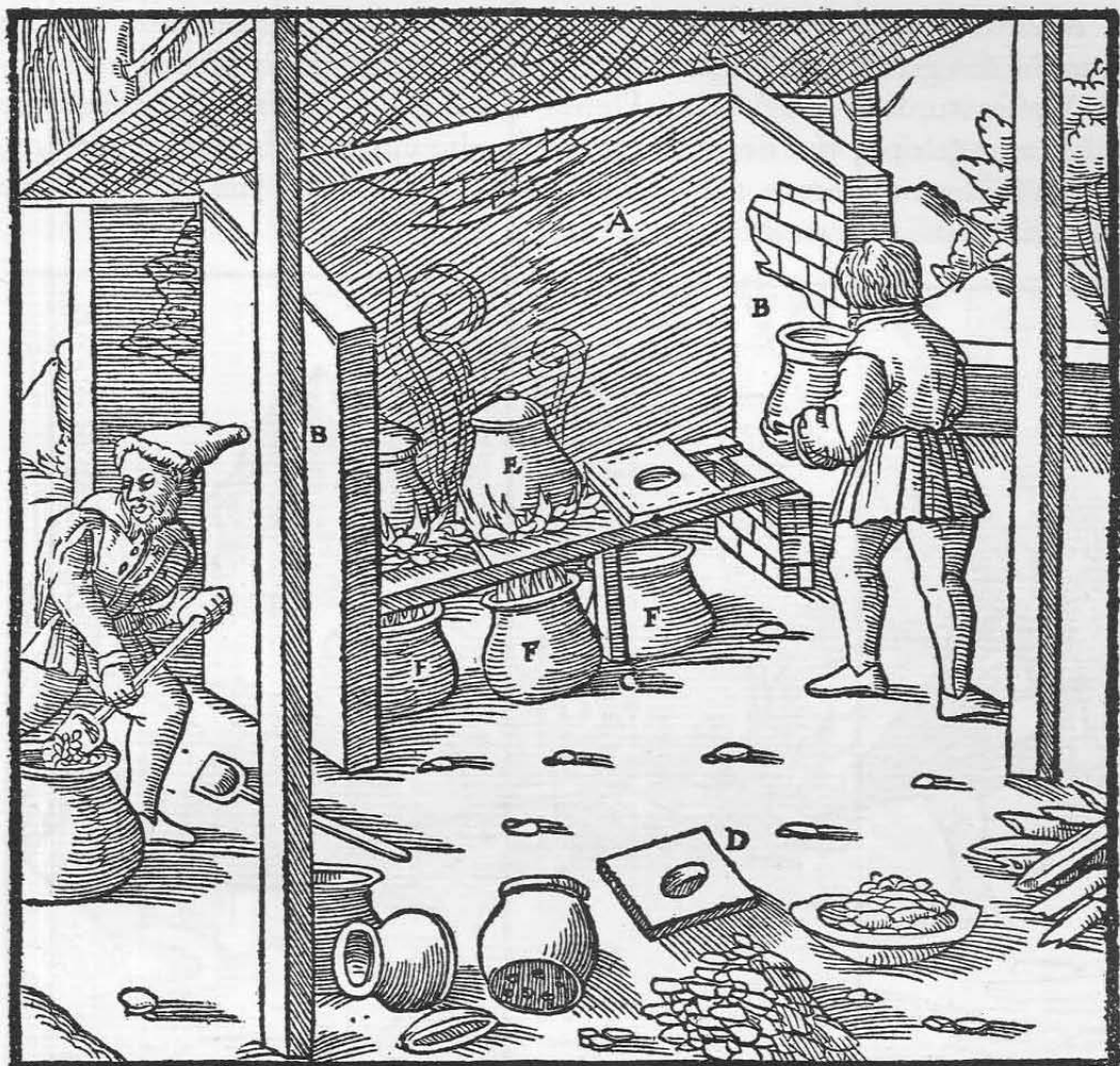
Die lange Mauer A. Die hohen Mauern B. Die niedrigen Mauern C. Eisenplatten D. Die oberen Töpfe E. Die unteren Töpfe F.
