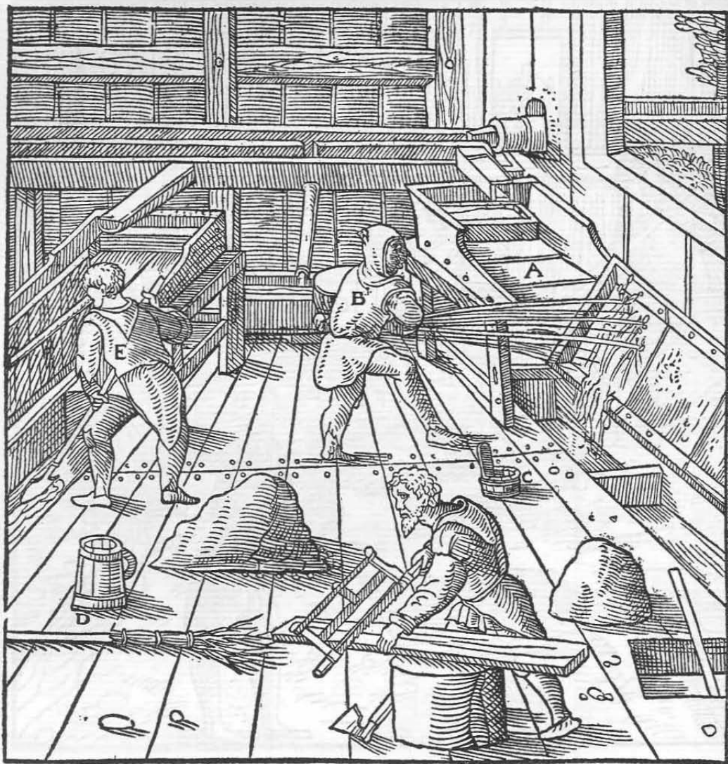
Der Herd A. Der Arbeiter, der das Wasser auf die Planen spritzt B. Die Kanne C. Eine andere Art von Kannen D. Ein Arbeiter, der das Erz oder die Graupen aus dem Graben aushebt E.
