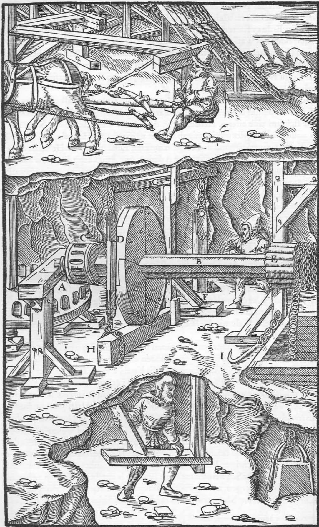
Das Kammrad an der stehenden Welle A. Die liegende Welle B. Das Getriebe C. Die Bremscheibe D. Der Seilkorb E. Der Bremschuh F. Der zweiarmige Hebel G. Der Bremsklotz H. Der Sturzhaken I.
