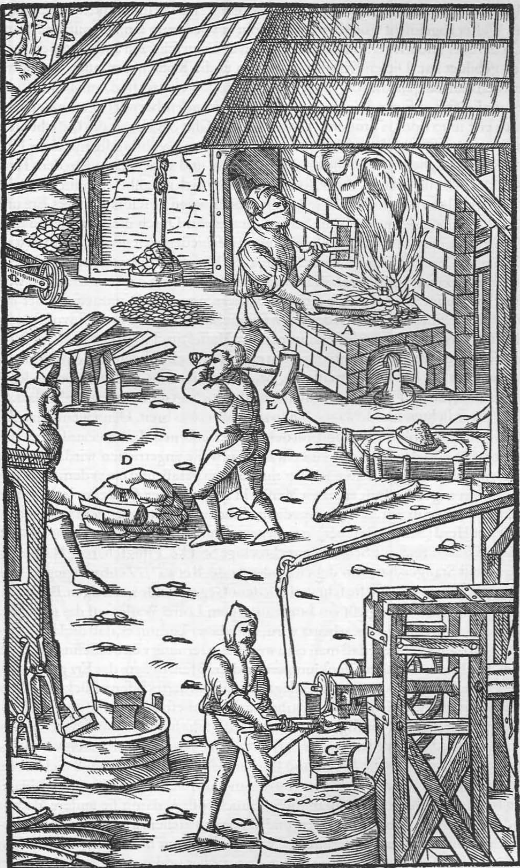
Der Herd A. Der Beschickungshaufen B. Der Schlackenabfluß C. Der Eisenklumpen (Masse) D. Die Holzhämmer E. Der große eiserne Hammer F. Der Amboss G.
