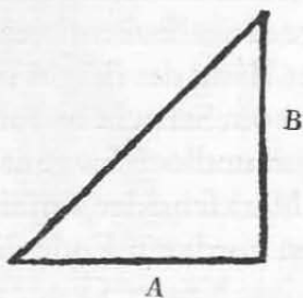
Gleichschenklig-rechtwinkliges Dreieck.
