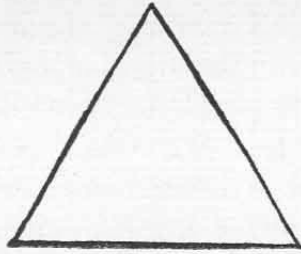
Gleichseitig-spitzwinkliges Dreieck.
