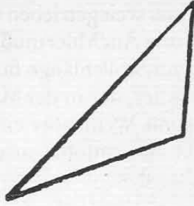
Ungleichseitig-stumpfwinkliges Dreieck.
