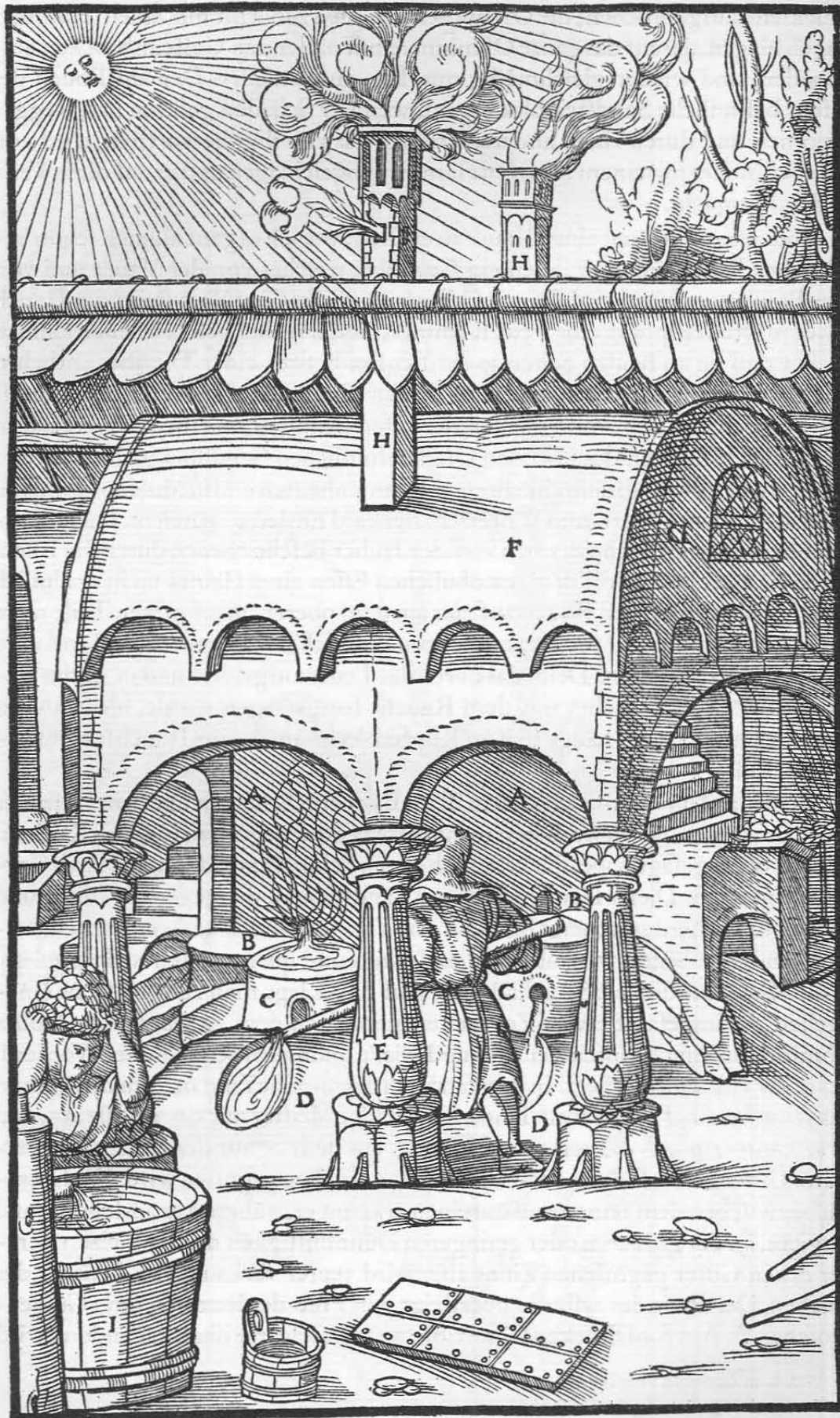
Die Öfen A. Der erste am Ofen befindliche Vorherd B. Sein Stich C. Der zweite Vorherd D. Die Pfeiler E. Die Flugstaubkammer F. Fenster G. Die Rauchfänge H. Gefäß, in dem die Kohlen gewaschen werden I.
