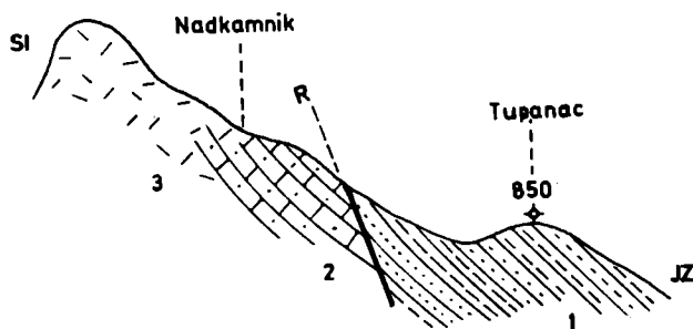
Профил 1. Геолошки односи код села Мојинаца. — 1. Лијаски лапорци и пешчари; 2. Догерски бречастии песковити кречњаци; 3. Малмски нестратификовани кречњаци; Р. Мојиначки расед.
