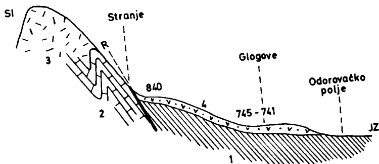
Профил 3. Морфолошки односи код Јанковог дола изнад села Смитовци. — 1. Покривени лијас; 2. Танкопложасте убрани догерски кречњаци; 3. Малмски нестратификовани кречњаци; 4. Дилувијалне и делувијалне насlage; Р. Смиловачки расед; 840 — 741. Абразиони нивои
