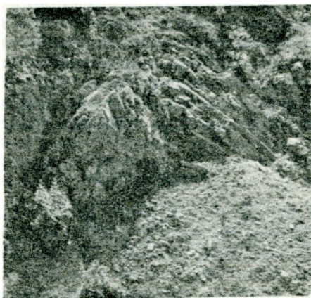
Сл. 1 Антиклинарна бора у Јанковом долу изнад водопада Рипало
