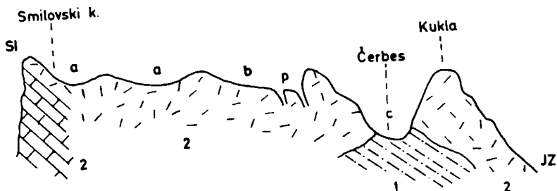
Профил 2. Геологија и морфологија Видлича изнад Чербеса. — 1. Лапорци и пешчари догера; 2. Нестратификовани и банковити кречњаци малма; а. Низ тањирастих вртача; б. Асиметрична вртача са понорима; ц. Циновска вртача Чербес.
