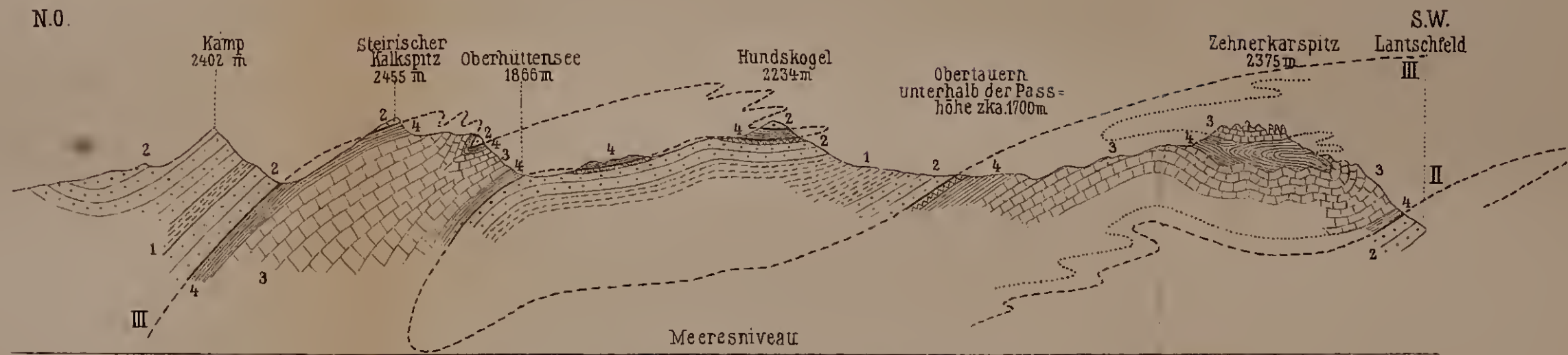
Fig. 4. Durchschnitt der Tauerndecke zwischen dem Lantschfeld, Obertauern und dem Lungauer Kalkspitz, etwas vereinfacht. Maßstab 1:75000.
