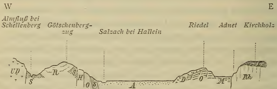
Profil durch den Salzachgraben nördlich von Hallein.
