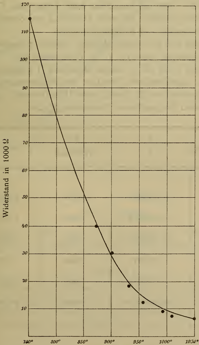
Fig. 3. Abkühlung des Adulars.
