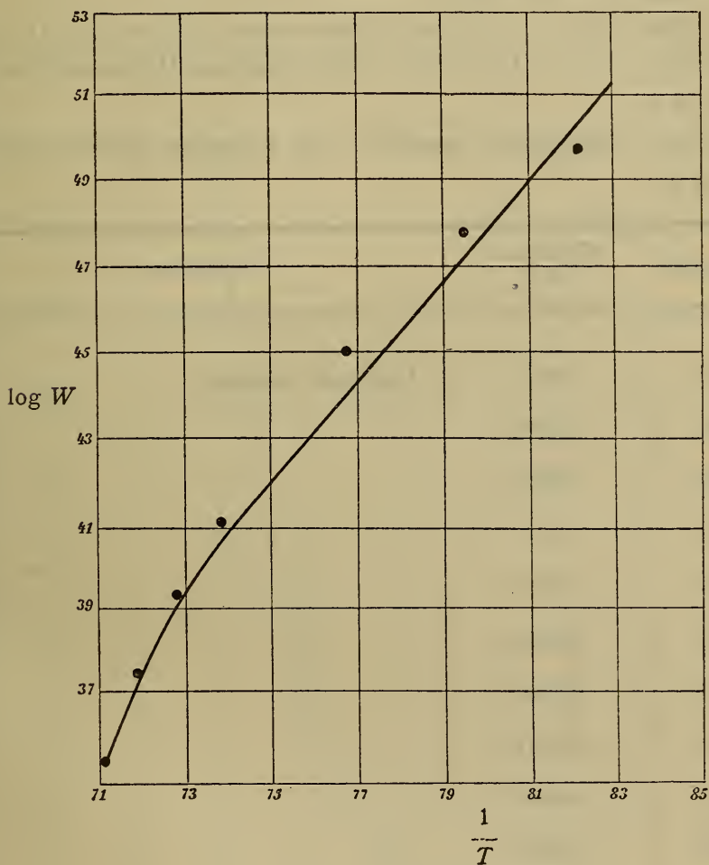
Fig. 4. Adular.
