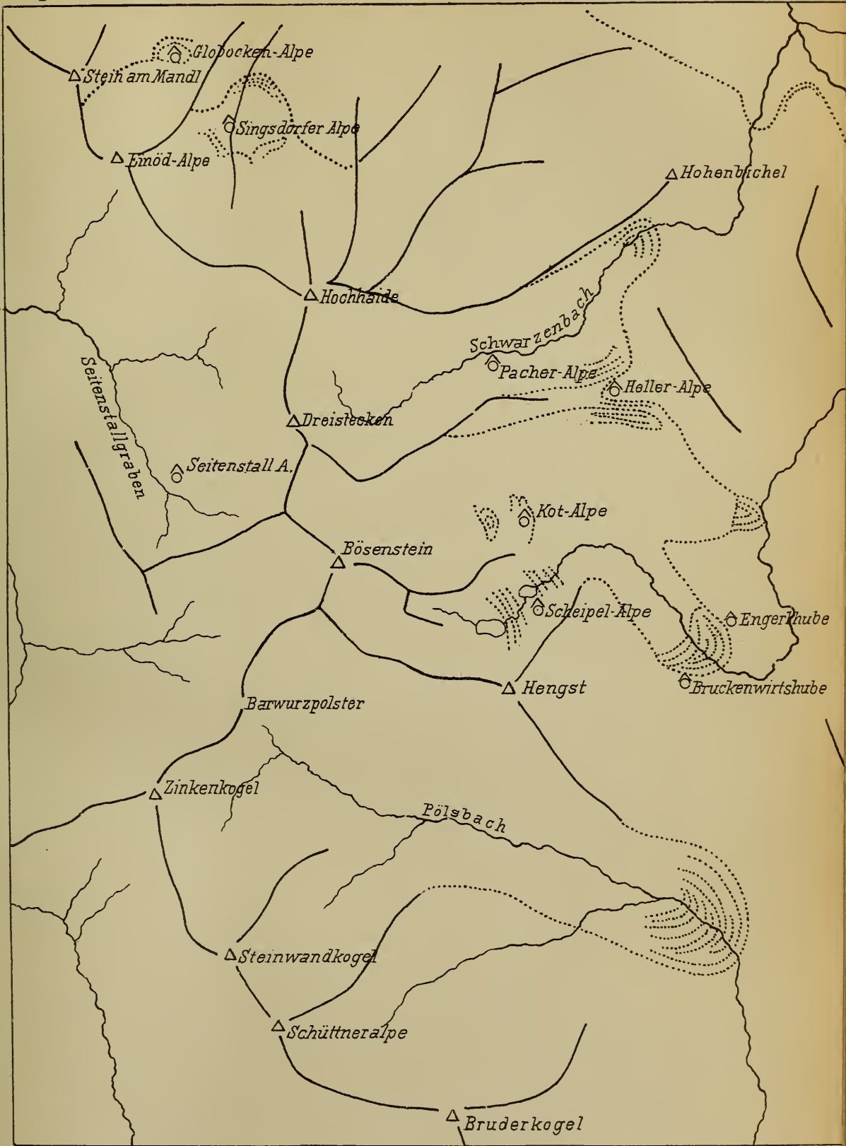
Die alten Gletscher der Bösensteingruppe
