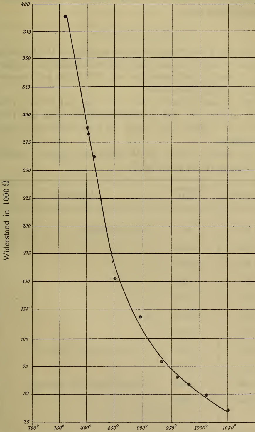
Fig. 5. Diopsid I.
