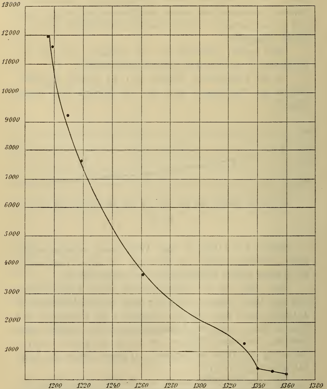
Fig. 6. Labradorit.
