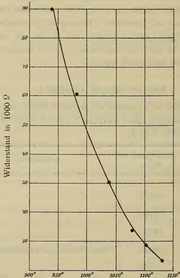
Fig. 2. Adular.
