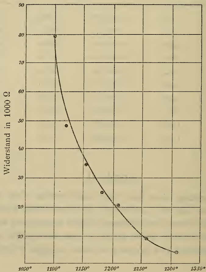
Fig. 8. Diopsid II.
