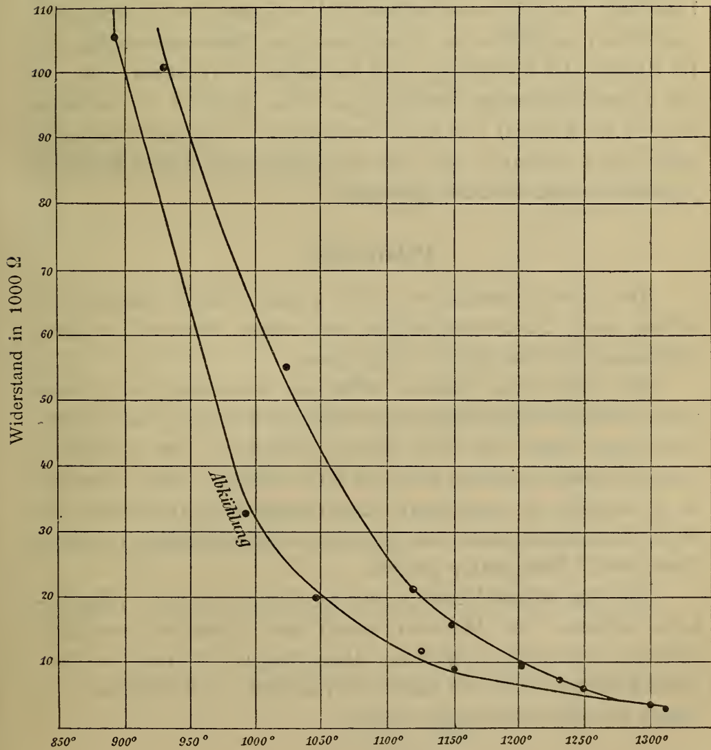
Fig. 9. Quarz.
