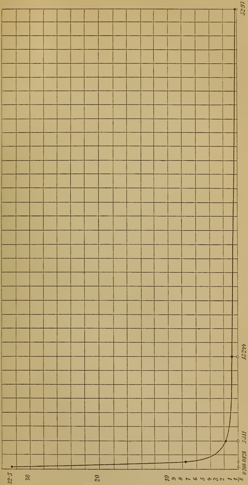
Kurve der heliotropischen Präsentationszeiten.
