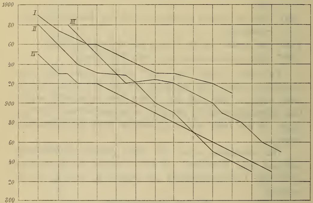
Fig. 2. Ägirin-Eläolith (Mineralgemenge).
