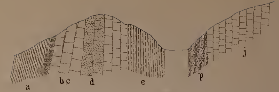
Fig. 2. Entwicklung der Juraformation an der tieferen Belemnitenfundstelle im Großwandkar (zwischen Großwand, Hirschwand und Pleislingkeil, Radstädter Tauern)
