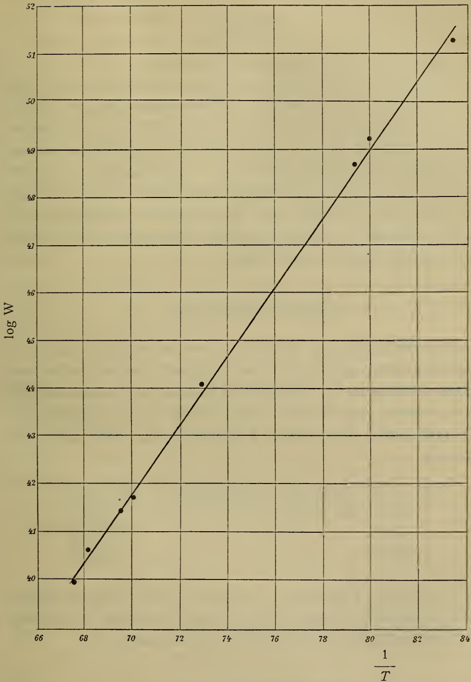
Fig. 11. Quarzglas.
