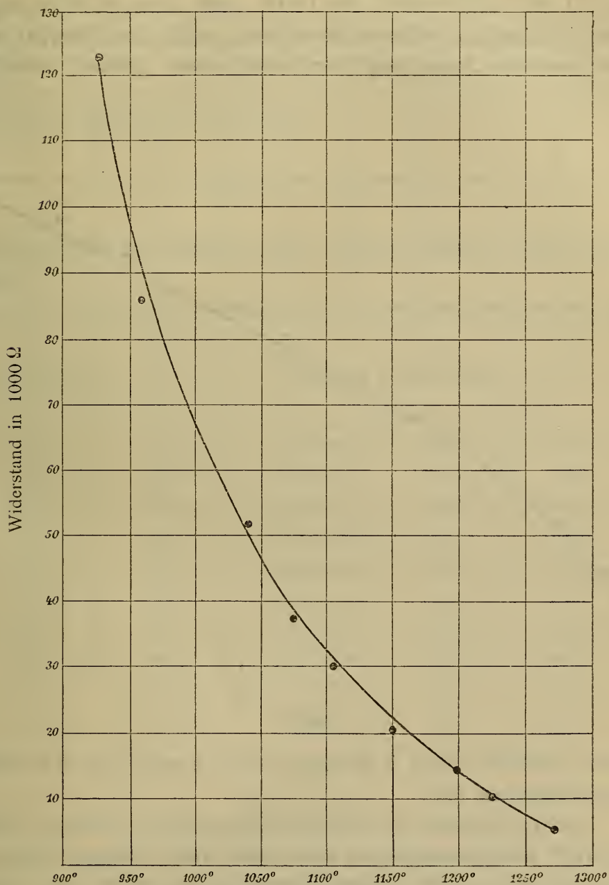
Fig. 6. Diopsid Ia.
