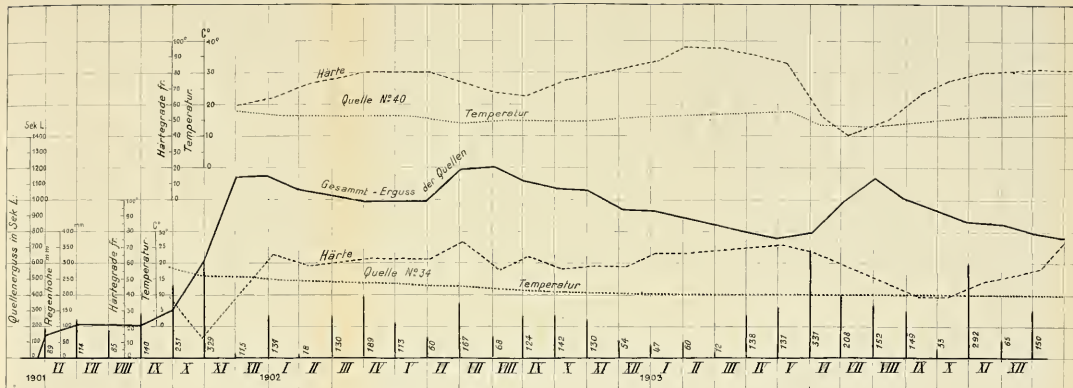
Fig. 11. Schwankungen des Gesamtergusses der kalten Quellen von Stieile zwischen km 3.860 u. 4.421, im Vergleich zur Regenmenge und der Temperatur- und Härte-Änderungen
