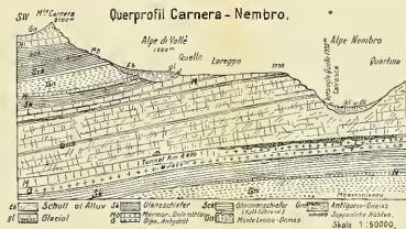
Fig. 12 u. 13. Querprofile durch die wasserführende Zone zwischen km 3.860 und 4.421 des südlichen Angriffs (Stieile)
