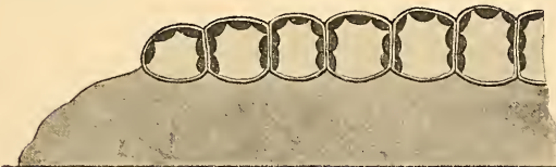
Fig. V. längere Zeit belichtet, resp. besontt
