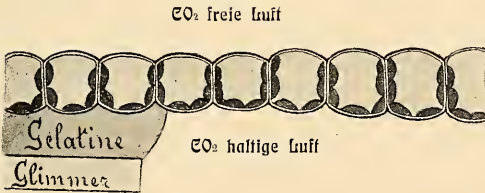
Fig. VIII. Querschnitt durch ein Funariablast das über ein Glimmerfenster geklebt und auf der einen Seite mit \text{CO}_2 freier, auf der andern Seite mit \text{CO}_2 haltiger Luft bespült worden war · Vergrösserung 340
