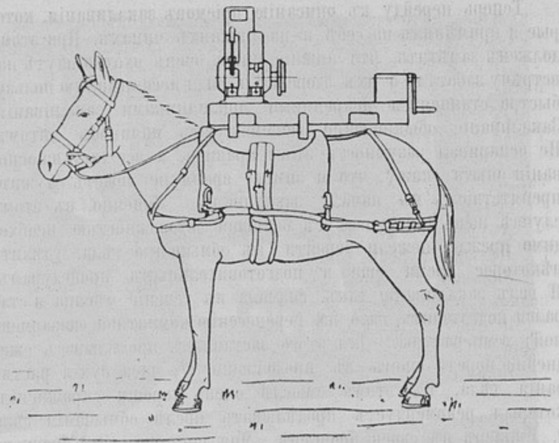
Рис. 2 Вьюкъ съ динамо и съ рамой.
