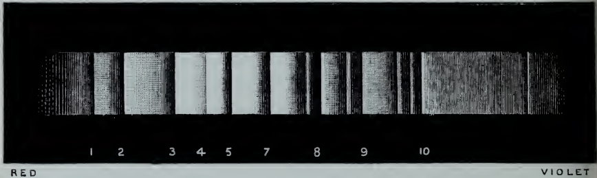
SPECTRUM OF MIRA CETI.
