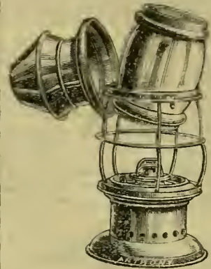
Linterna "Perfecta" de Anthony para placas secas.
