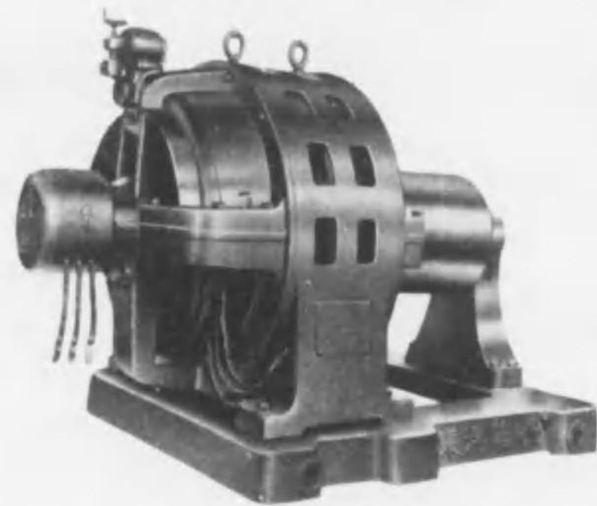
14 極 250 馬力 270-540 回轉每分 550 「ヴォルト」 0 「サイクル」
