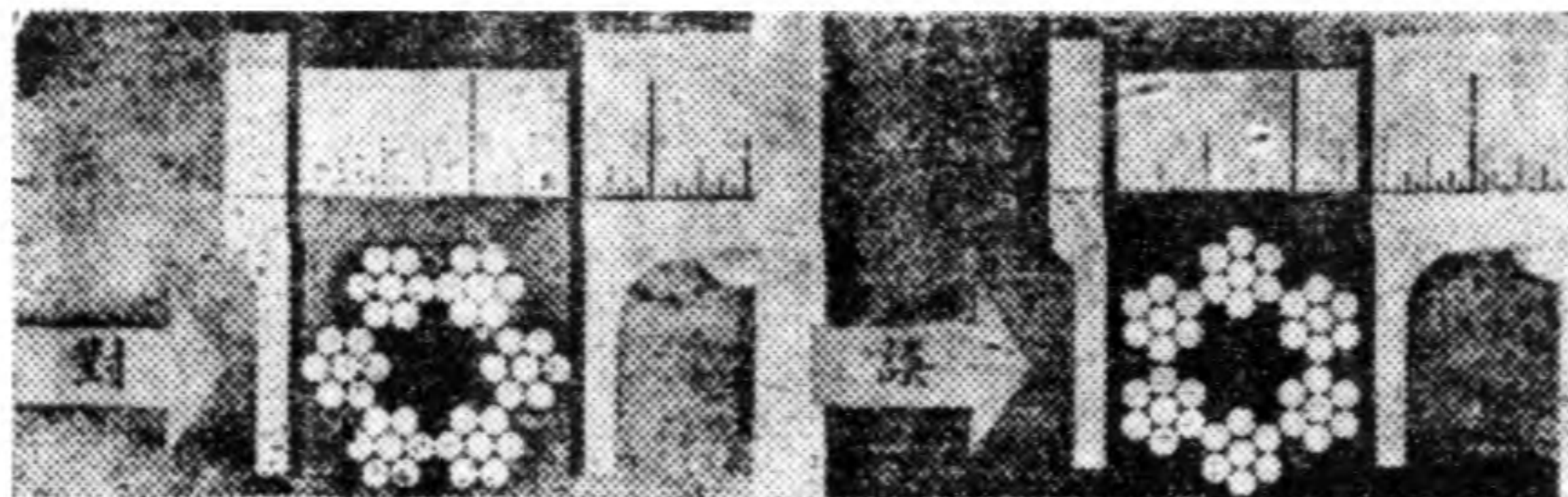
鋼索量計法
