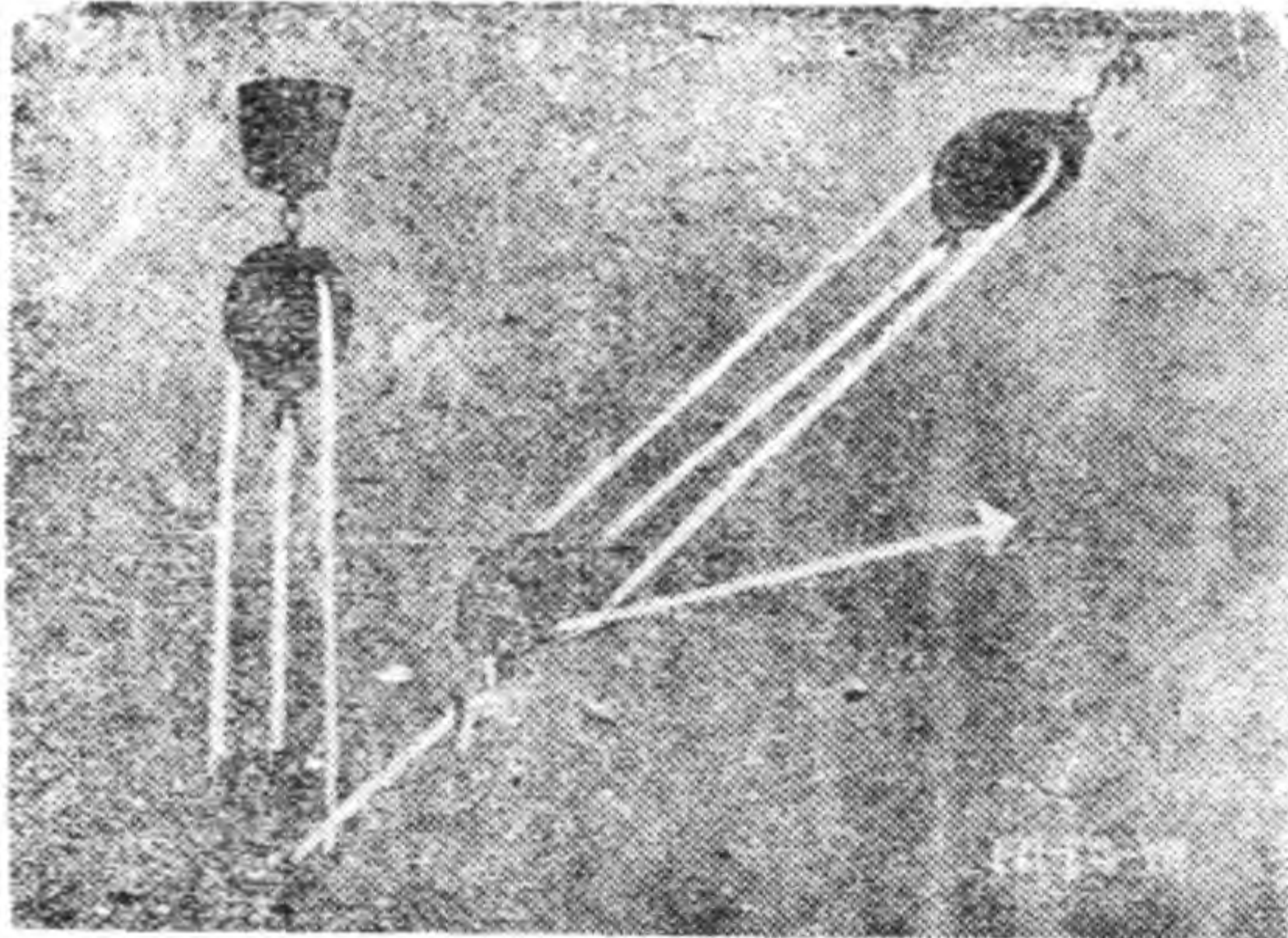
重疊大滑車
