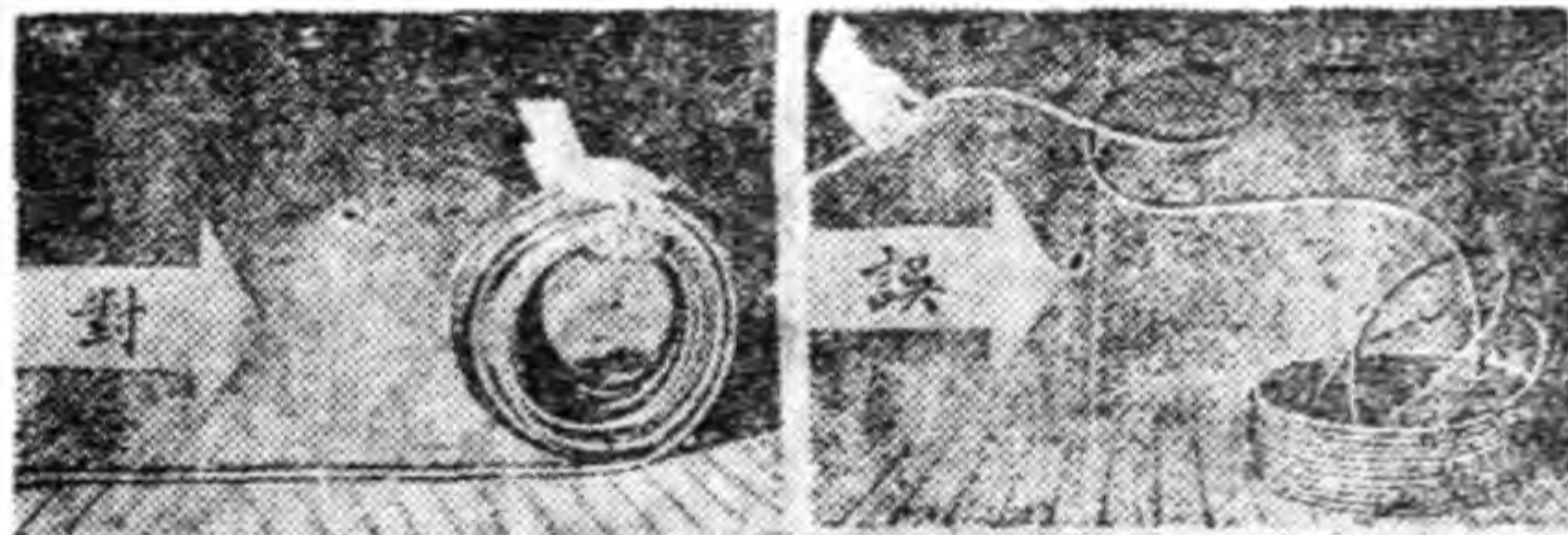
法 捲 開 索 網
