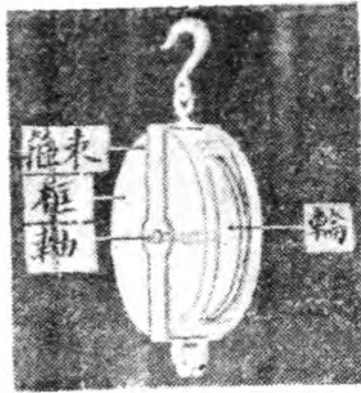
滑車各部分名稱
