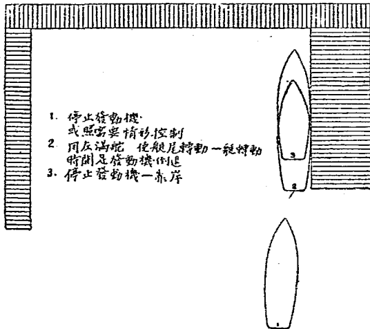
右 舷 靠 岸
