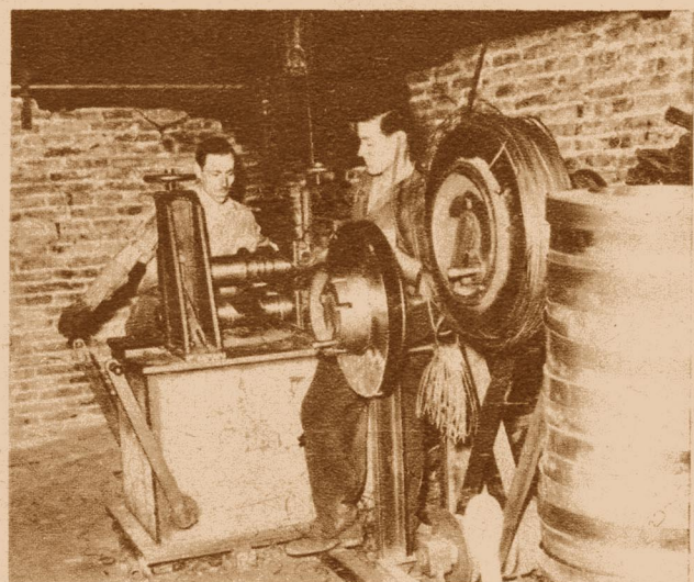
CORTANDO EL FLEJE. Una vez laminados los mismos, son cortados de acuerdo a las necesidades del consumidor. Esta máquina ha sido construída en el mismo taller, siendo su resultado magnífico y de gran rendimiento comparada a otras similares fabricadas en los más importantes centros industriales del mundo.
