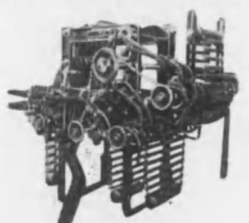
普通ドビー装置
