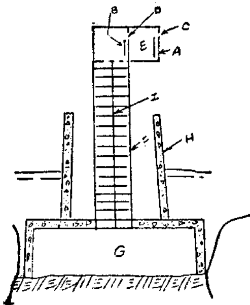
圖三 沉箱 氣閘和進管剖面圖
