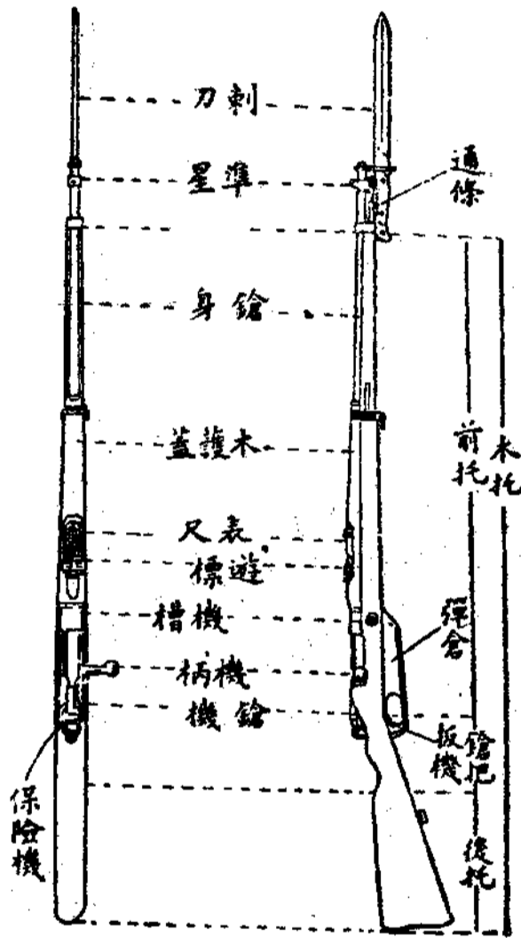
步鎗構造的一斑
