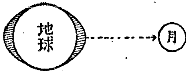
這個圖是表示大洋的水因月的亮的引力而發生海潮的漲落
