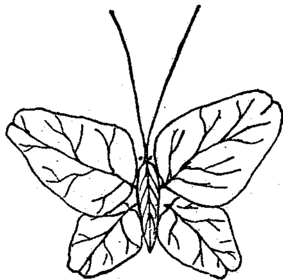
蝶 翅
