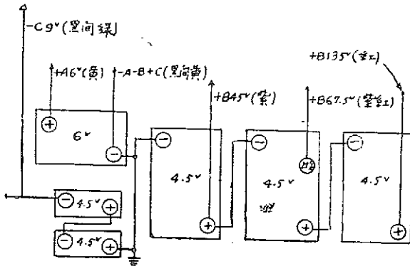
電池接綫 (圖二)
