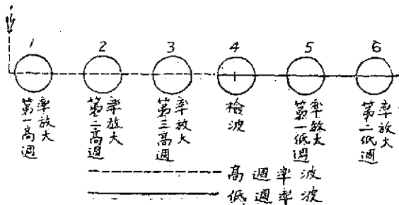
真空管順序及電波傳遞情形 (圖一)
