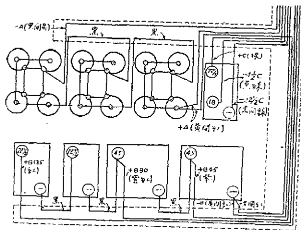
電池接綫(圖二)
