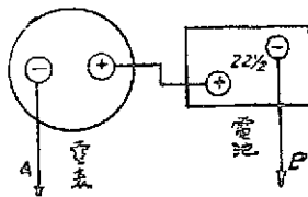
檢驗用電池電表接法 (圖三)
