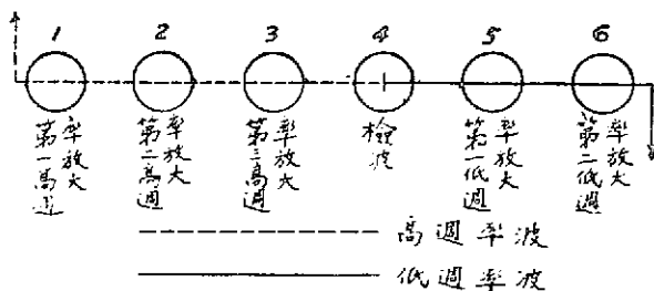
真空管順序及電波傳遞情形 (圖一)
