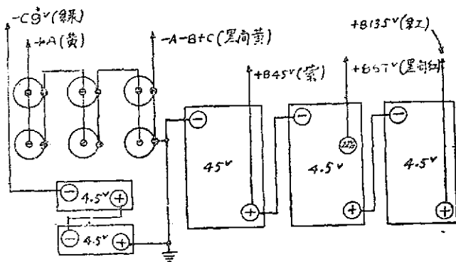
電池接綫 (圖二)
