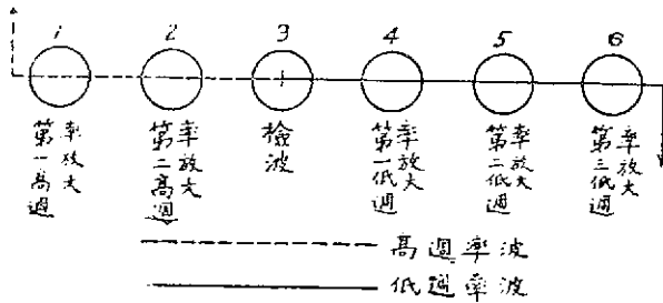
真空管順序及電波經過情形 (圖一)
