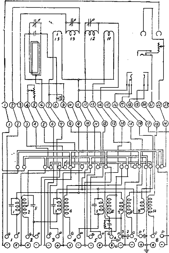
二十八號收音機線路 (圖五)
