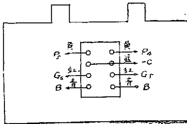
低週率變壓器(圖五)
