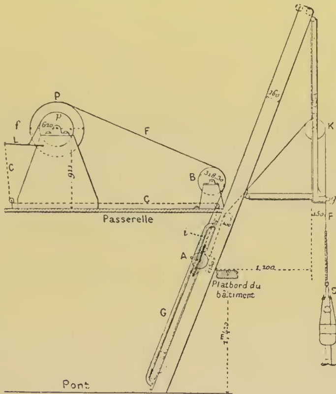
Fig. 63. — Machine à sonder du Talisman .
