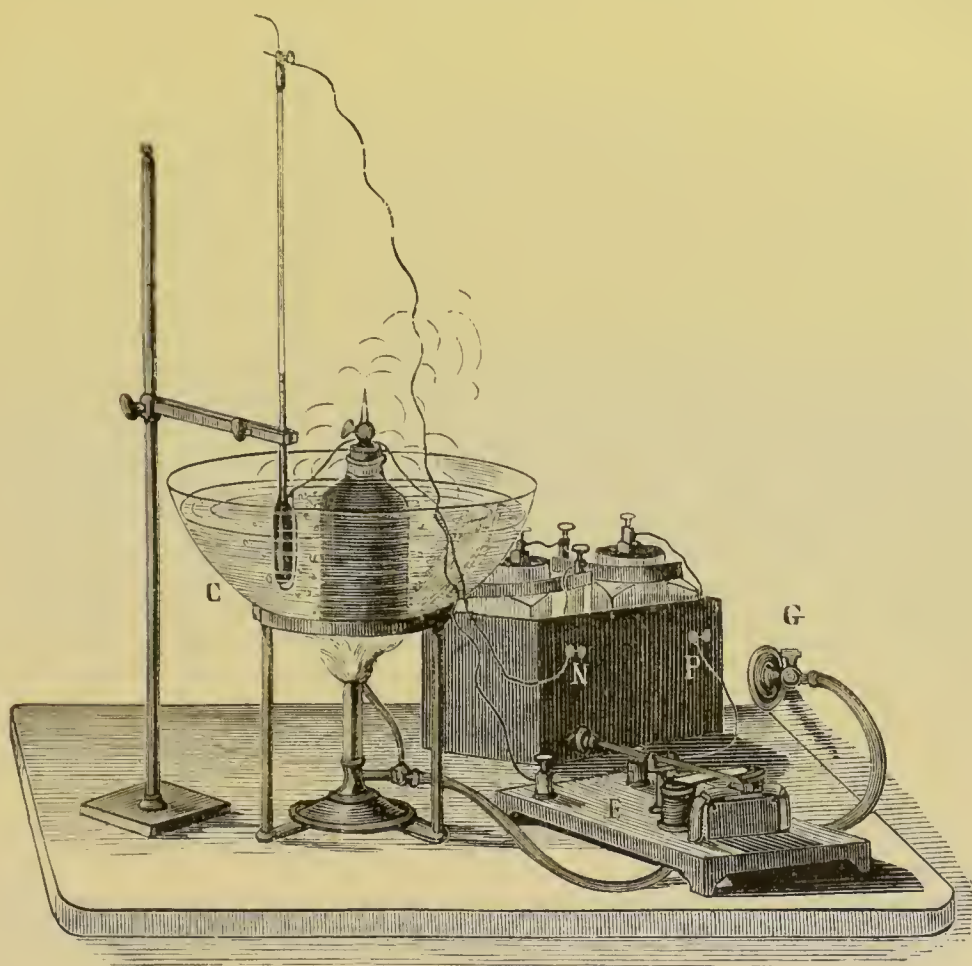
Fig. 78. — Thermostat électrique.
