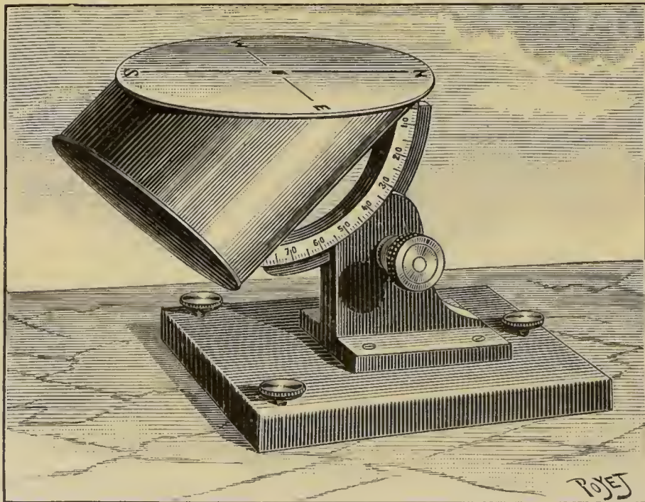
Fig. 100. — Héliographe de Maurer.
