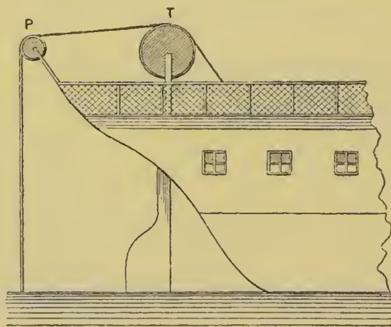
Fig. 59. — Compteur du sondeur Delacroix.
