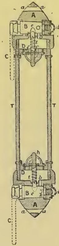
Fig. 170. — Bouteille du Talisman .
