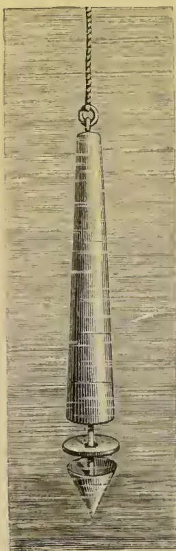
Fig. 52. — Sonde à coupe.
