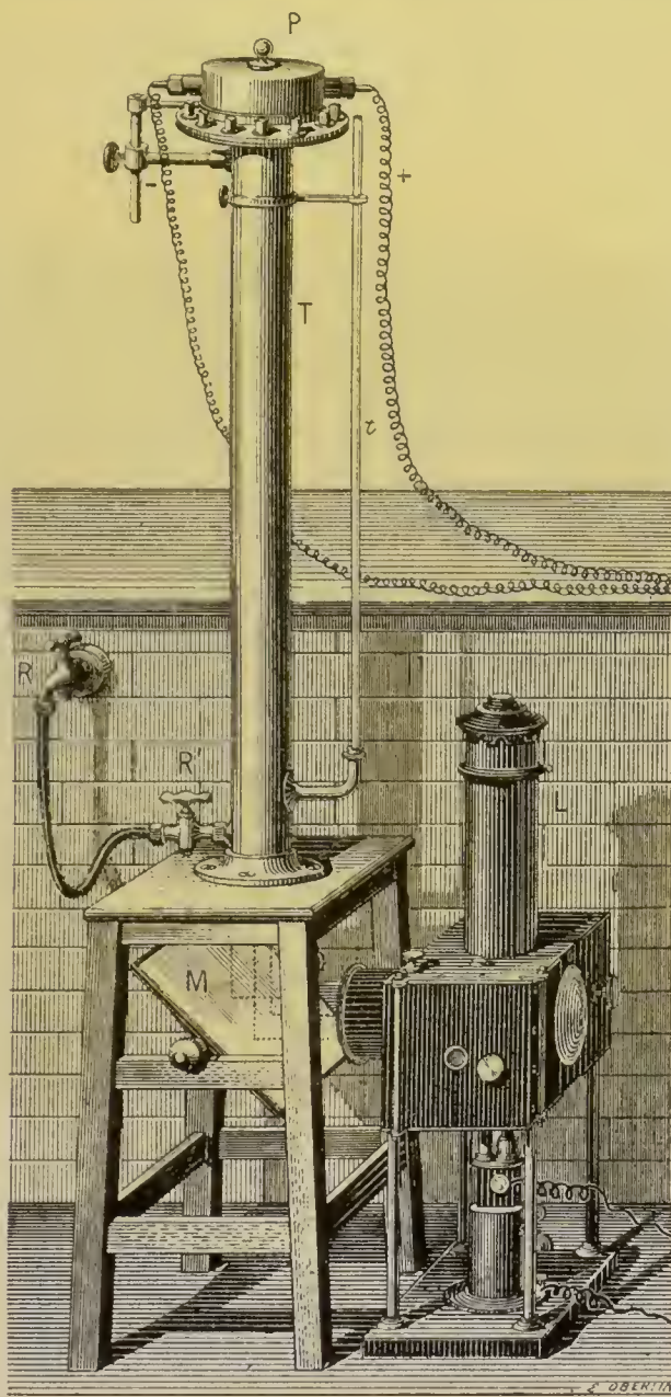
Fig. 108. — Dispositif destiné à mesurer l'absorption de la lumière par l'eau pure distillée ou filtrée.
