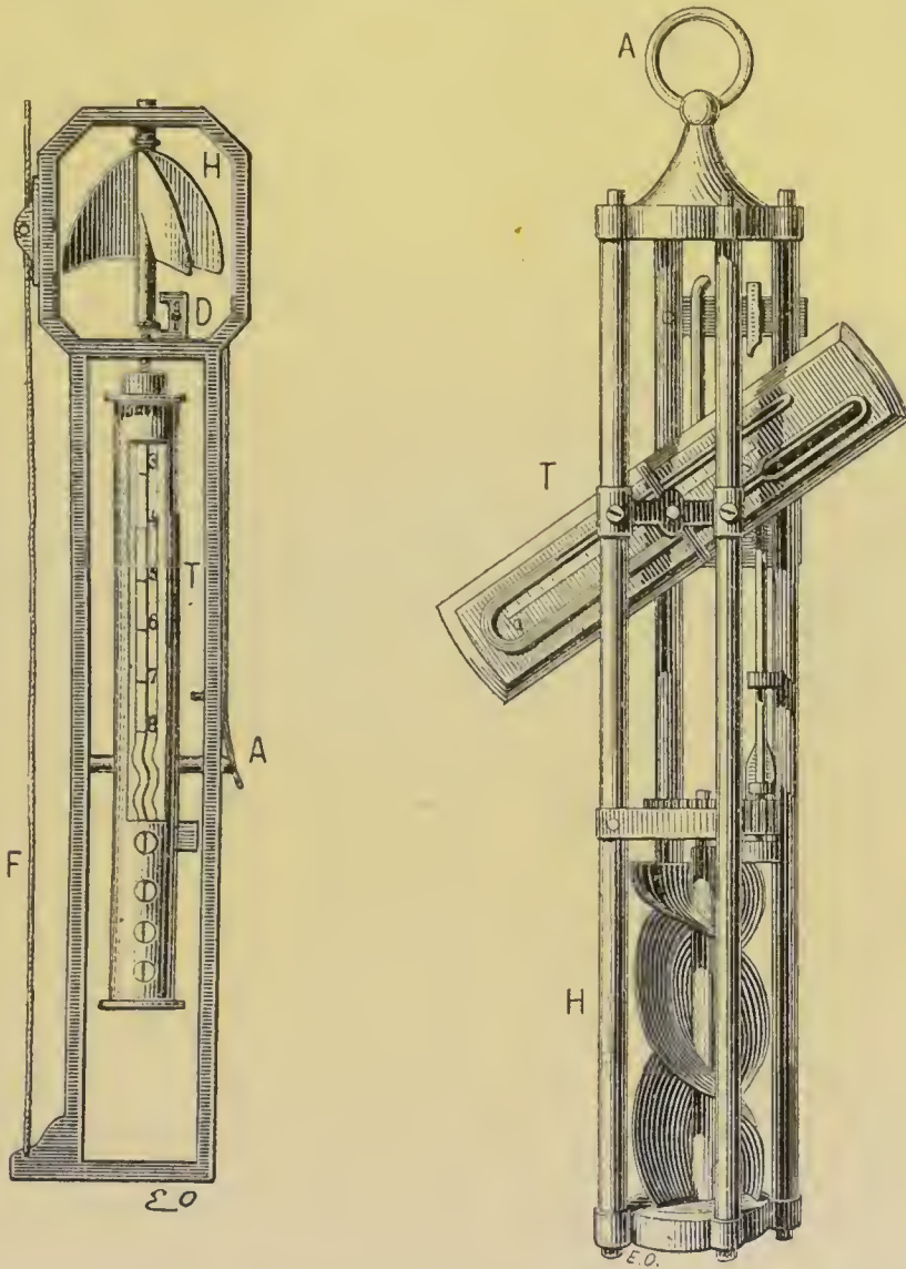
Fig. 138. — Appareil à retournement de l'amiral Magnaghi.
