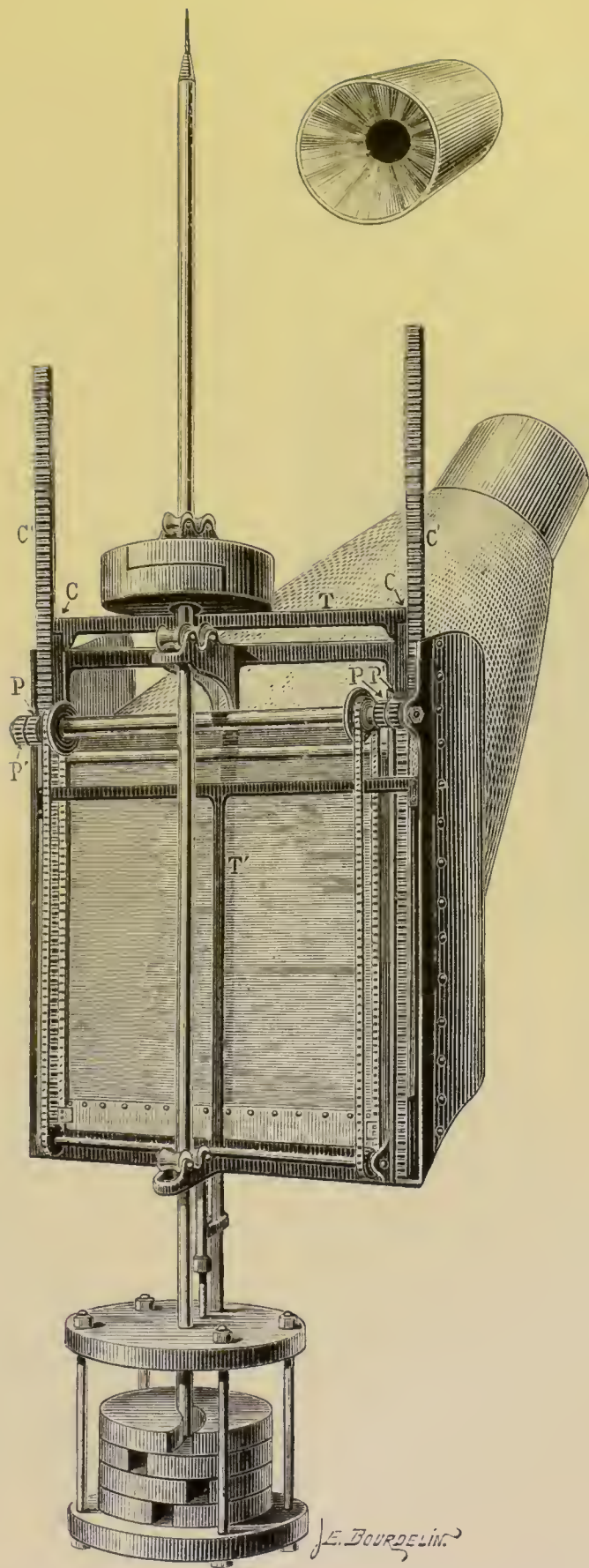
Fig. 13. — Filet pélagique du prince de Monaco représenté au moment où il est fermé et où on le remonte.
