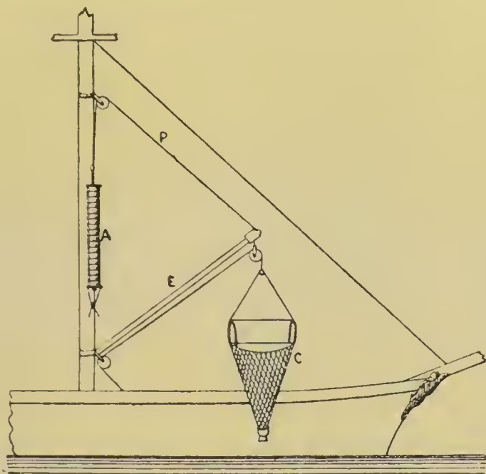
Fig. 8. — Dispositif de la bigue et de l'accumulateur sur le Talisman .
