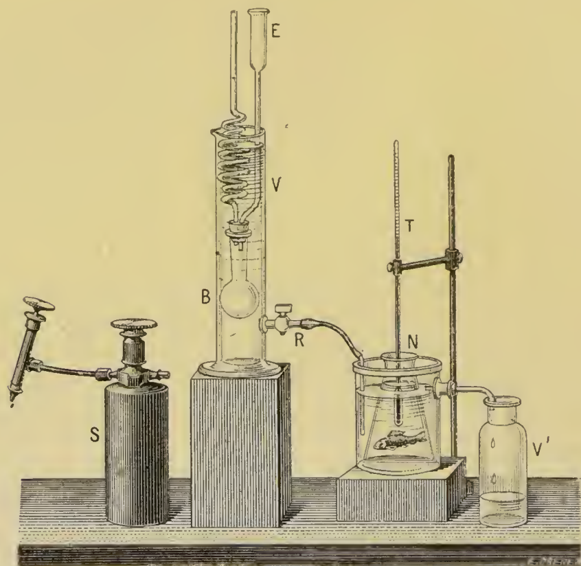
Fig. 156. — Appareil destiné à porter les animaux aquatiques à des températures au-dessous de 0^{\circ} .
