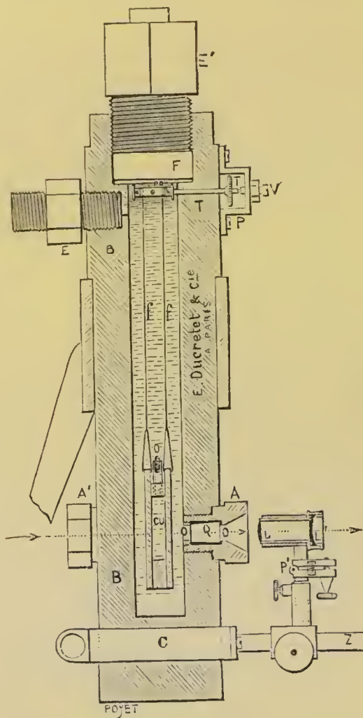
Fig. 89. — Bloc complet de P. Regnard, percé de hublots pour l'étude de l'action des hautes pressions sur la vie.
