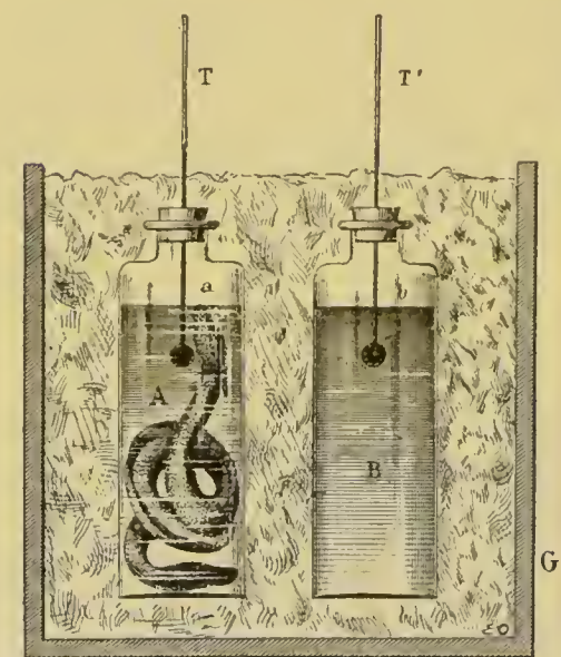
Fig. 153. — Expérience destinée à déterminer approximativement la production de chaleur chez un animal aquatique.
