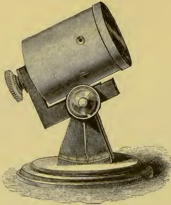
Fig. 99. — Appareil de Jordan pour enregistrer photographiquement les variations de la lumière.
