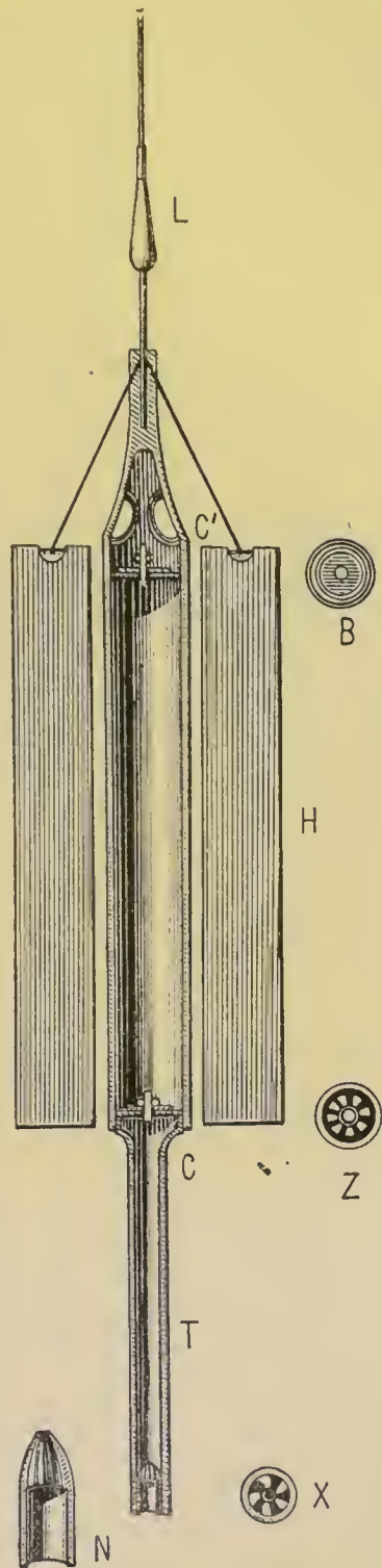
Fig. 166. — Bouteille-sonde du Challenger.
