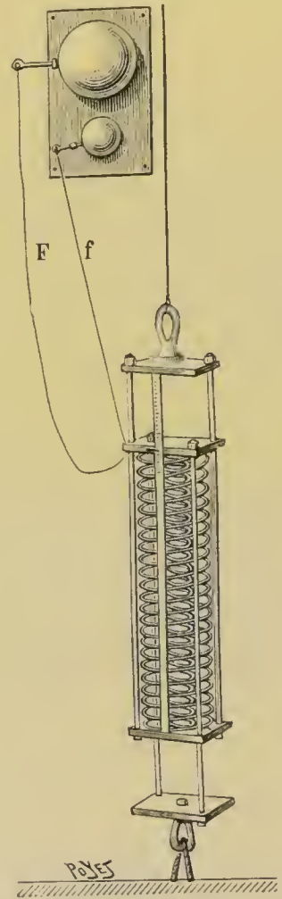
Fig. 10. — Appareil avertisseur des tensions. (Hirondelle.)
