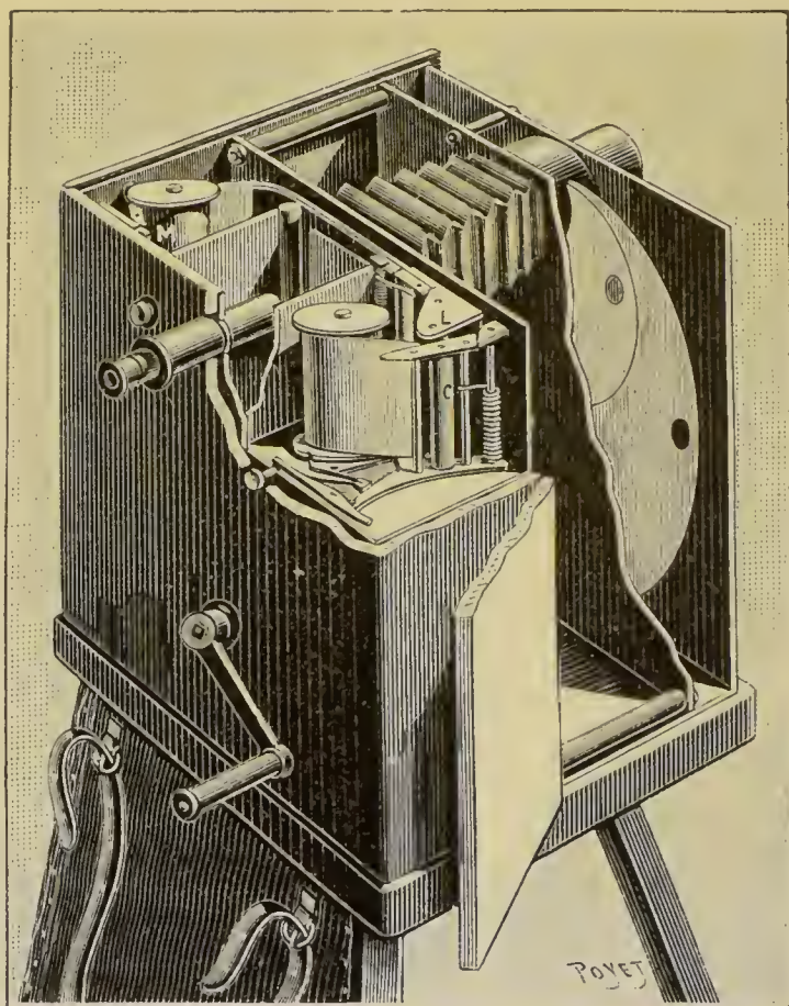
Fig. 227. — Détail de l'appareil Photochronographique de Marey.
