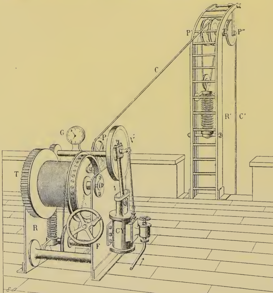
Fig. 66. — Machine à sonder de la Princess-Alice .
