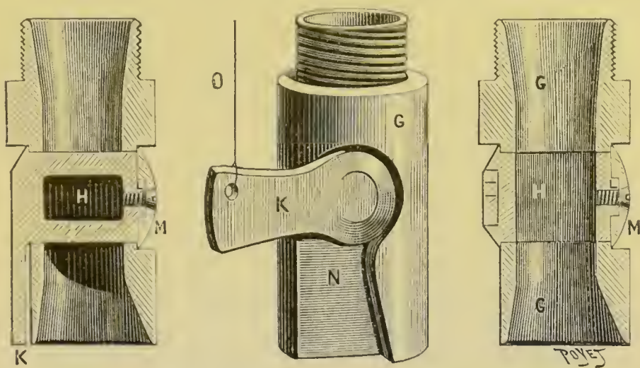
Fig. 61. — Détail du robinet du sondeur à clef.
