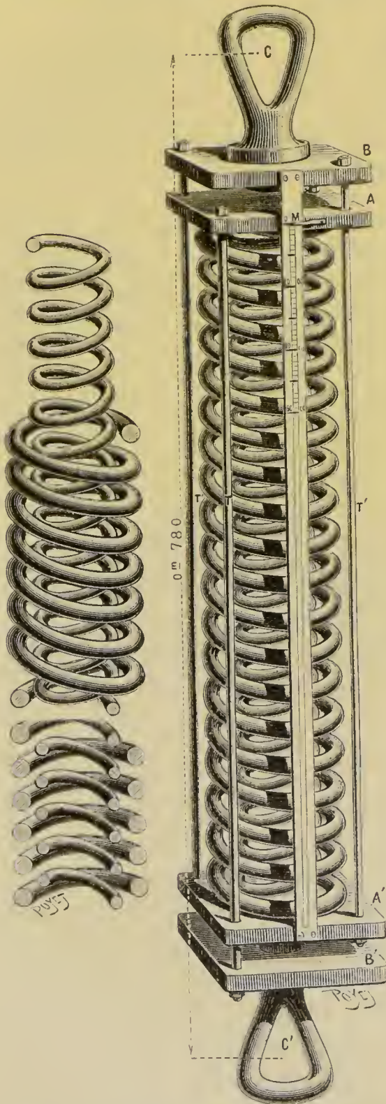
Fig. 9. — Accumulateur de l'Hirondelle.
