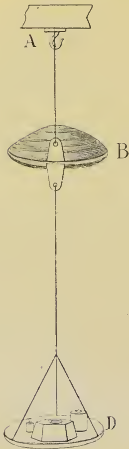
Fig. 220. — Schéma de l'appareil de Plateau destiné à mesurer la force des muscles d'un Mollusque.
