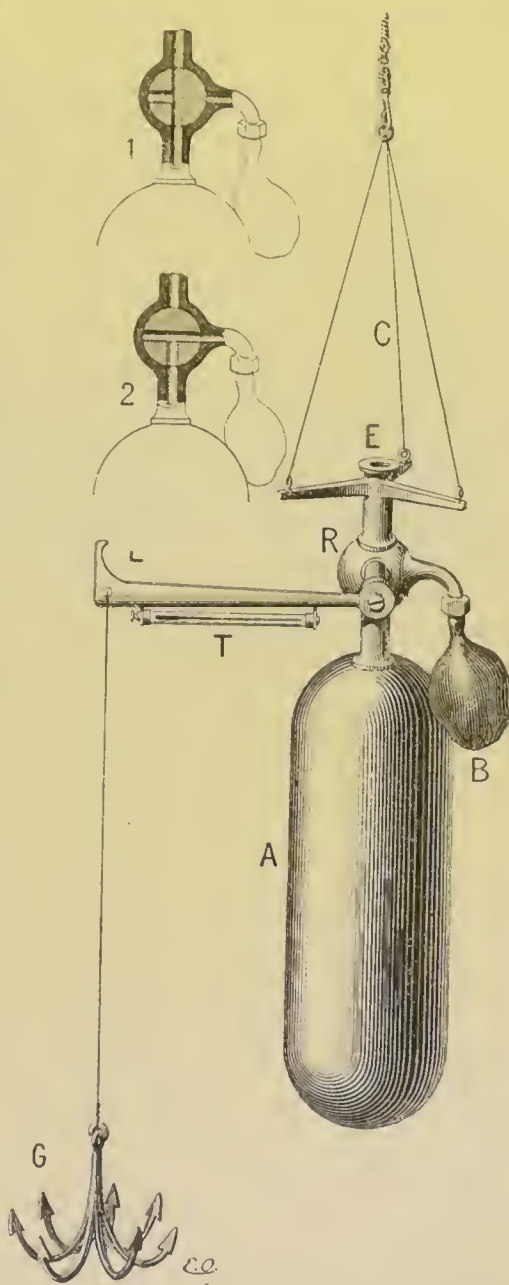
Fig. 69. — Bathomètre de Regnard.
