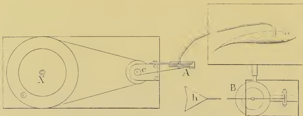
Fig. 218. — Poisson artificiel de Corblin.
