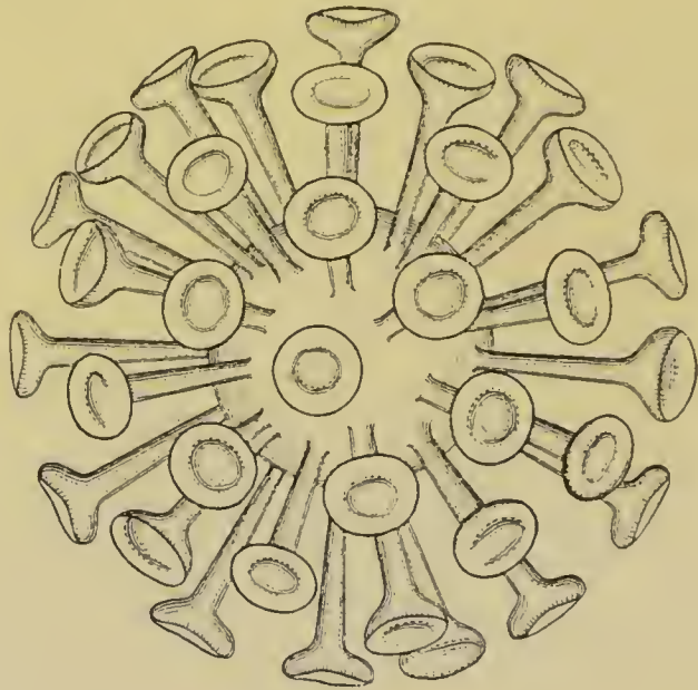
Fig. 36. — Rhabdosphère .
