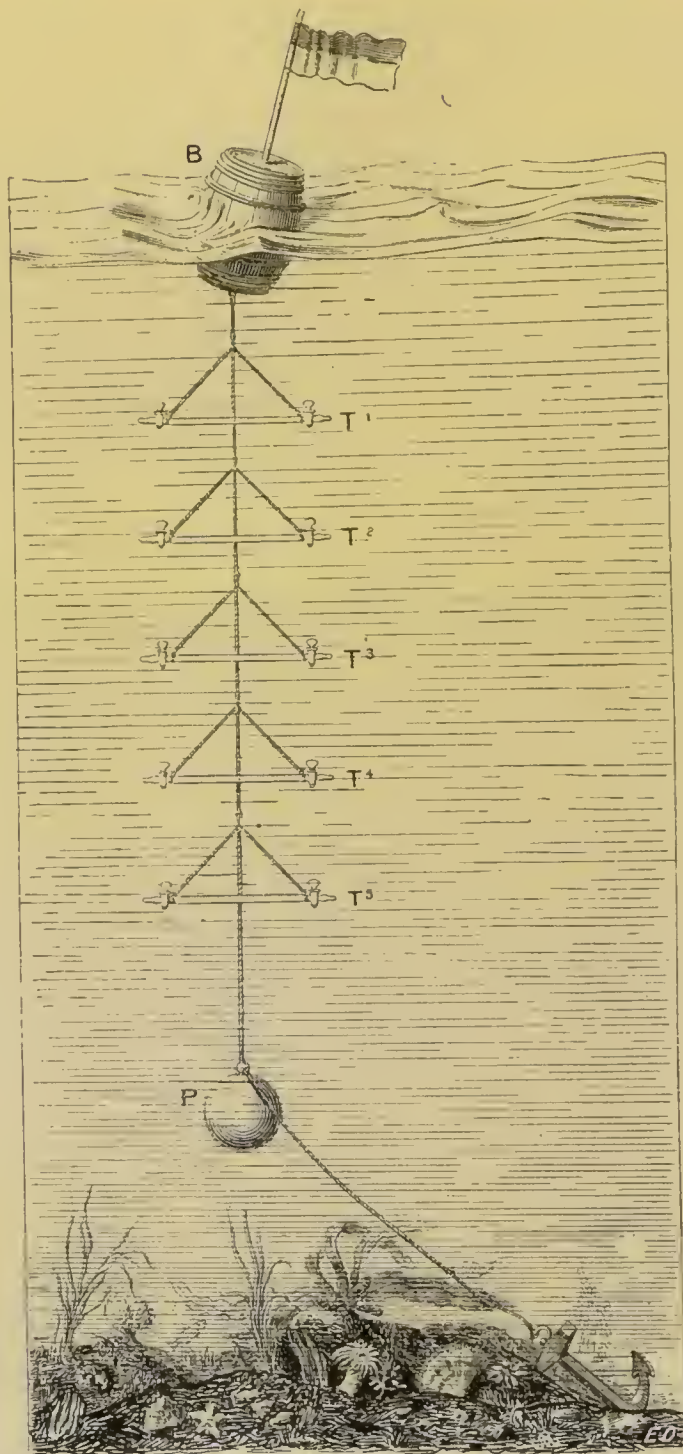
Fig. 113. — Tubes remplis d'un mélange égal d'H et de Cl, suspendus dans la mer.
