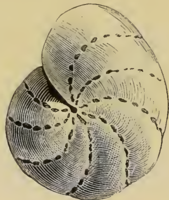
Fig. 29. — Polystomella umbiliculata .
