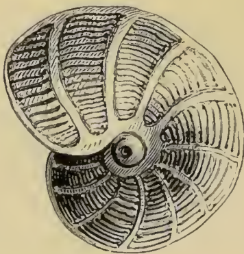
Fig. 28. — Peneroplis planatus .
