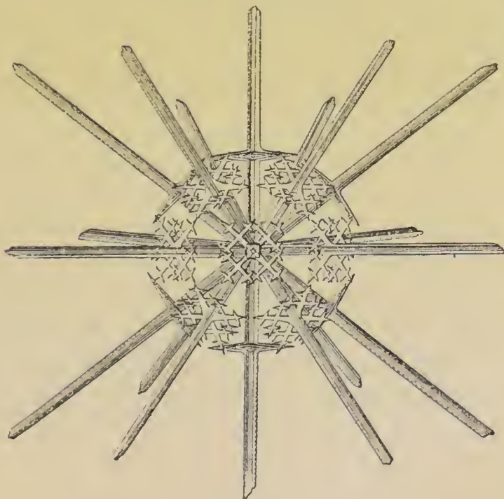
Fig. 33. — Xiphacantha .
