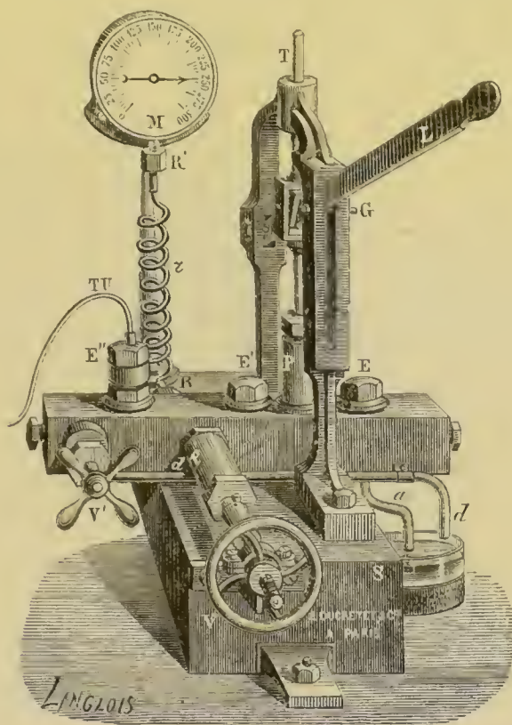
Fig. 74. — Presse hydraulique de Cailletet.
