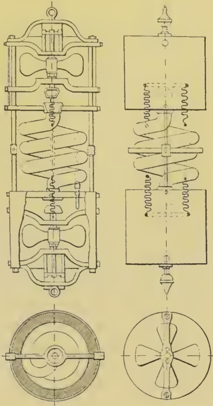
Fig. 169. — Bouteille de Wille.
