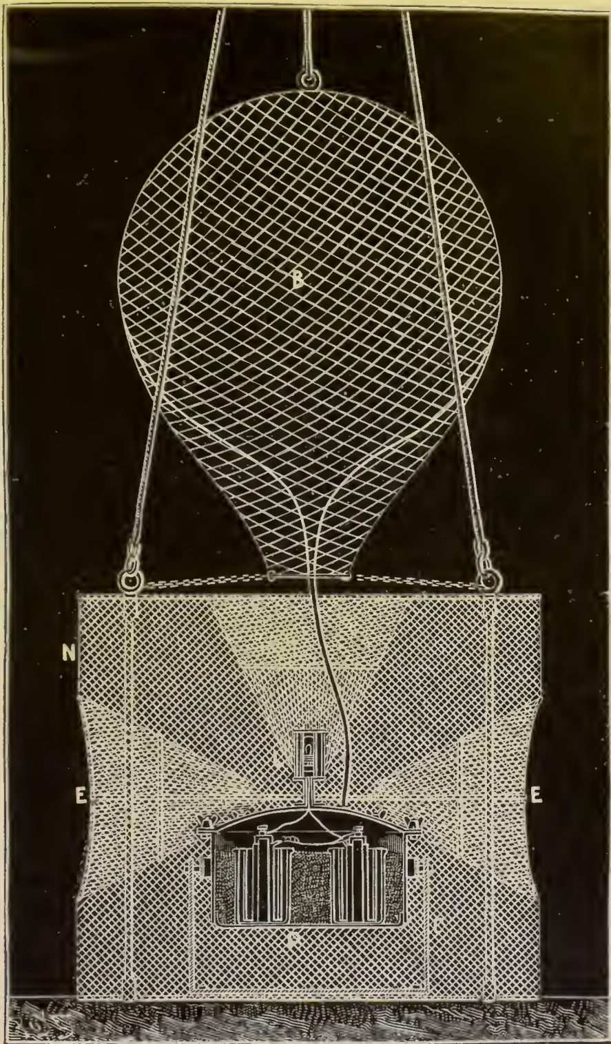
Fig. 17. — Schéma représentant le dispositif qui permet d'envoyer dans la mer une pile en compensant la pression exercée sur ses parois. (Dr P. Regnard).
