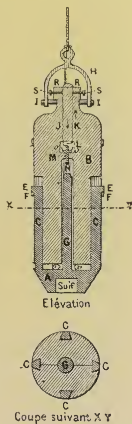
Fig. 58. — Sonde électrique de Delacroix.
