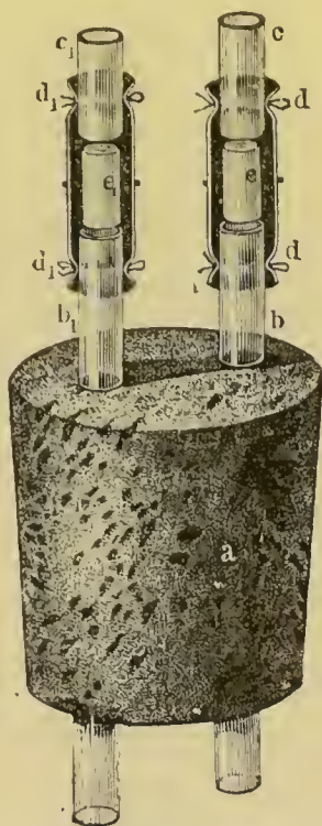
Fig. 159. — Robinet en caoutchouc de Bunsen.
