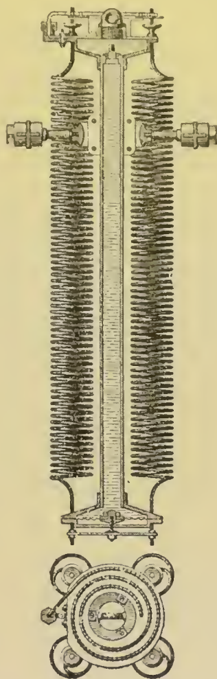
Fig. 70. — Bathomètre de Siemens.
