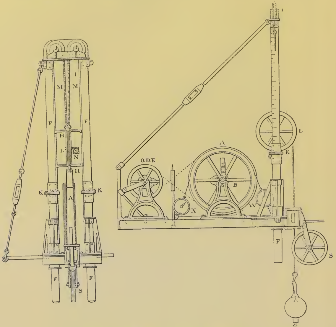
Fig. 64. — Machine à sonder de Sigsbee.
