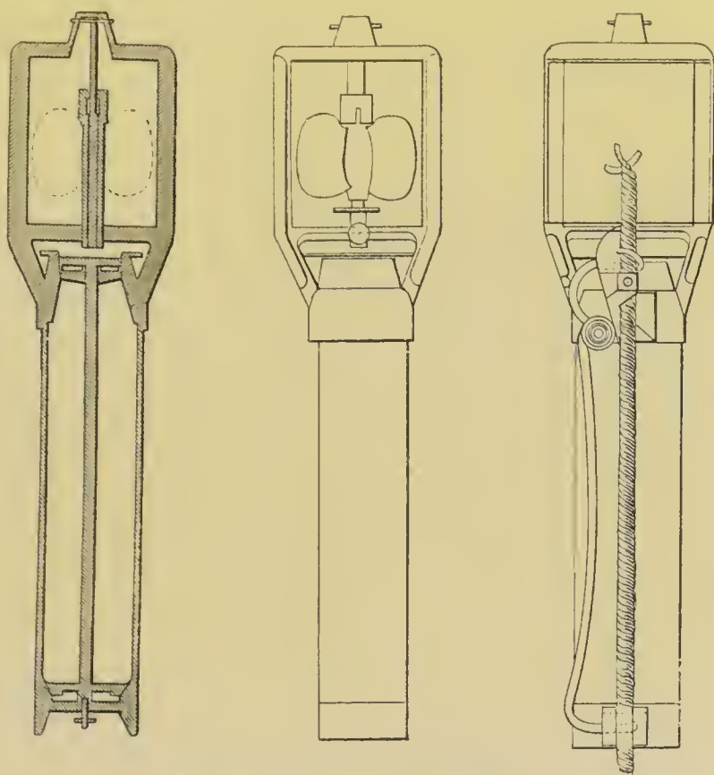
Fig. 168. — Bouteille de Sigsbee.
