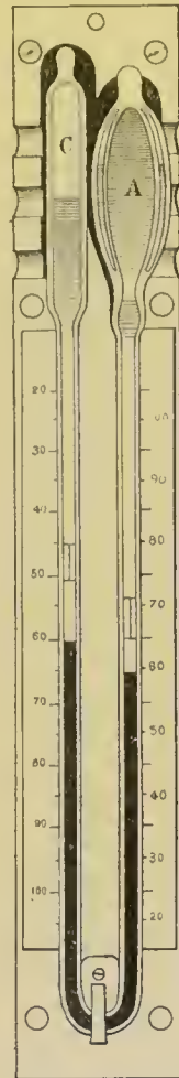
Fig. 133. — Thermomètre Miller-Casella.
