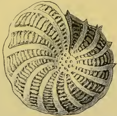
Fig. 27. — Polystomella crispa .
