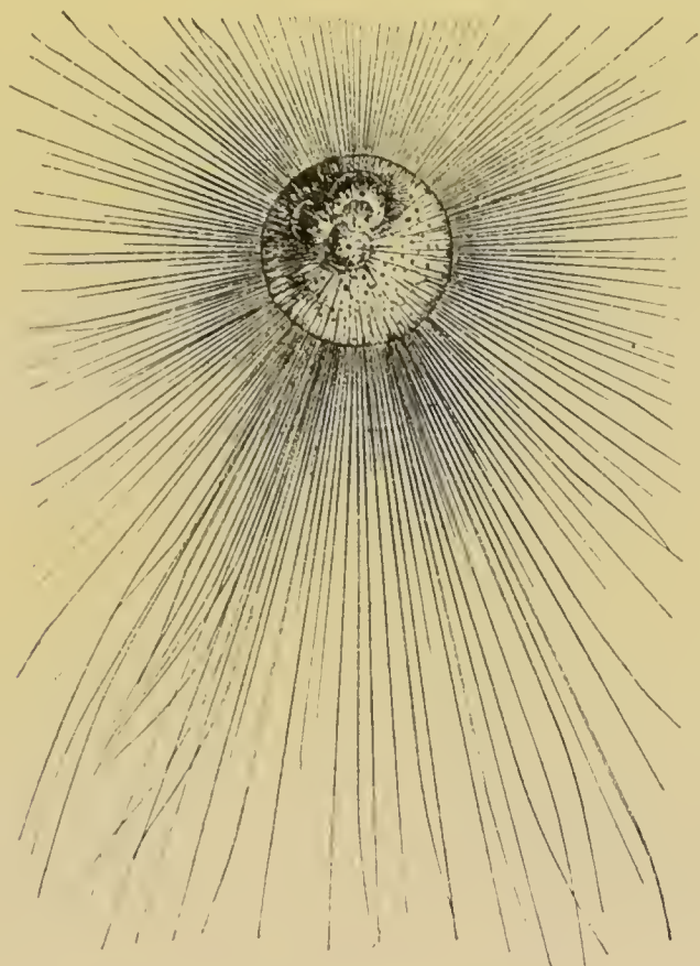
Fig. 20. — Orbulina universa .
