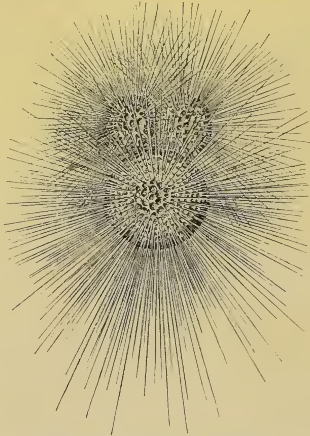
Fig. 21. — Globigerina bulloïdes .
