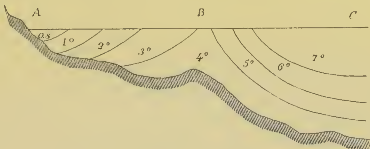
Fig. 146. — Barre thermique des lacs.
