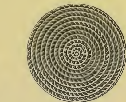
Fig. 23. — Nummulites nummularia .
