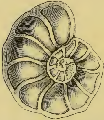
Fig. 26. — Navionina crassula .
