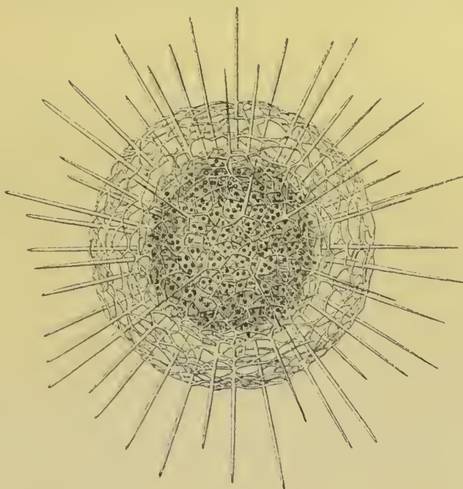
Fig. 32. — Haliomma .
