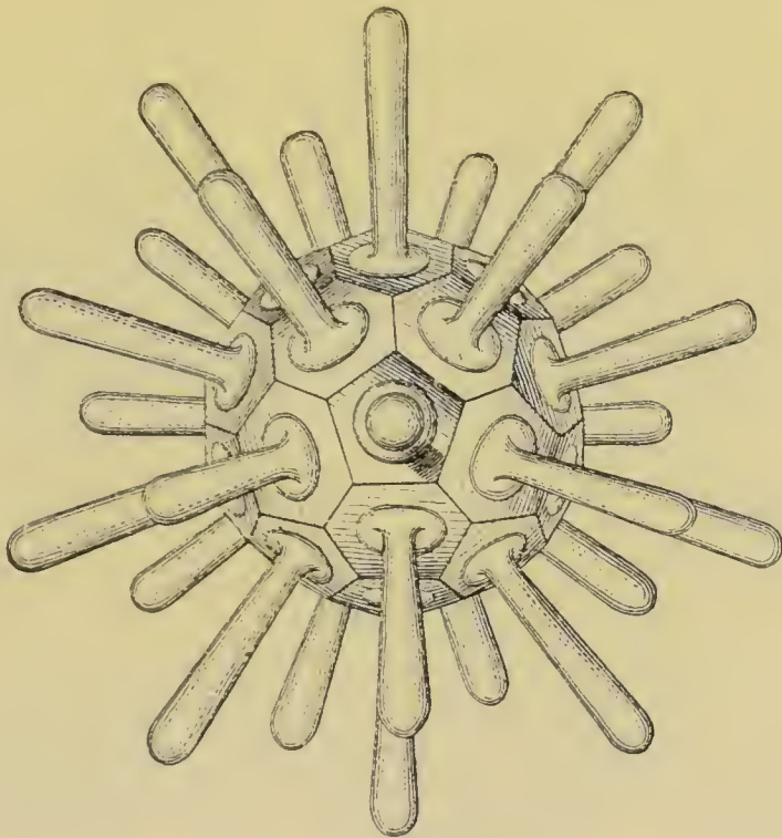
Fig. 37. — Rhabdosphère .
