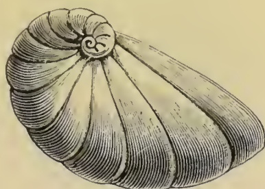
Fig. 25. — Rotalina turgida .
