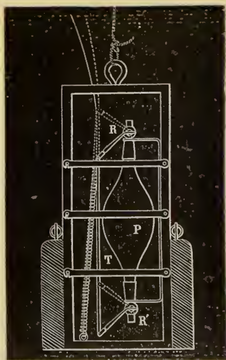
Fig. 162. — Appareil de Jolyet et Regnard pour recueillir l'eau à de faibles profondeurs.
