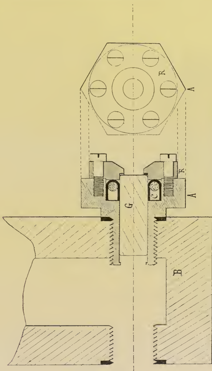
Fig. 88. — Montage des hublots à cuir embouti.
