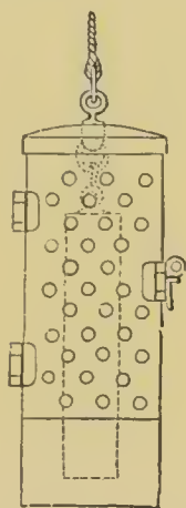
Fig. 131. — Seau à clapet pour prendre la température de la surface de la mer.
