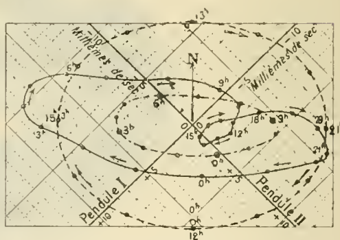
Fig. 5. — Fortes déclinaisons australes (de - 17° à - 19° S; moyenne - 16° 20').
