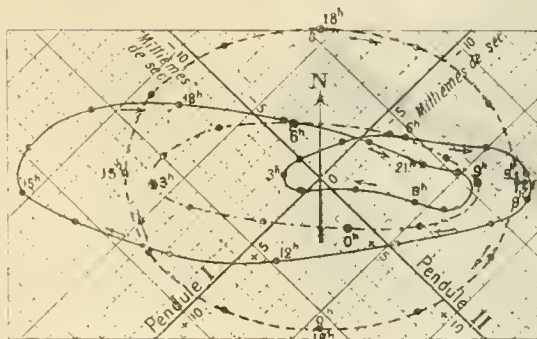
Fig. 4. — Fortes déclinaisons boréales (de + 13° à + 19° N; moyenne + 16° 15').
