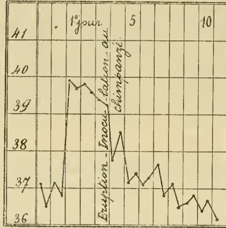
Courbe M.B.K.D. Typhus exanthématique. Courbe 1.
