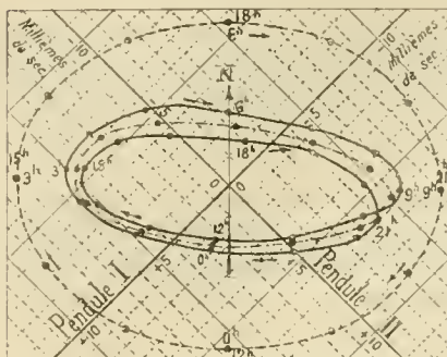
Fig. 2. — Décembre 1902 à mai 1905.
