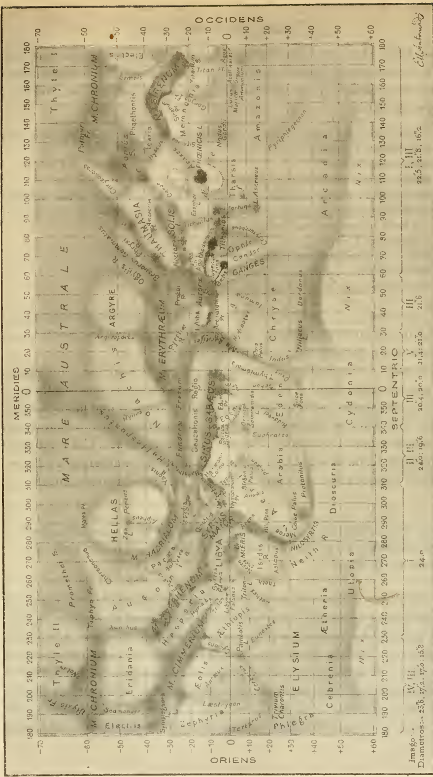
Carte de la planète Mars, dressée sur la projection de Mercator, d'après les observations faites, à l'Observatoire de Meudon, du 20 septembre au 9 novembre 1909. Abréviations : M , Mare; L , Lacus; Fl , Fluvius; R , Regio; I , Insula; Ch , Chersonesus; Pr , Promontorium.
