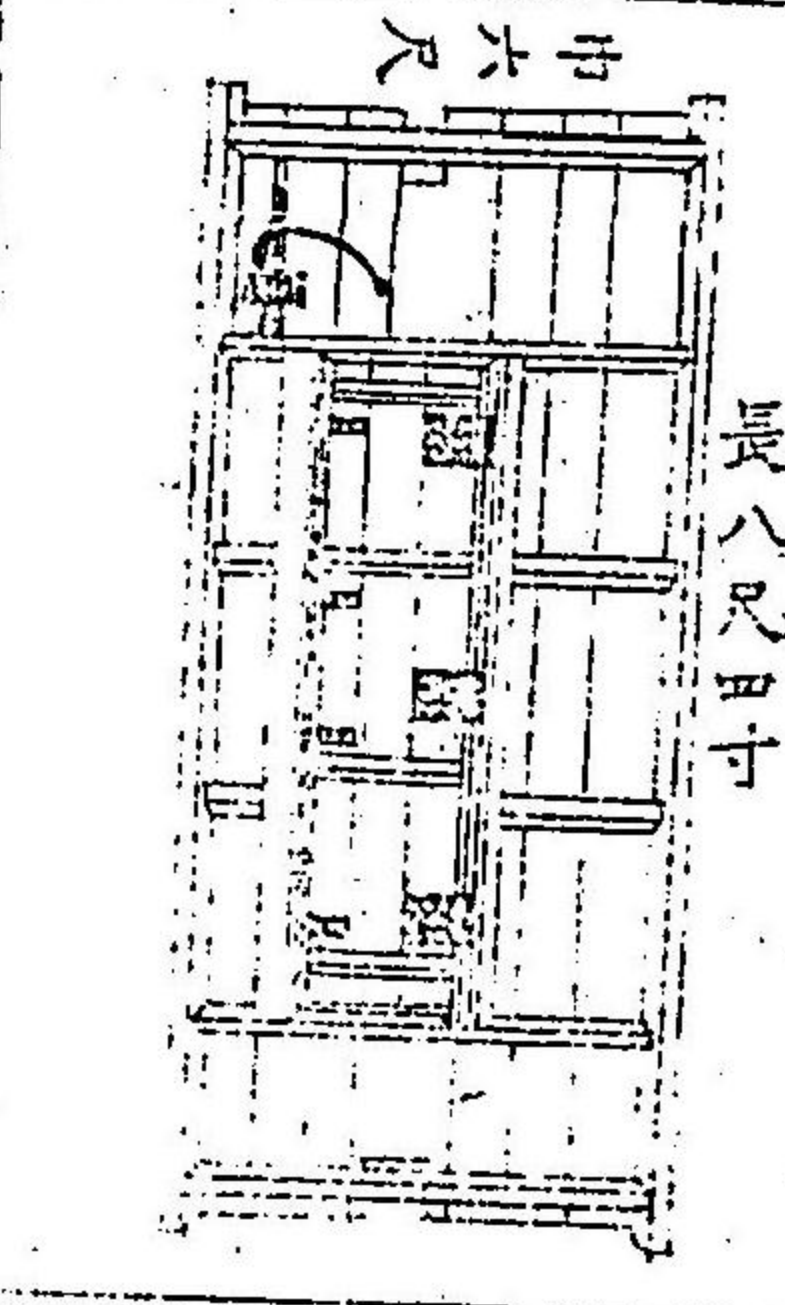
踏板裏面圖
