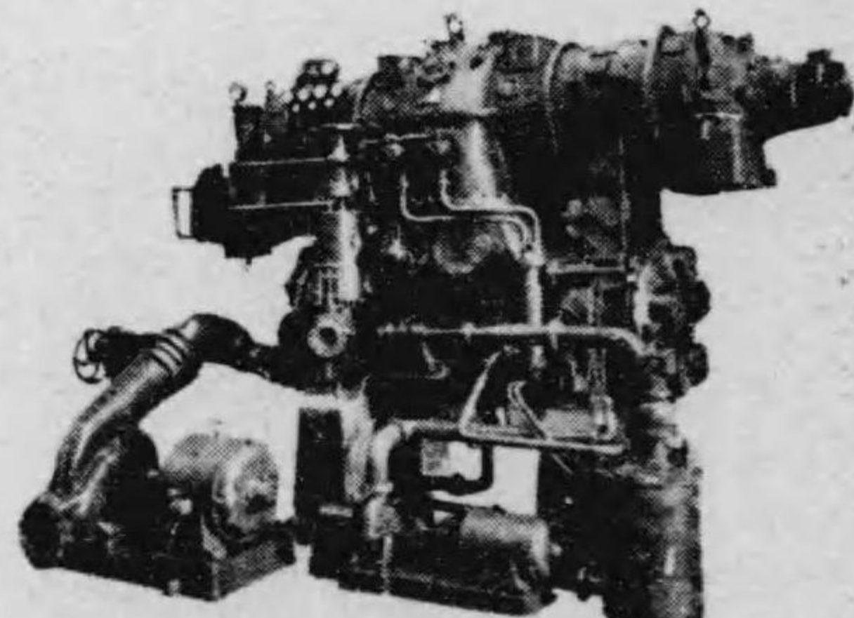
神戶造船所製造 1,500 K. W エンゲストロームターボ發電機
