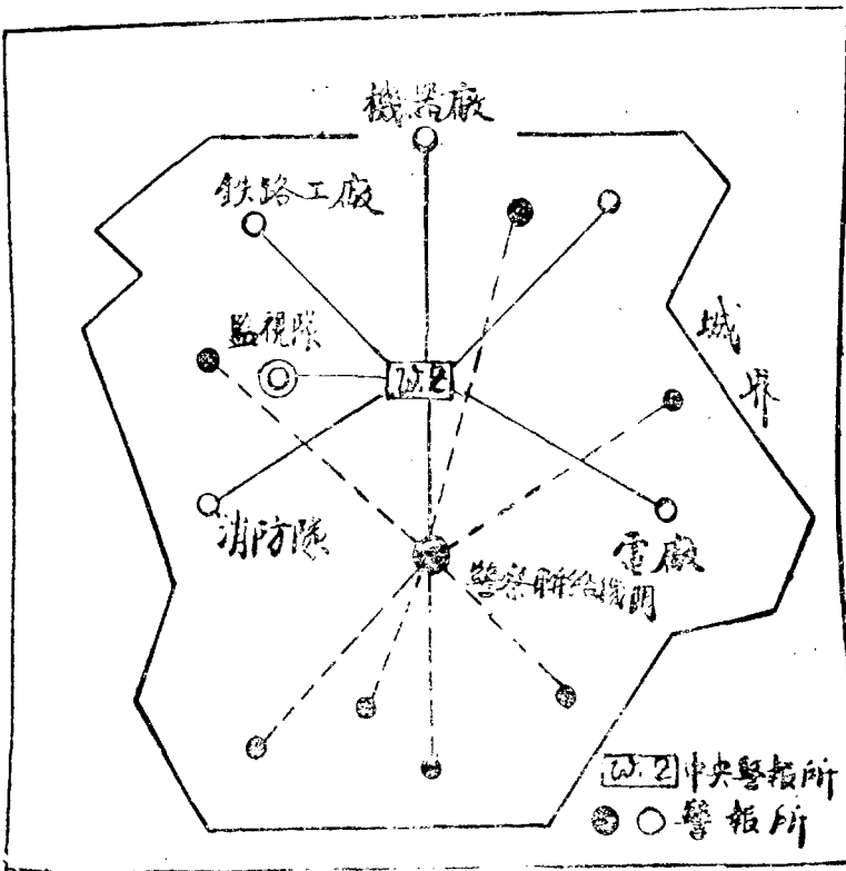
第十七圖 城市各處與中央警報所的聯絡
