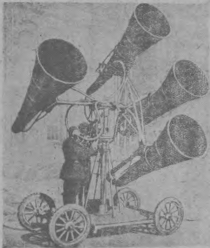
圖 一 十 第 機 音 聽 空 院 國 美 第
