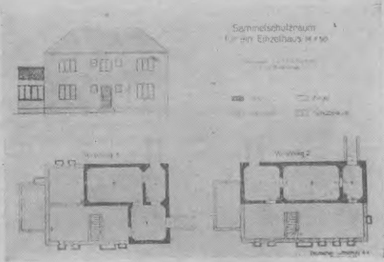
第二十圖 德國防空協會的設計
