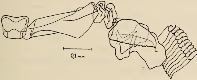
FIG. 3. Radula de Neritina tiassalensis .
