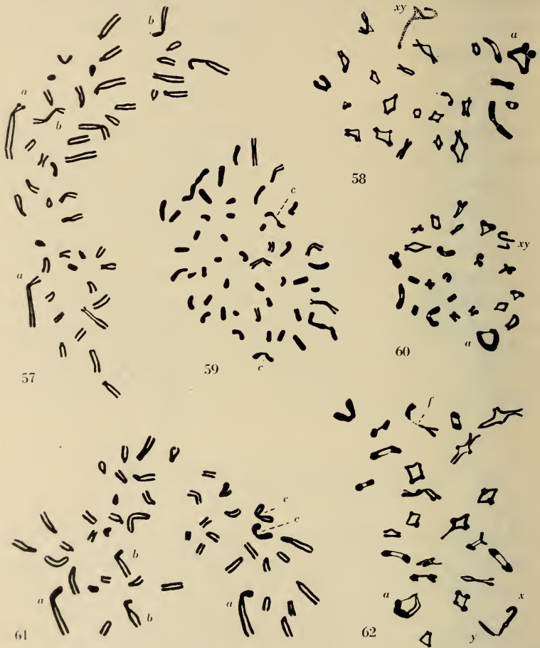
FIG. 57-62. — Pitmys multiplex et Pitmys fatioi .
