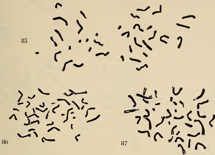
FIG. 85-87. — Arvicola terrestris persicus . Fig. 85-87: métaphases spermatogoniales. — \times 1.800 .
