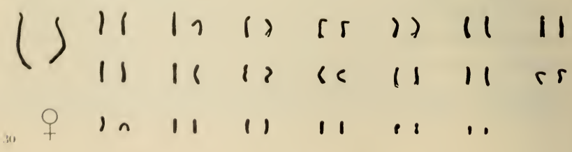
FIG. 25-30. Sériation des chromosomes chez le ♂ et la ♀ de Gerbillus gerbillus .
