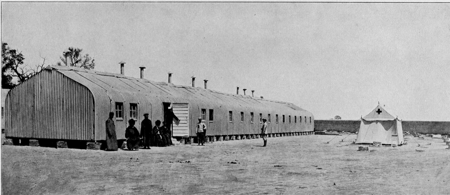
Складной цинковый барак для раненыхъ Георгіевской общины Краснаго Креста. Наружный видъ.
