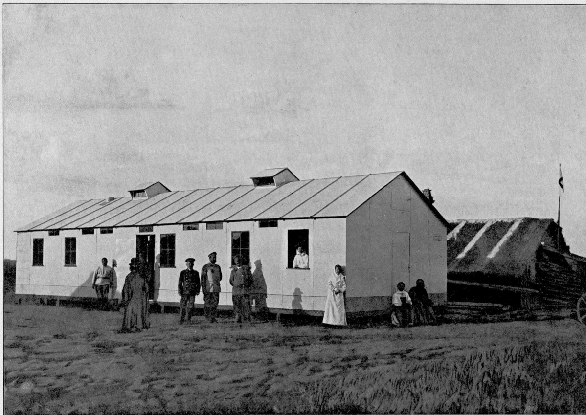
Складной картонный баракъ.
