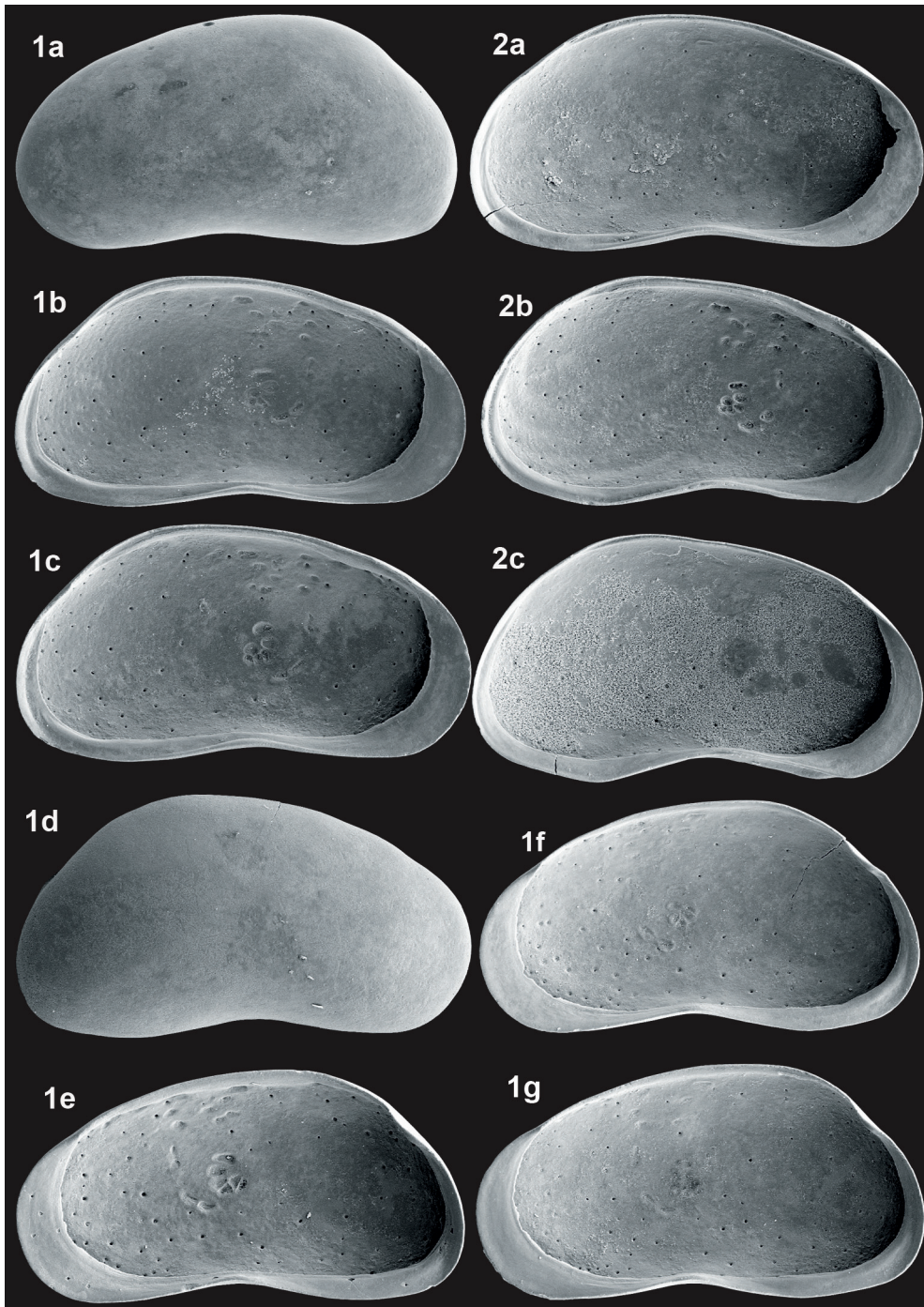
Fabaeformiscandona tricatricosa (DIEBEL & PIETRZENIUK, 1969) – Zauschwitz (59) mWKz Weibchen: 1a - LVa (L 1,19), 1b - LVi (L 1,16), 1c - LVi (L 1,19), 1d - RVa (L 1,14), 1e - RVi (L 1,20), 1f - RVi (L 1,16), 1g - RVi (L 1,15), Männchen: 2a - LVi (L 1,20), 2b - LVi (L 1,16), 2c - LVi (L 1,16).
