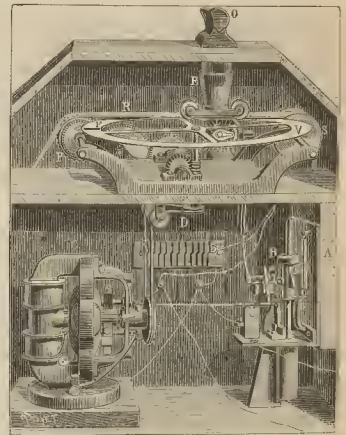
Fig. 3. - Mecanismo motor del kinetoscopio
