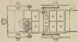
Fig. 3. Plano del coche eléctrico. BB Acumuladores M. Máquina. - C. Conmutador
