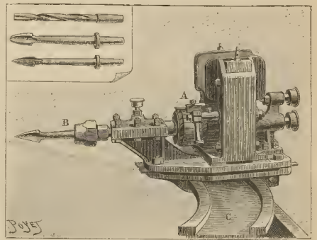
Fig. 2. Vista exterior de la perforadora eléctrica y de las piezas que sirven para labrar la madera
