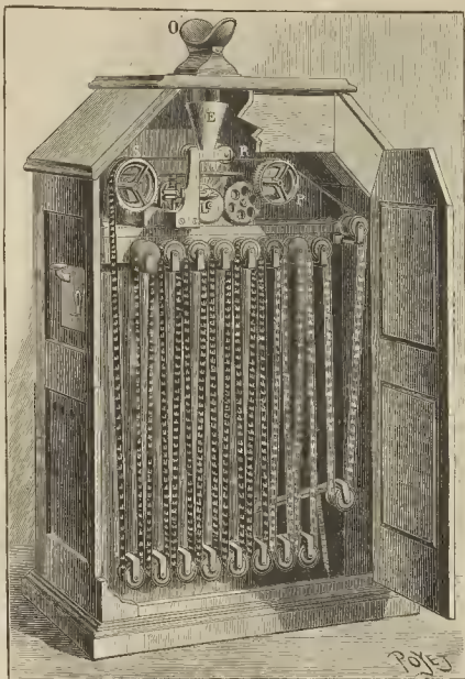
Fig. 4. - Modo de arrollar en el cinematógrafo la cinta de celuloide en la cual se han sacado las pruebas cronofotográficas.
