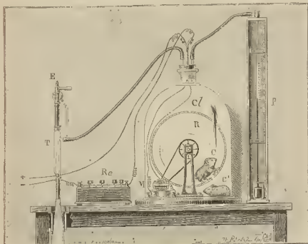
Aparato del doctor Regnard para el estudio del mal de montaña. - Cl. Campana en la que se puede hacer el vacío. - CC'. Conejos de Indias. - R. Rueda puesta en rotación por un motor eléctrico M. - Re. Caja de resistencia para regular la presión. - TE. Bomba de agua. - P. Manómetro.
