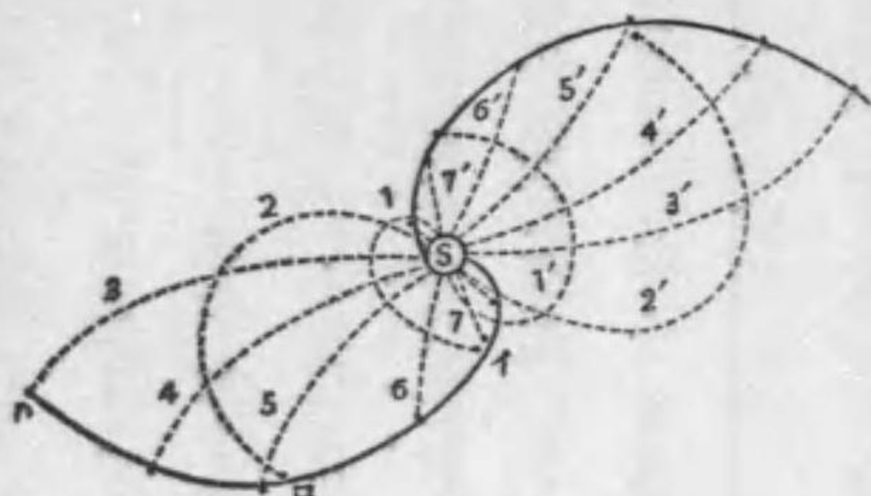
渦狀流
