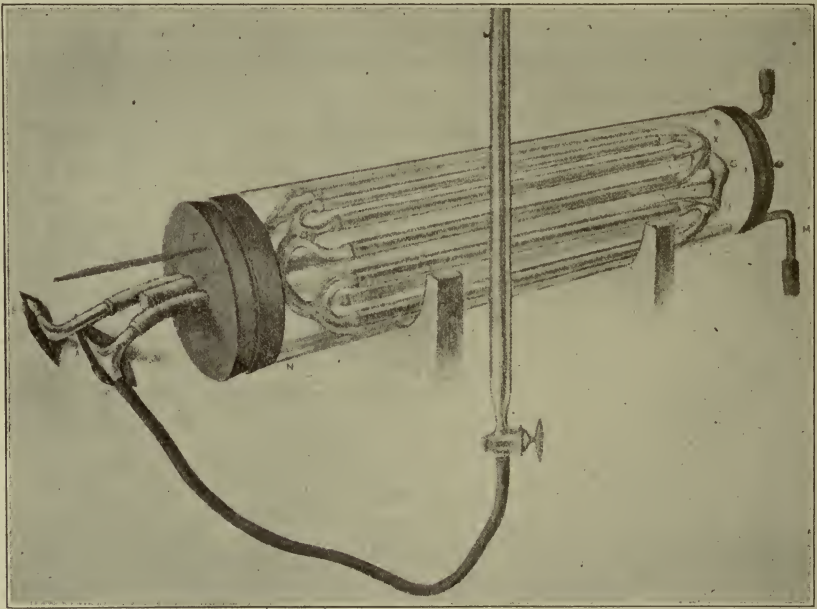
Fig. 187.—Vividiffusion apparatus of J. J. Abel.
