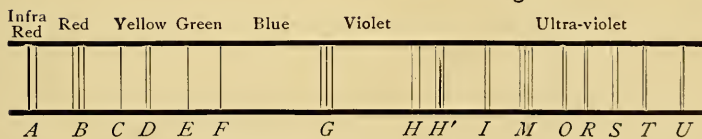
Fig. 9. 2 —Solar Spectrum.
