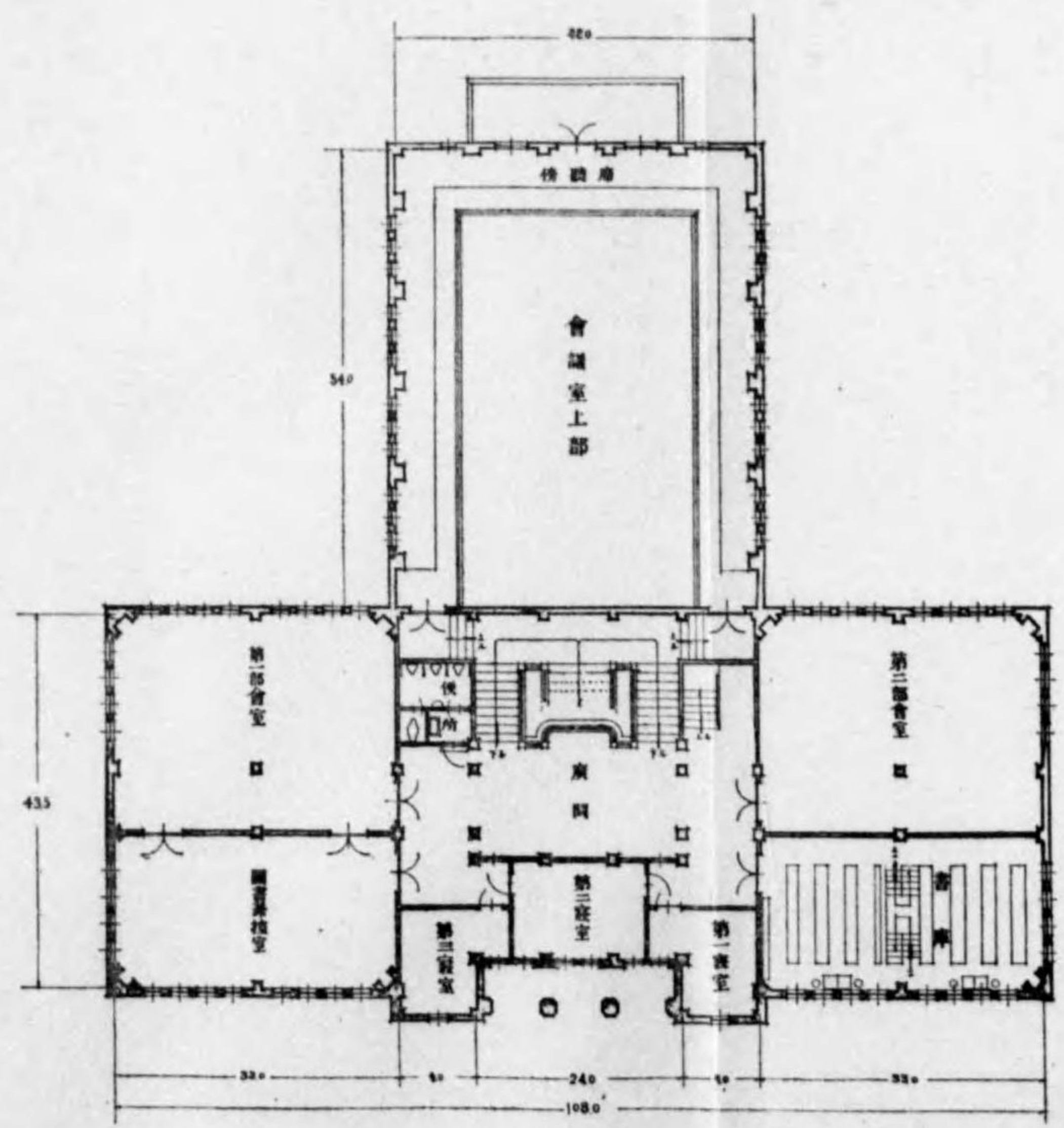
三階平面圖
