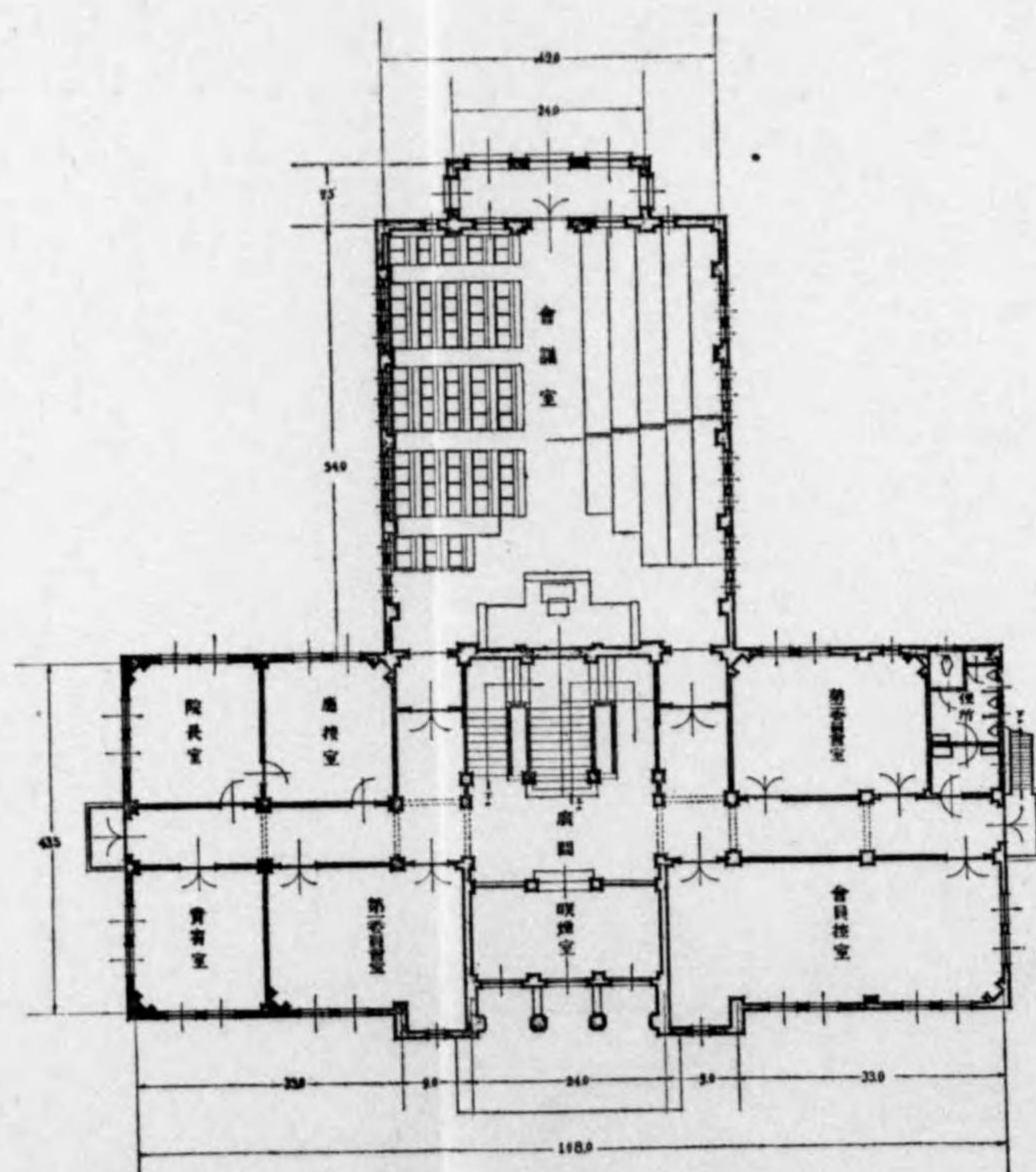
二階平面圖
