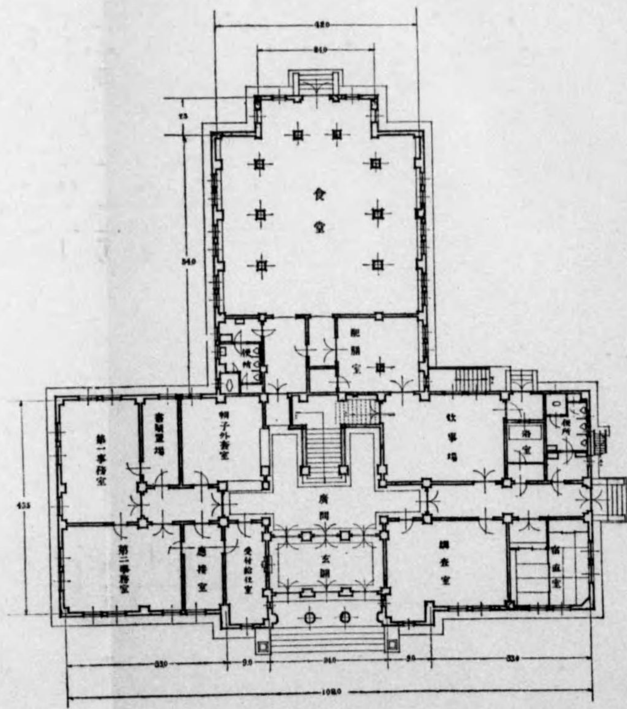
一階平面圖
