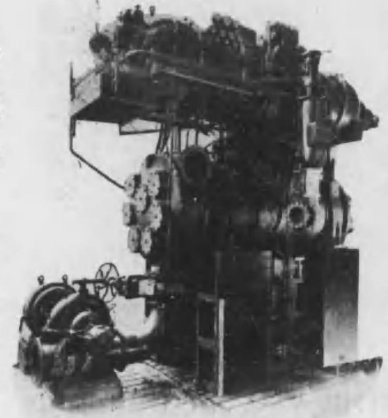
神戸造船所製作 5,000 K.W. ユングストロームターボ發電機
