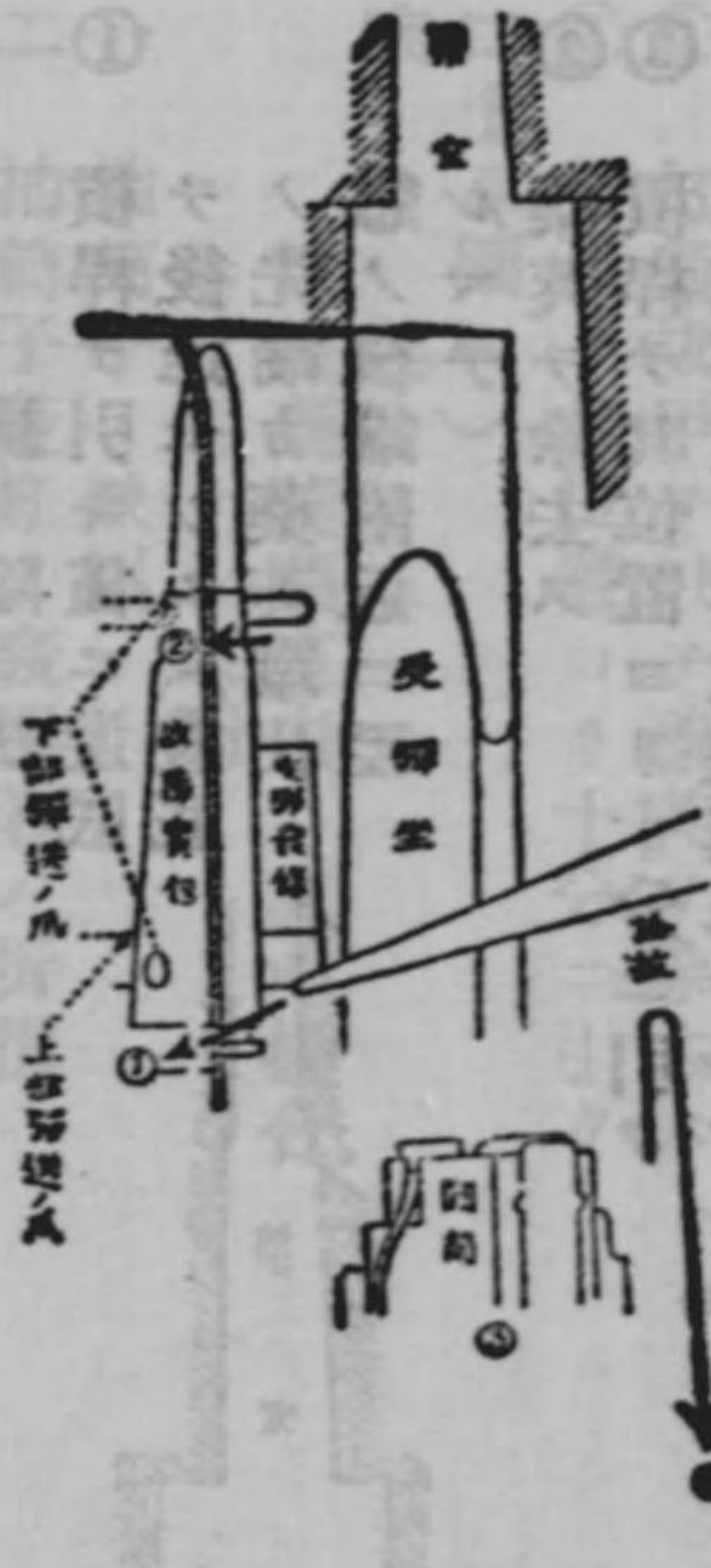
藥英蹴出ヨリ見ル圓筒通路附板
