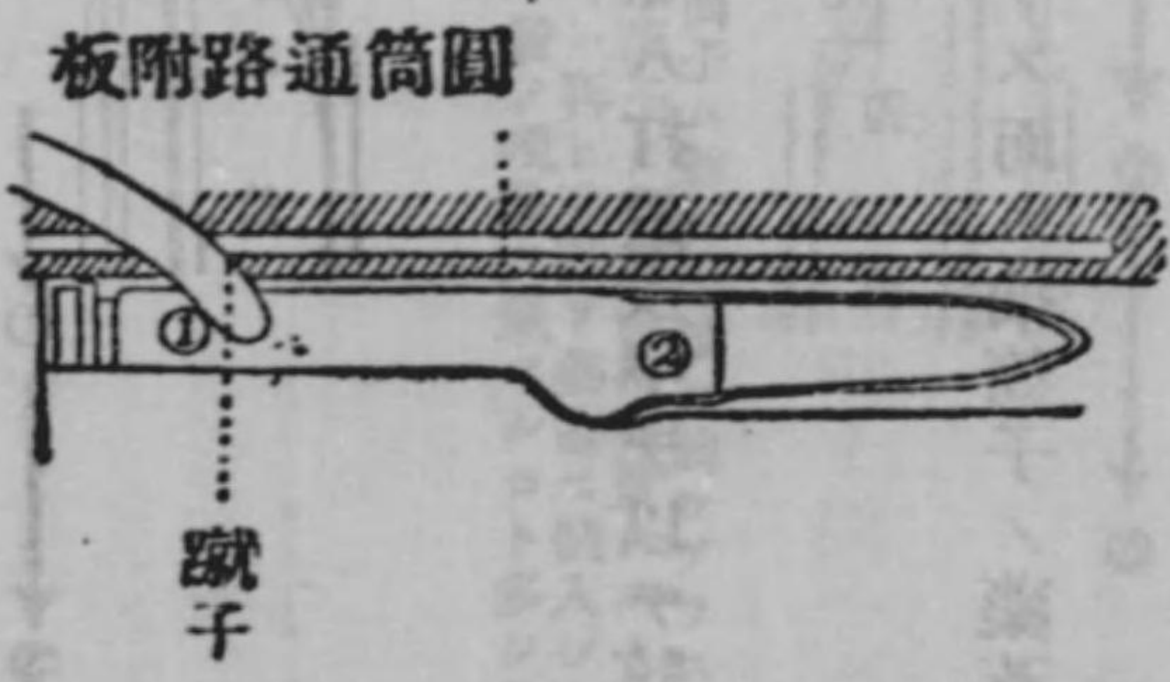
藥英蹴出ヨリ見ル圓筒通路附板
