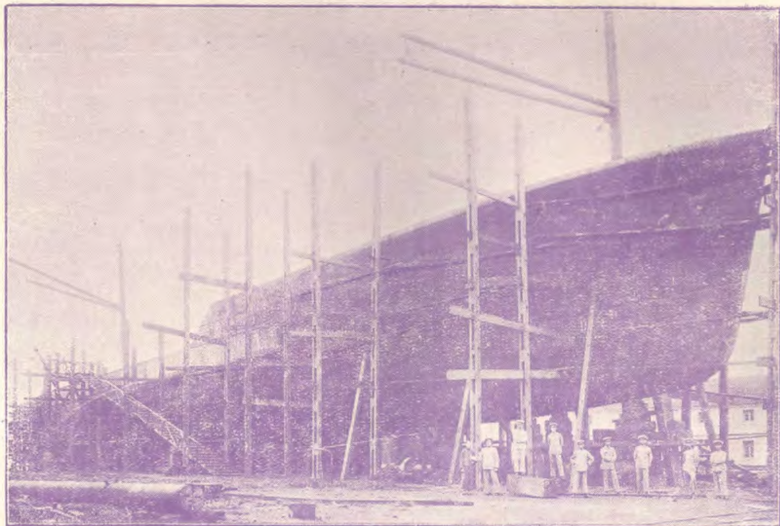
建 造 中 之 逸 仙 軍 艦 之 側 面
