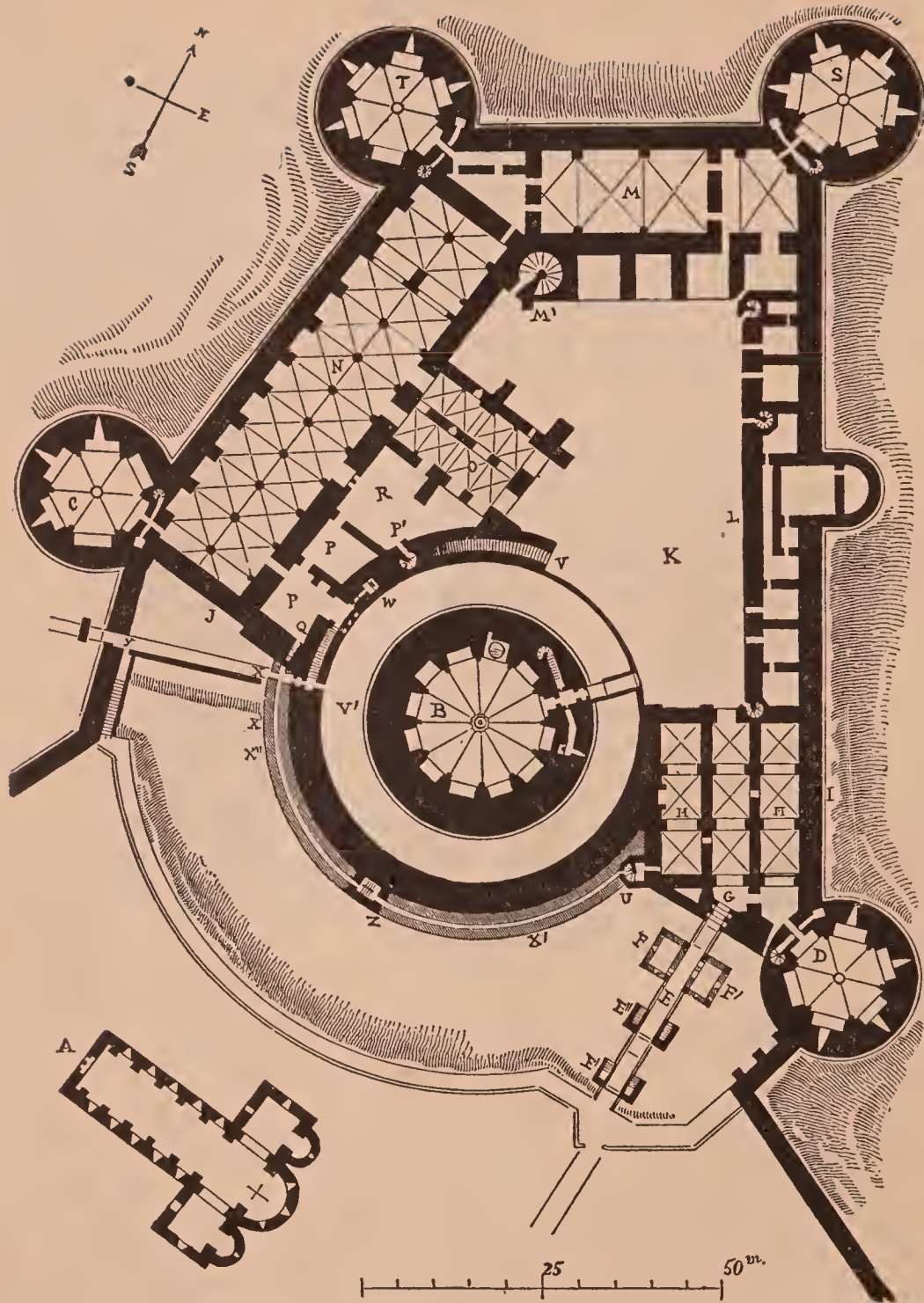
CHÂTEAU DE COUCY (Ground Plan)
