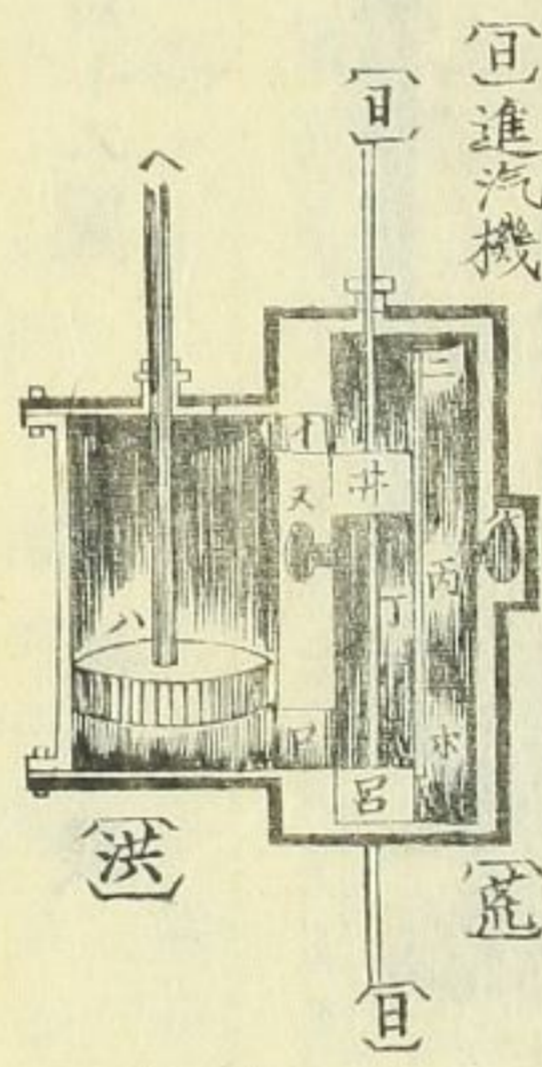
進汽機降リシ時ノ内景
