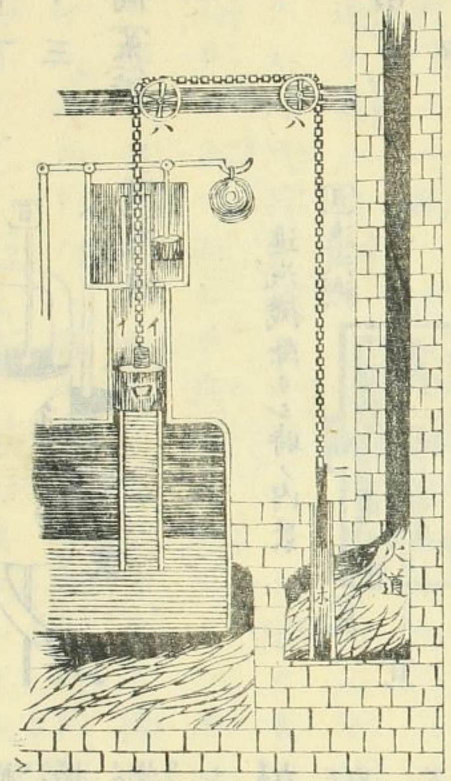
第百十二圖 直鎮火機
