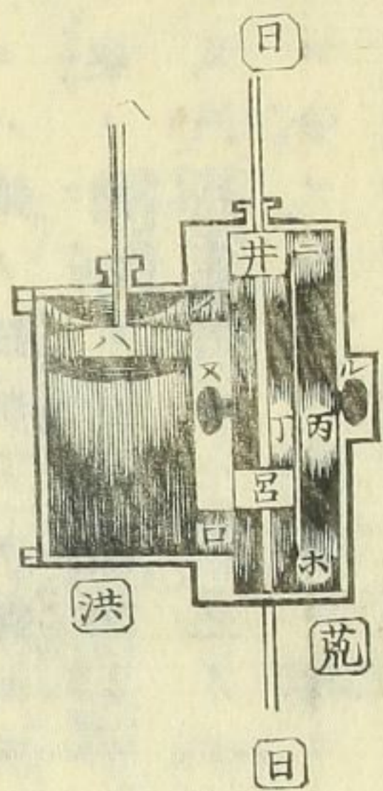
進汽機昇リシ時ノ内景
