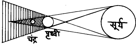
आकृती २ : चंद्रगिराण
