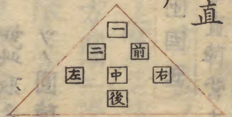
如此モ銳陣ナリ
