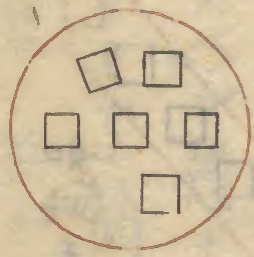
如此ナルモ圓陣營ノ筭ナリ
