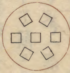
如此取タルモ圓陣ナリ
