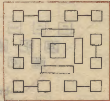
如此取タルモ方陣營ナリ
