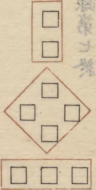
此ハ方陣ト直陣ノ筭ニテスムナリ
