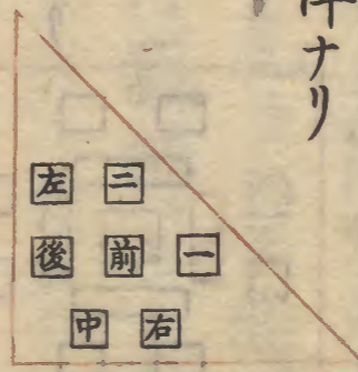
如此モ銳陣ナリ
