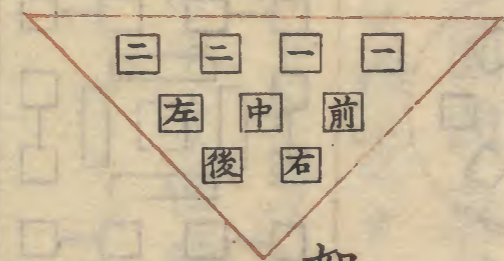
如此モ銳陣ナリ
