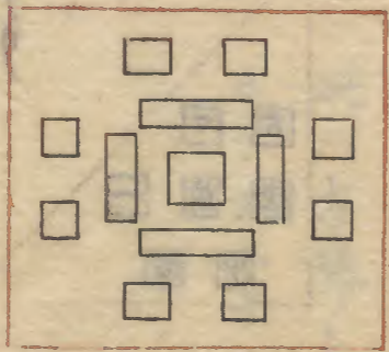
如此取タルモ方陣營ナリ 筭ニテ角欠タル ユヘ方陣營ナリ 人數ノ多少ニヨリ テ替レリ
