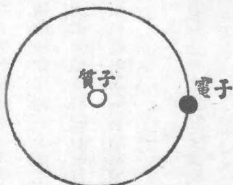
圖 1. 氫原子
