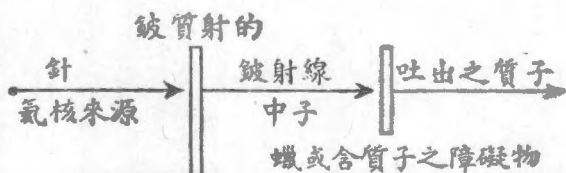
圖 2. 中子之產生
