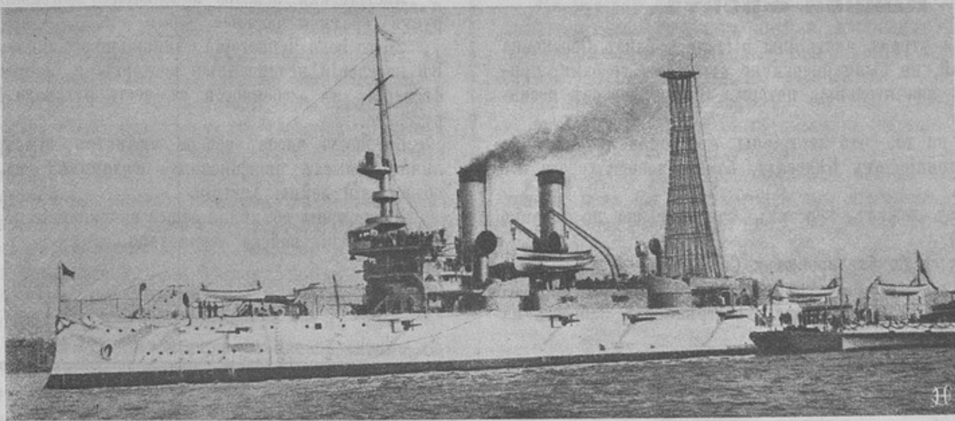
Броненосецъ „Идахо“, купленный у Америки Греціей.
