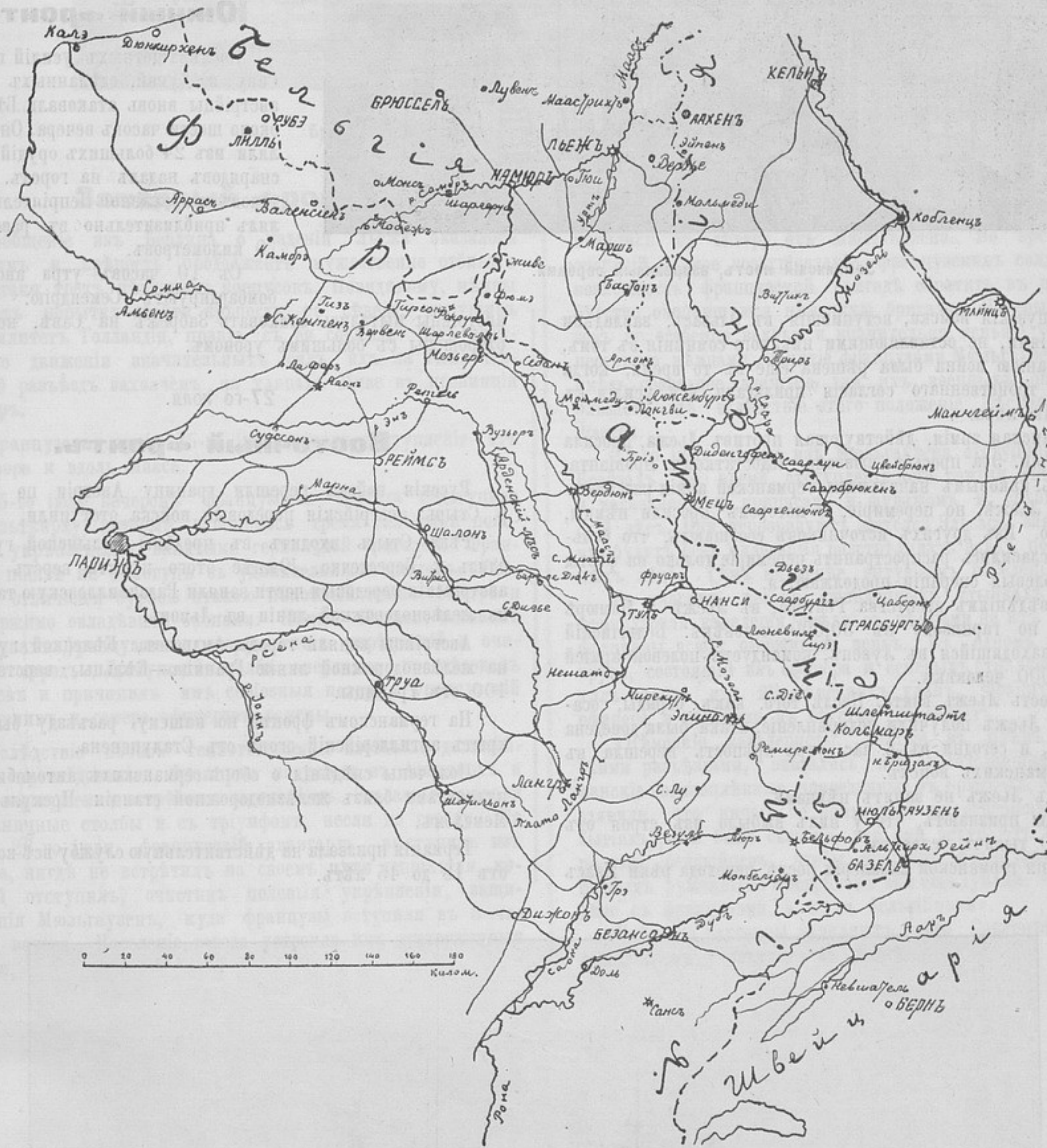
Пограничное пространство Франціи, Бельгіи и Германіи.
