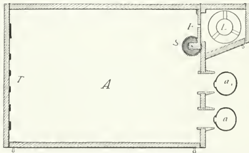
FIG. 100.—Photometer of Förster (Fuchs).
