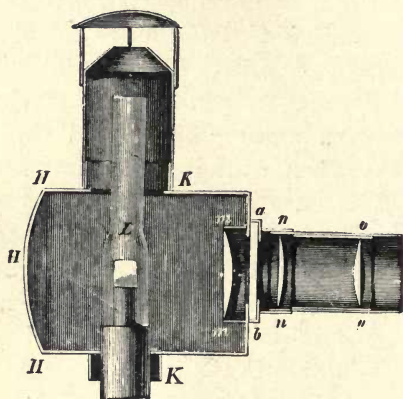
Magic Lantern.
