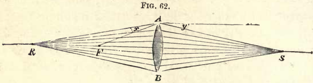
Conjugate foci.
