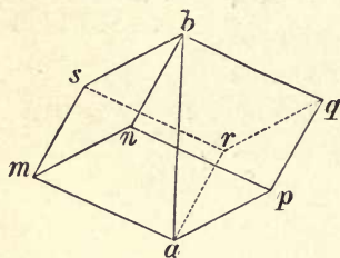
Rhombohedron.
