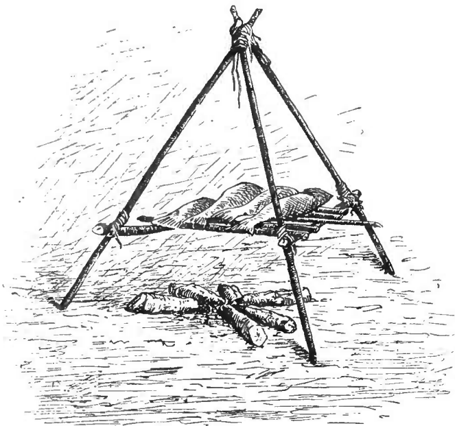
Abb. 30. Bratständer (Trempe). ( \frac{1}{30} nat. Gr.)
