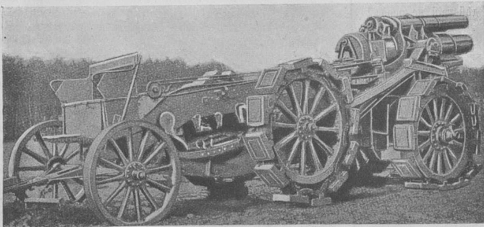
21-сантиметровая нѣмецкая позиціонная гаубица.
