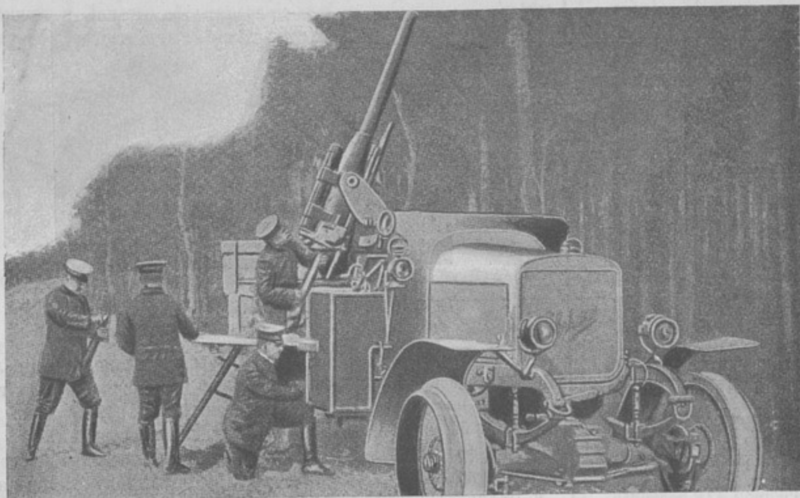
Блиндированный автомобиль съ пушкой для обстрѣливанія воздушныхъ аппаратовъ.
