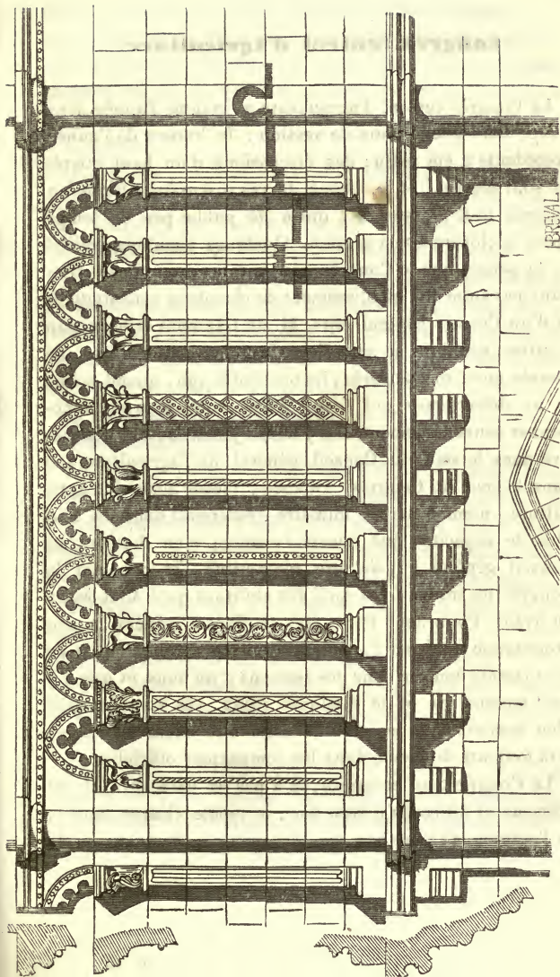
ARCATURES A L'EGLISE DE LA CHARITE-SUR-LOIRE.
