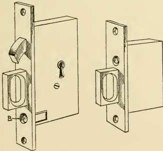
Fig. 386 — Sliding Door Lock.
