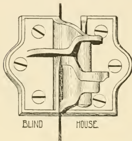
Fig. 444—Ideal Blind Hinge.
