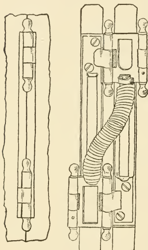
Fig. 351—Chicago Spring Butt.
