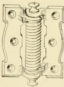
Fig. 413.—Columbia Spring Hinge.
