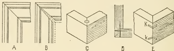
Fig. 201.—Mitre Joints.
