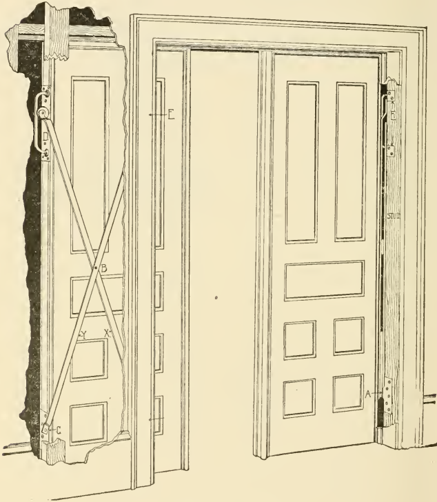
Fig. 362.—Prescott Door Hanger.
