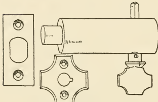
Fig. 403 Gem Bolt.
