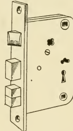
Fig. 384.—Communicating Door Lock.
