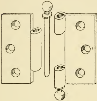
Fig. 342.—Loose-Pin Butt.
