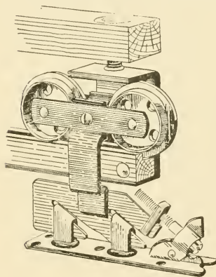
Le Roy Hanger. Fig. 355.
