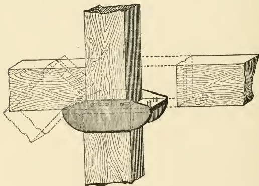
Fig. 465.—Duvinage Cap.
