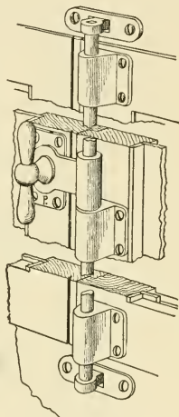
Fig. 434.—Double Rim Espagnolette Bar.
