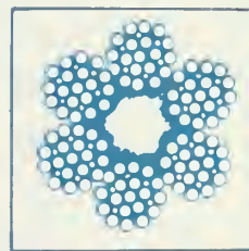
6x25 FILLER WIRE
